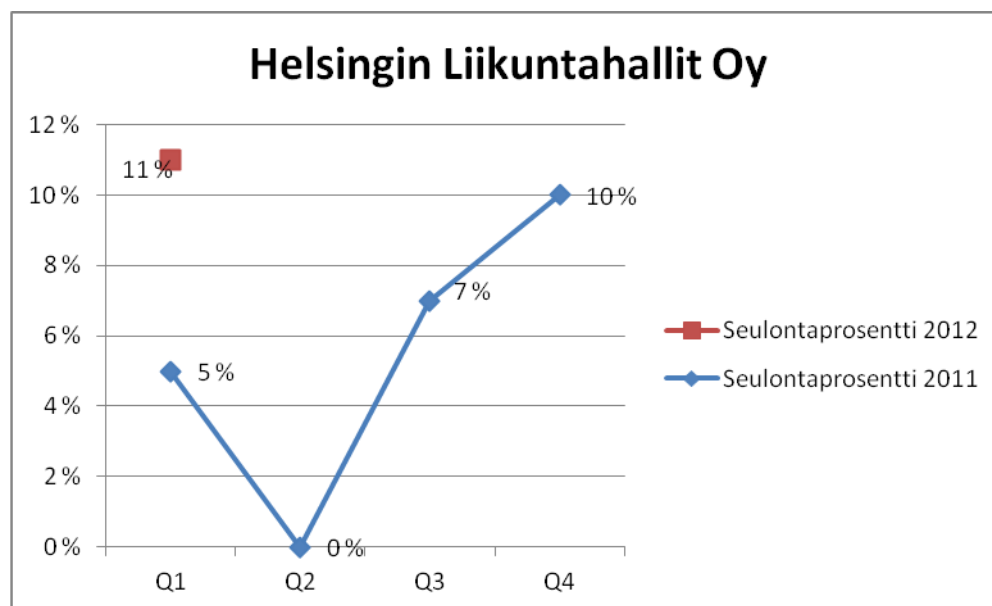
Kuva 124. Seulontaprosentin kehitys.
