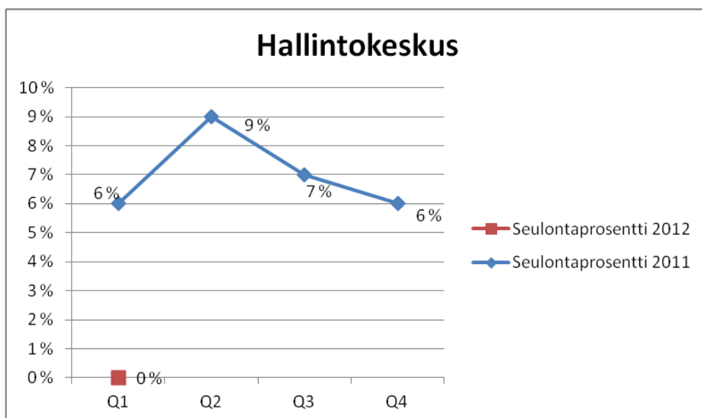
Kuva 30. Seulontaprosentin kehitys.
