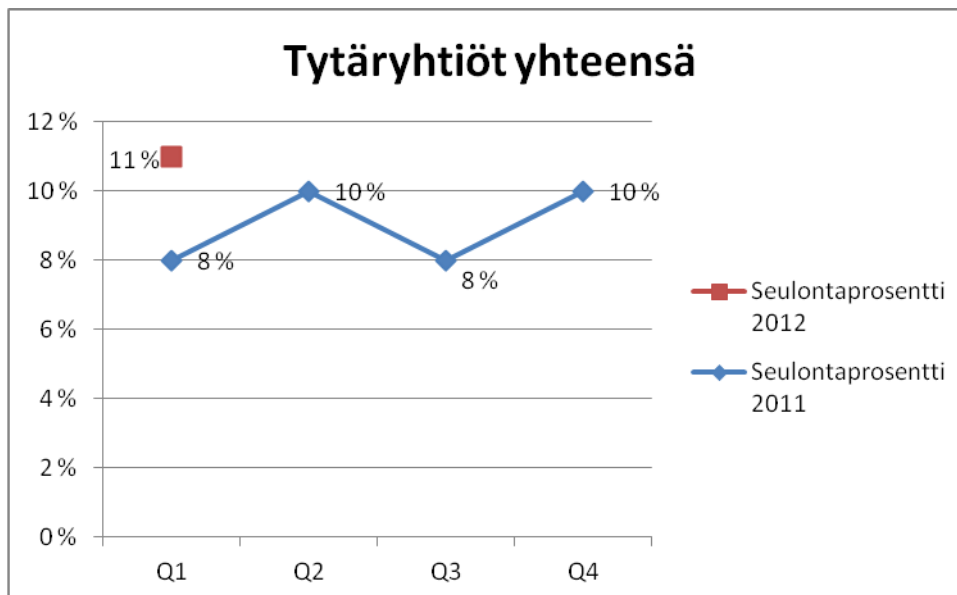
Kuva 25. Seulontaprosentin kehitys.
