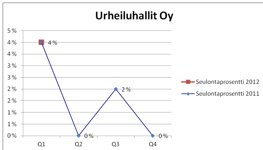
Kuva 162. Seulontaprocentin kehitys.
