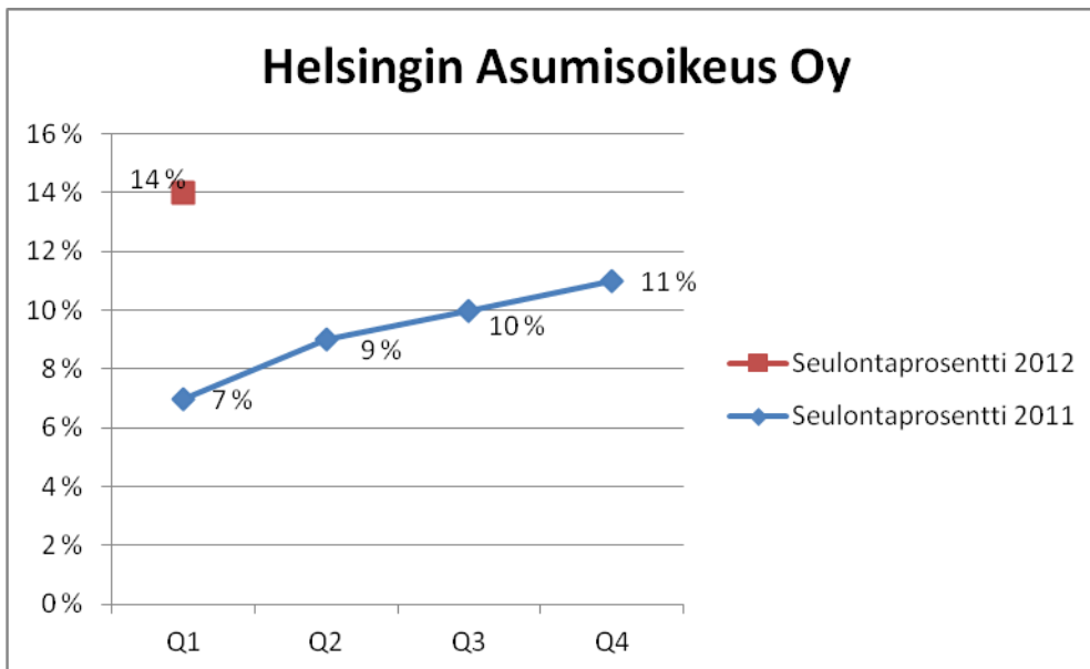
Kuva 116. Seulontaprosentin kehitys.
