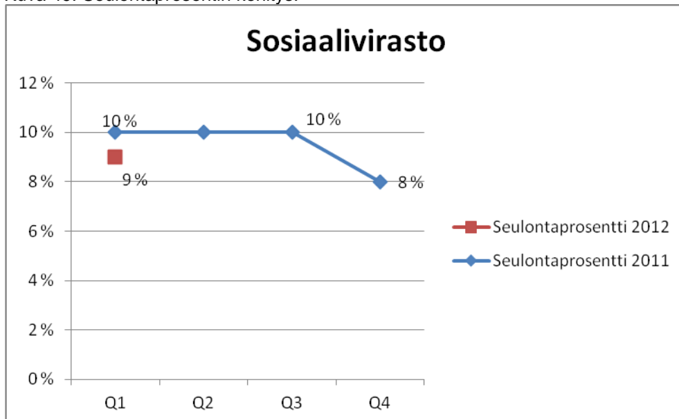
Kuva 49. Seulontaprosentin kehitys.
