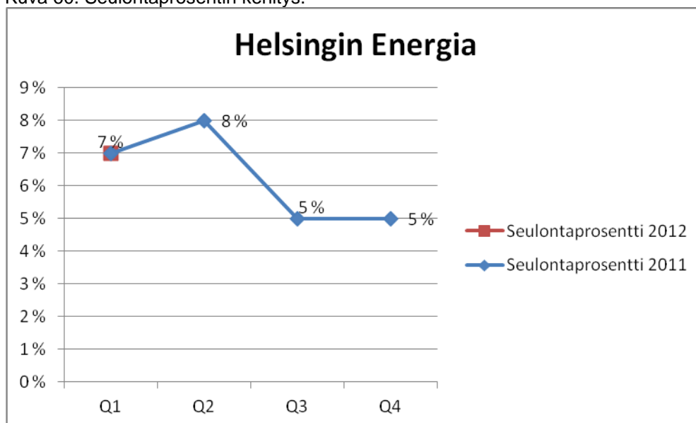
Kuva 60. Seulontaprosentin kehitys.
