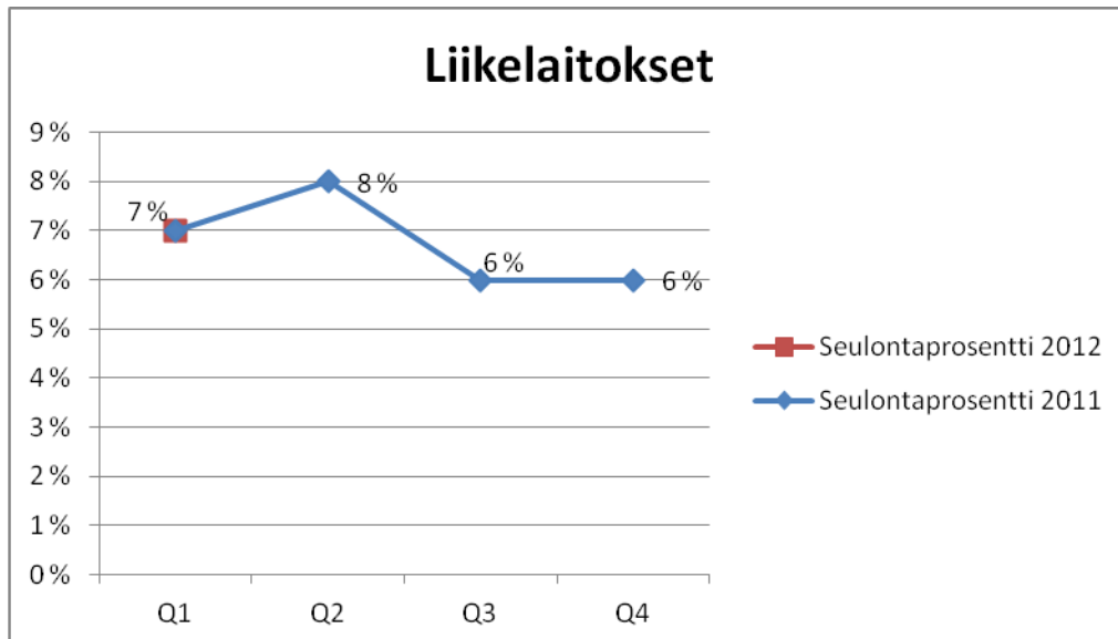
Kuva 19. Seulontaprocentin kehitys.
