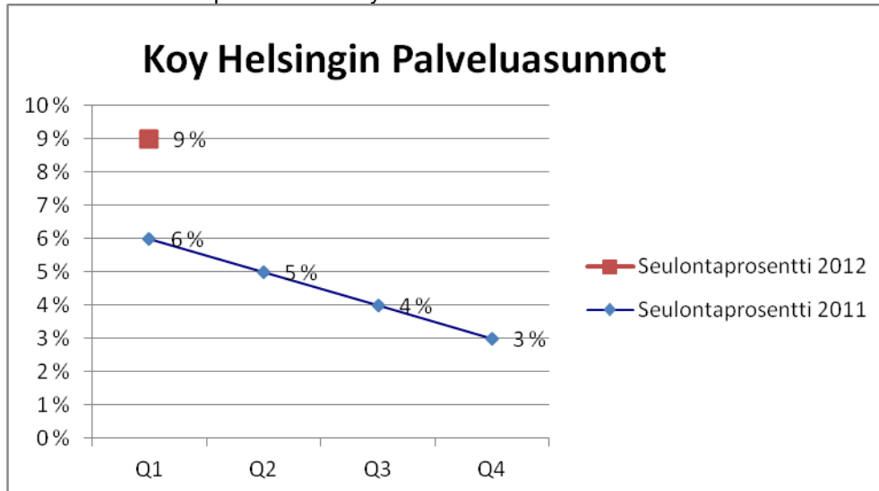
Kuva 128. Seulontaprosentin kehitys.
