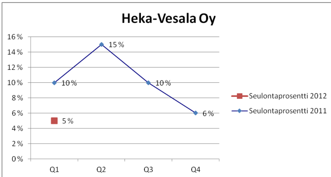
Kuva 112. Seulontaprosentin kehitys.
