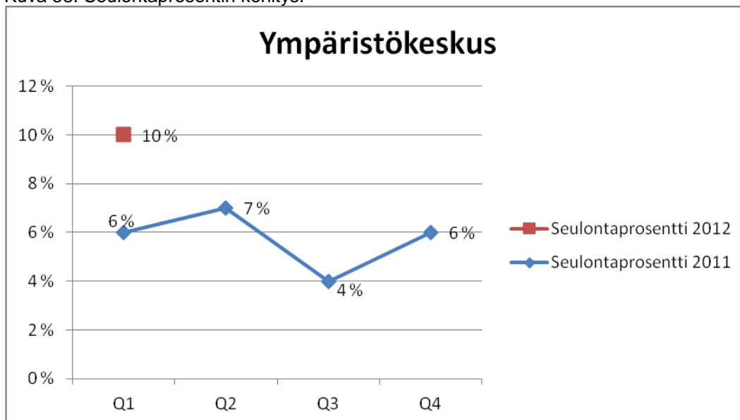
Kuva 58. Seulontaprosentin kehitys.
