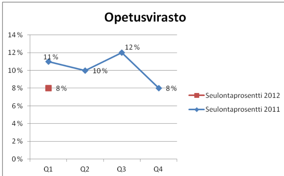
Kuva 45. Seulontaprocentin kehitys.
