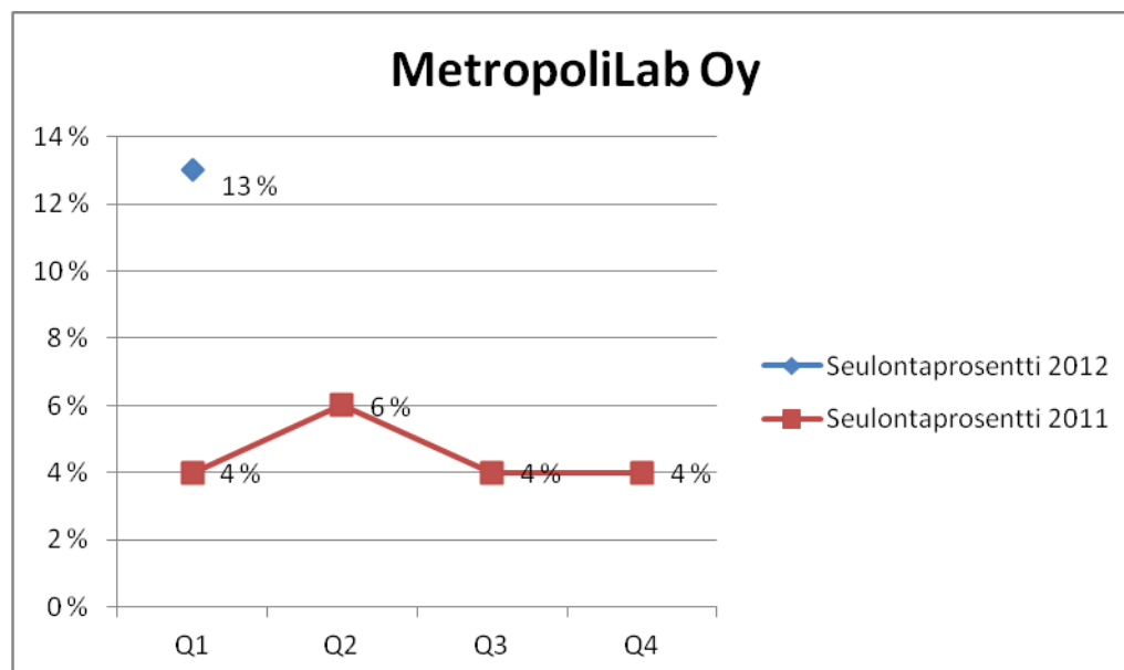
Kuva 143. Seulontaprosentin kehitys.
