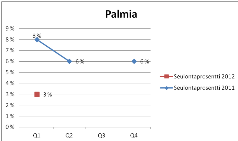
Kuva 68. Seulontaprocentin kehitys.
