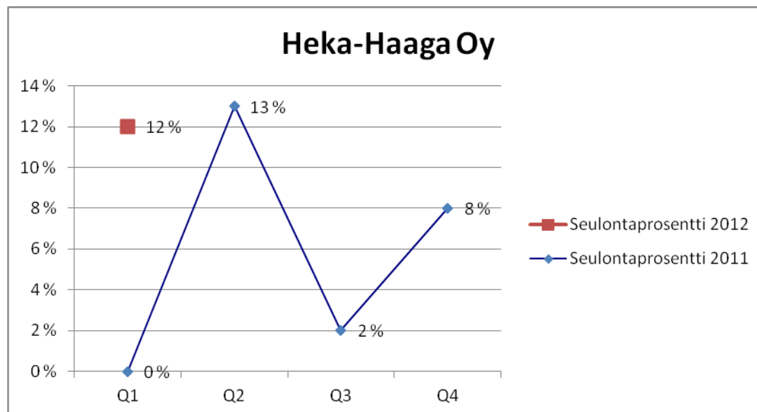
Kuva 85. Seulontaprosentin kehitys.
