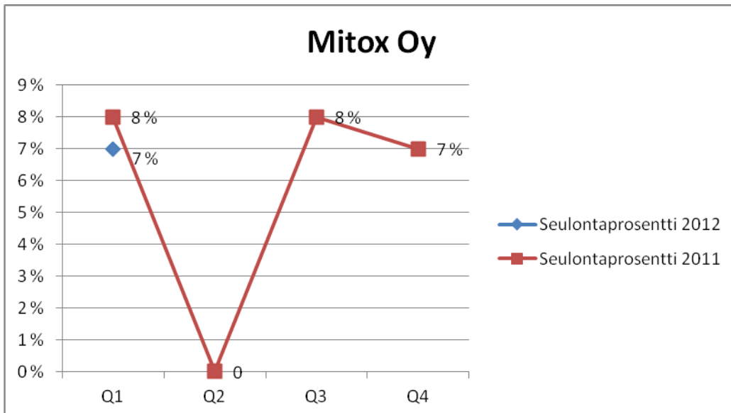
Kuva 145. Seulontaprosentin kehitys.
