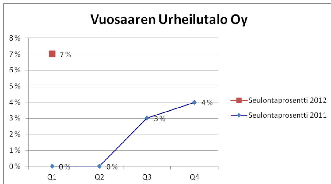
Kuva 165. Seulontaprosentin kehitys.
