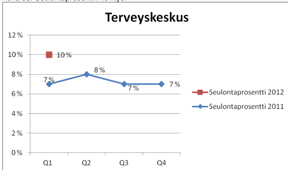
Kuva 55. Seulontaprosentin kehitys.
