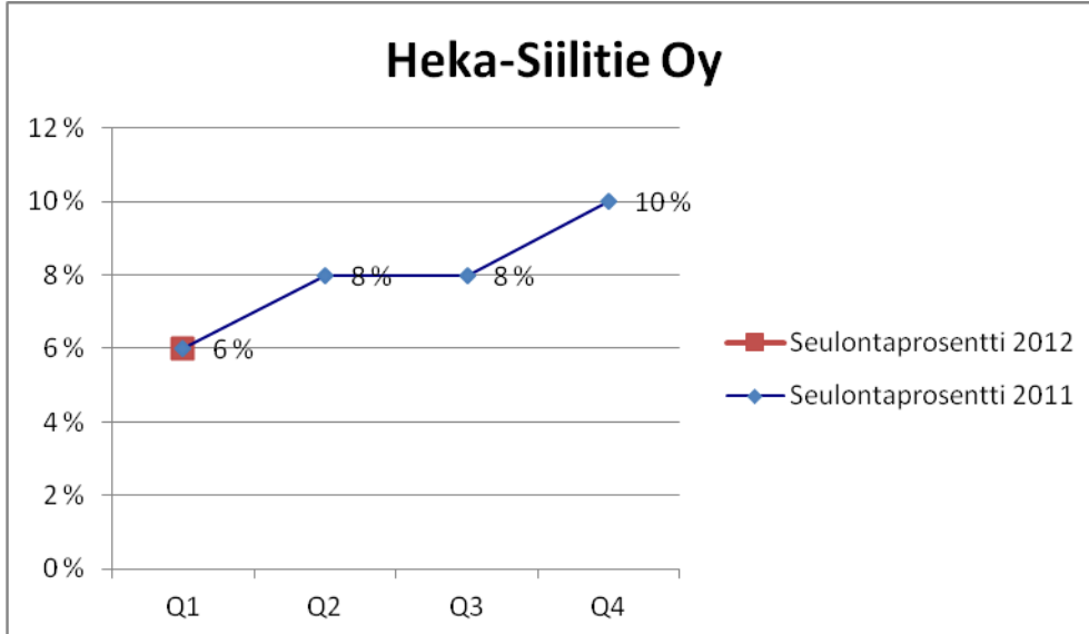
Kuva 108. Seulontaprosentin kehitys.
