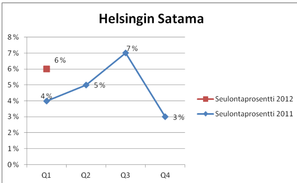
Kuva 62. Seulontaprosentin kehitys.
