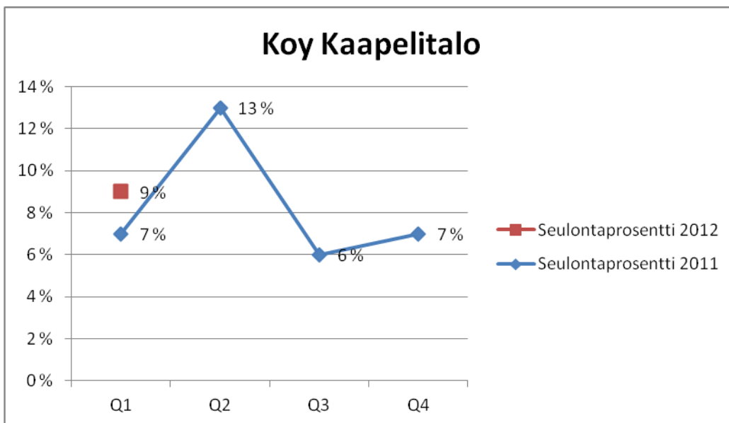
Kuva 138. Seulontaprosentin kehitys.
