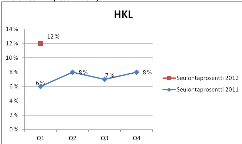
Kuva 64. Seulontaprocentin kehitys.
