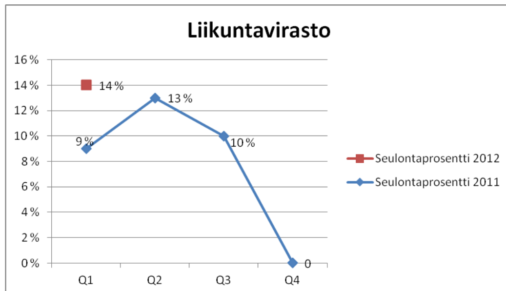
Kuva 43. Seulontaprosentin kehitys.
