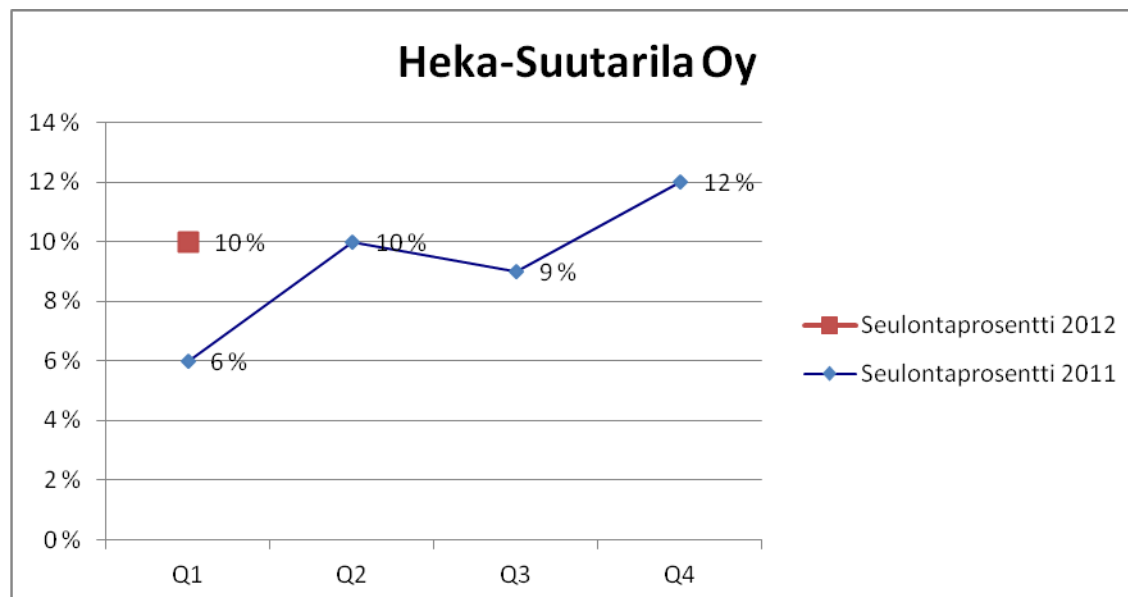
Kuva 110. Seulontaprosentin kehitys.
