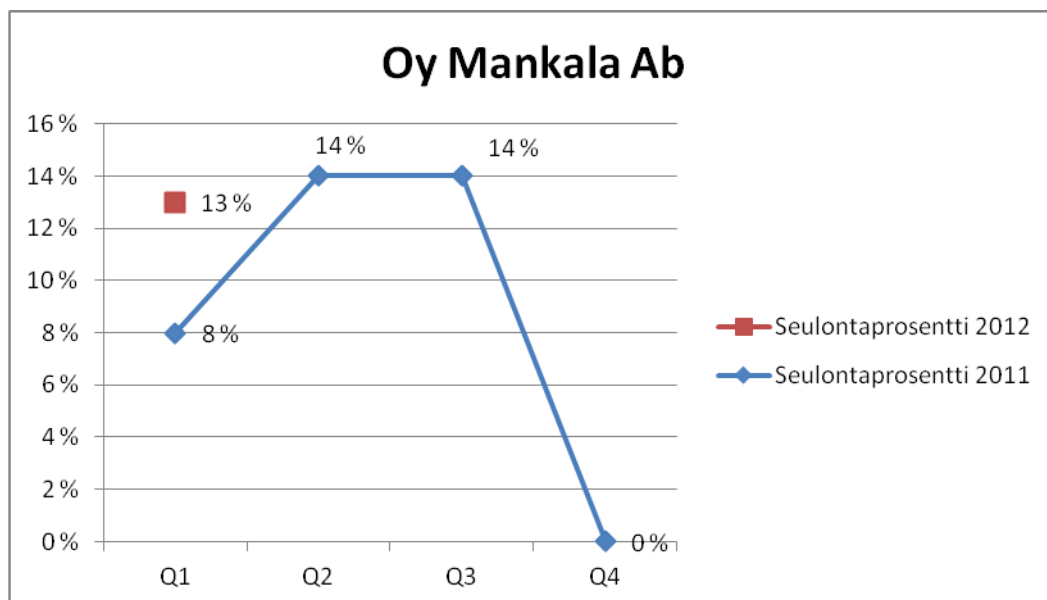
Kuva 141. Seulontaprosentin kehitys.
