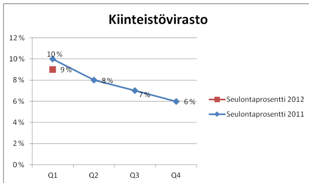
Kuva 46. Seulontaprosentin kehitys.
