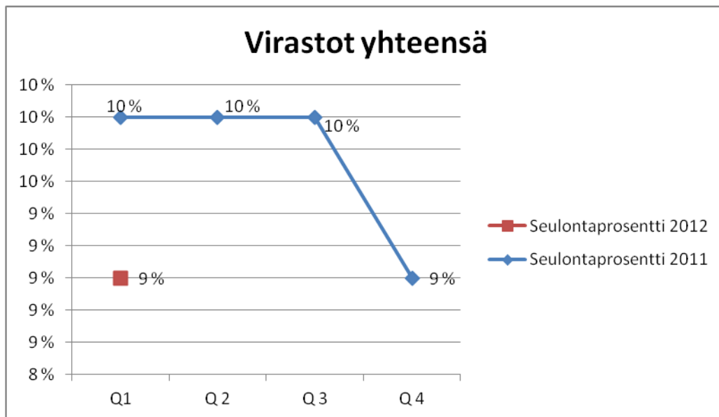
Kuva 16. Seulontaprosentin kehitys.
