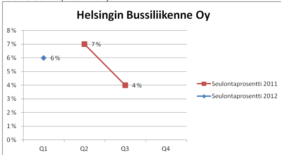
Kuva 119. Seulontaprosentin kehitys
