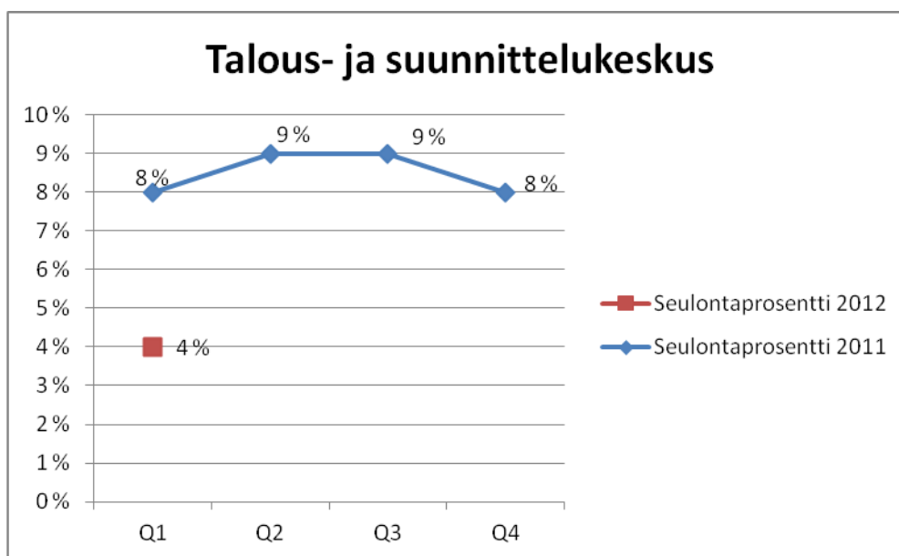
Kuva 51. Seulontaprosentin kehitys.
