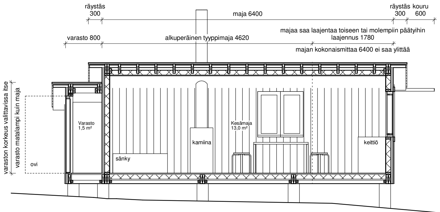
VANHAN TYYPIMAJAN LAAJENNUS, LEIKKAUS A
