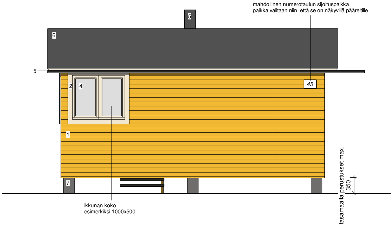
UUSI TYYPPIMAJA, TAKAA
