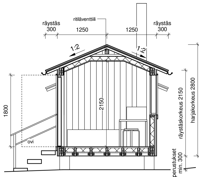
VANHAN TYYPIMAJAN LAAJENNUS, LEIKKAUS B
