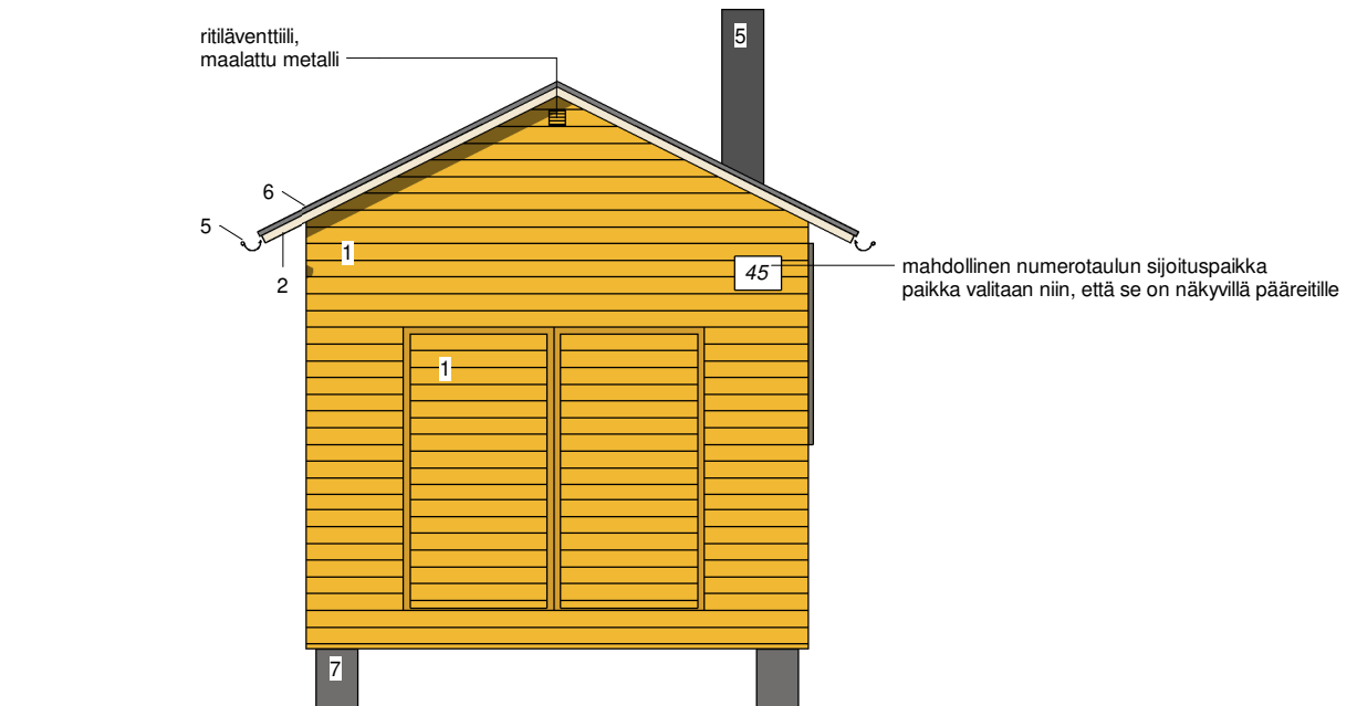
UUSI TYYPPIMAJA, SIVULTA
