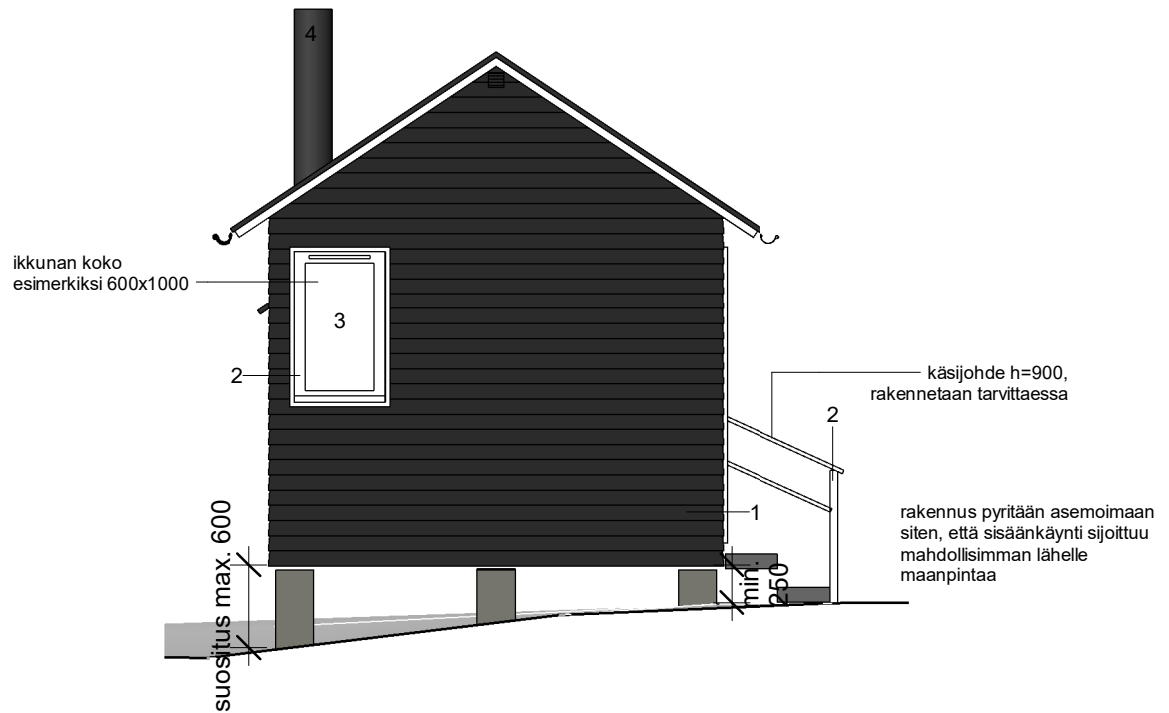
JULKISIVU, pääty 1:50
