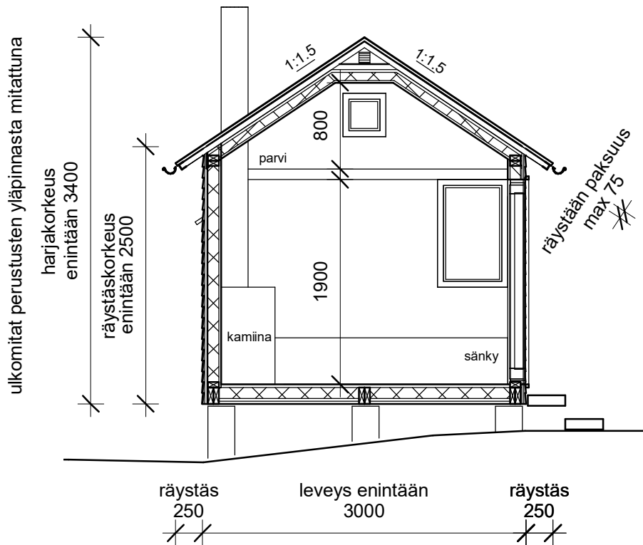
LEIKKAUS A-A 1:50
