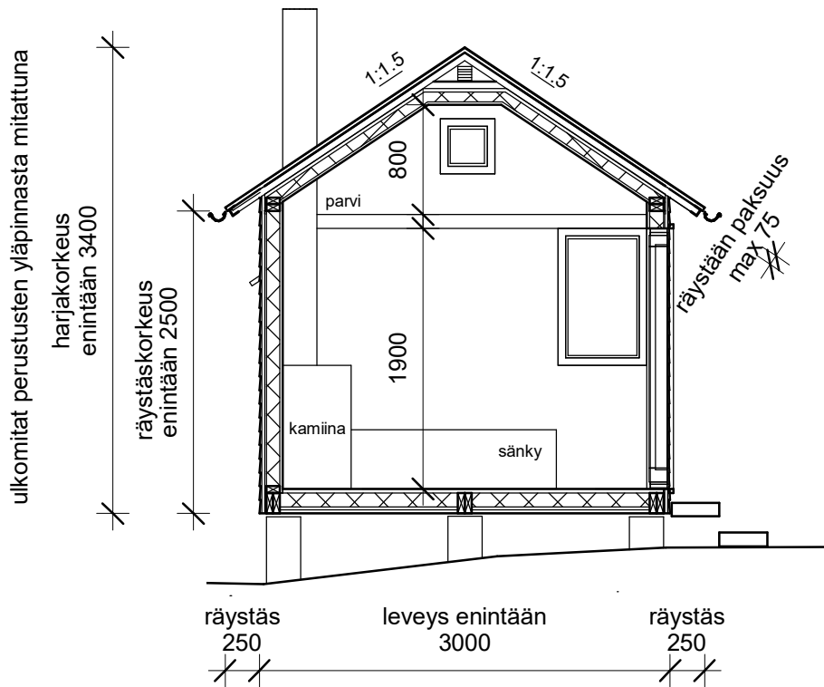
LEIKKAUS A-A 1:50
