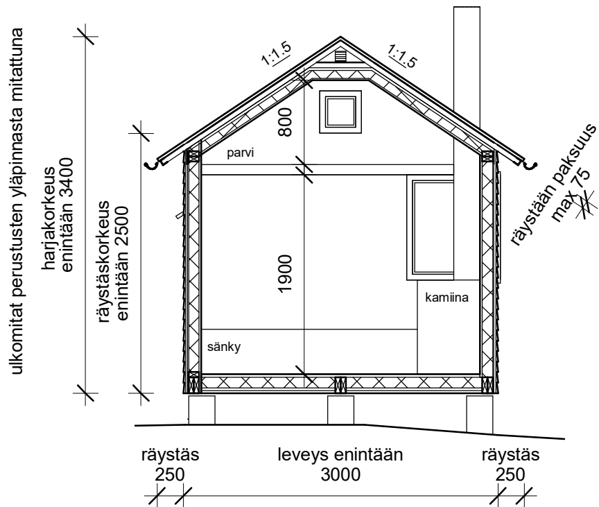
LEIKKAUS A-A 1:50
