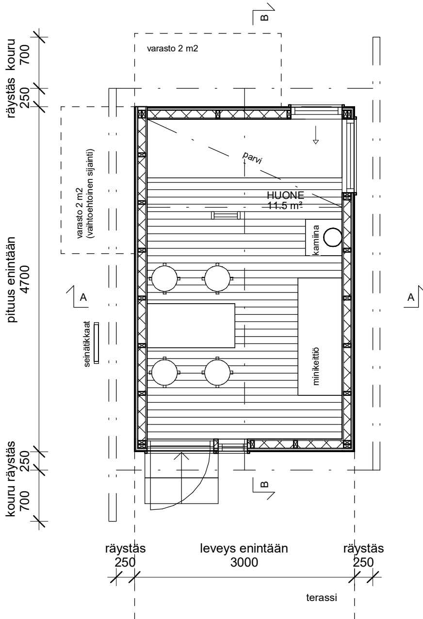
POHJAPIIRROS 1:50
