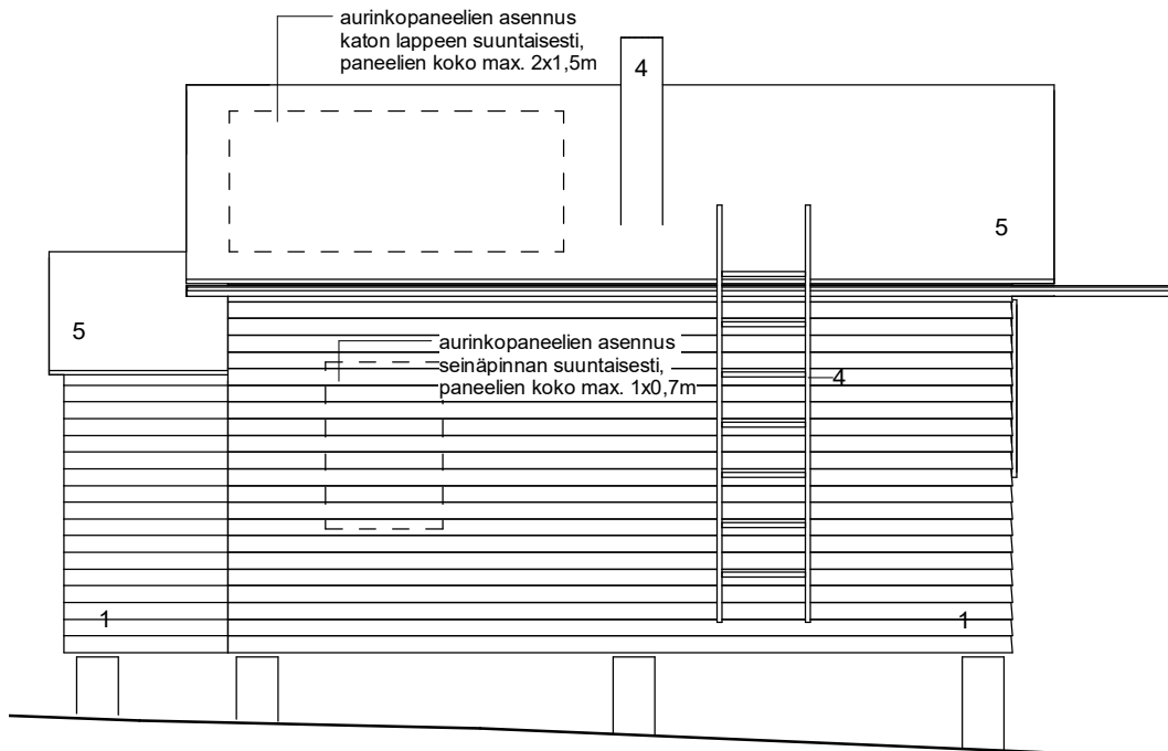
JULKISIVU, sisäänkäynti 1:50
