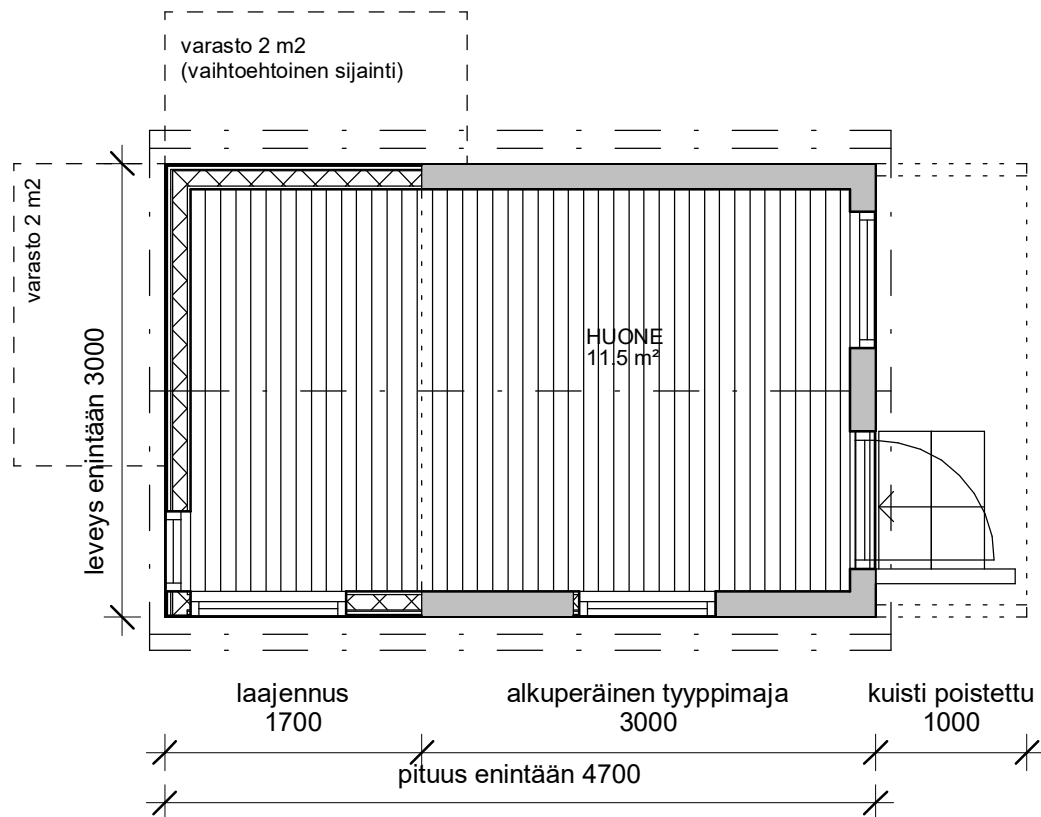
POHJAPIIRROS 1:50, laajennus päätyjulkisivun suuntaan, kuisti puretaan
