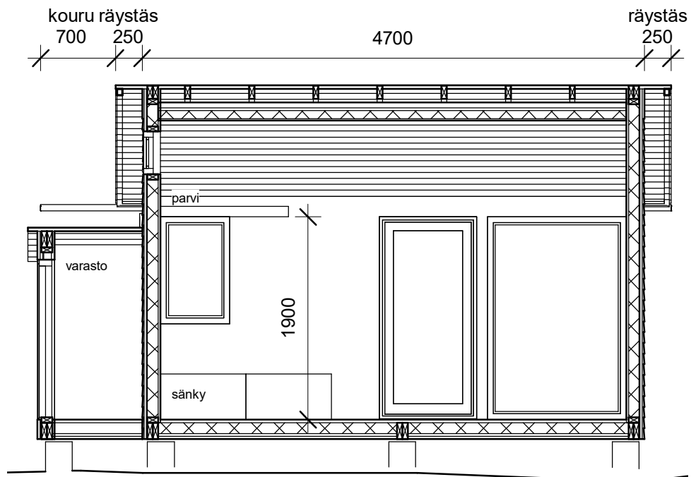
LEIKKAUS B-B 1:50
