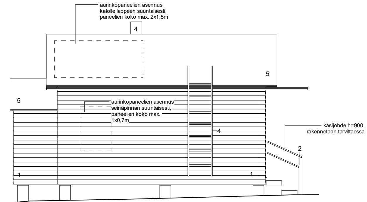
JULKISIVU, sivulta 1:50
