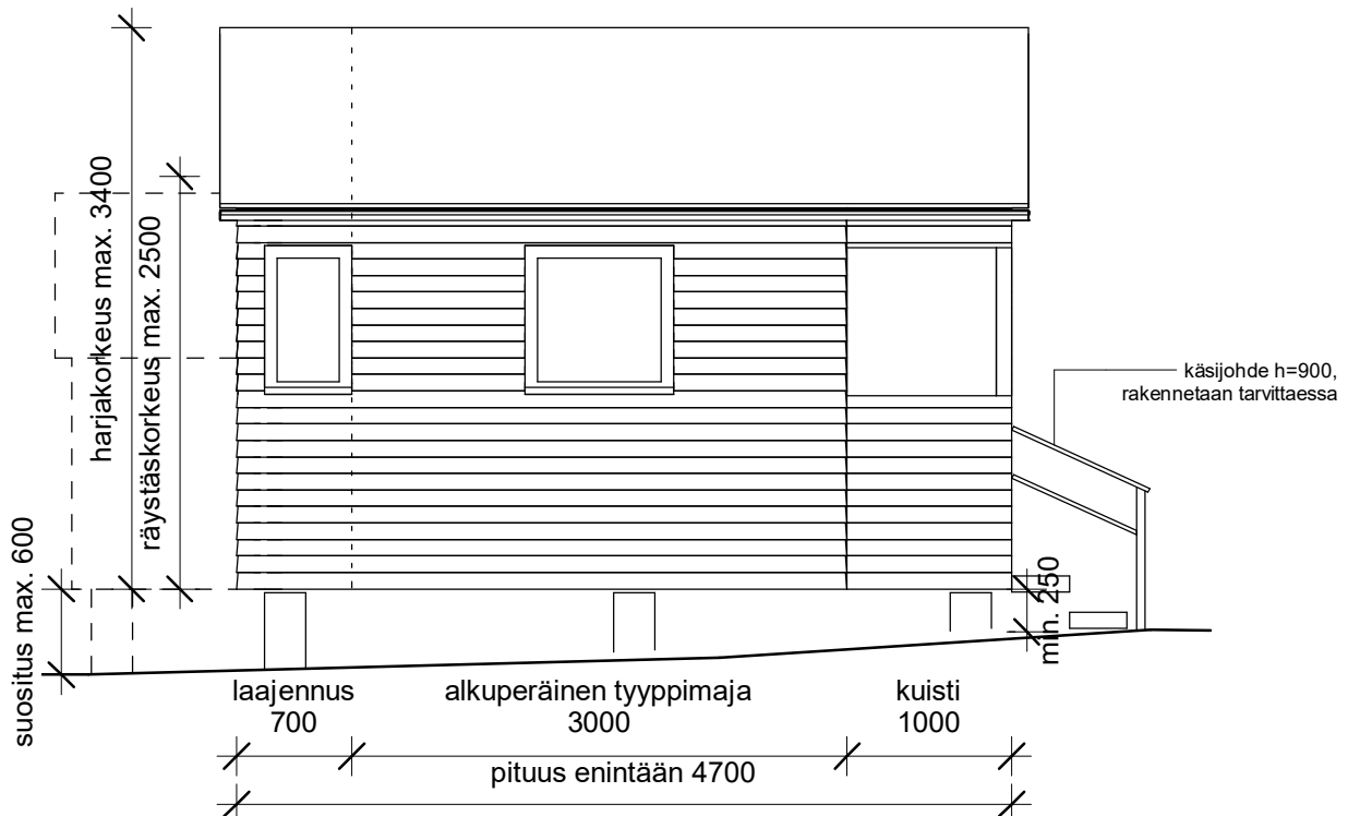
JULKISIVU 1:50, laajennus olemassa oleva kuisti säilyttäen
