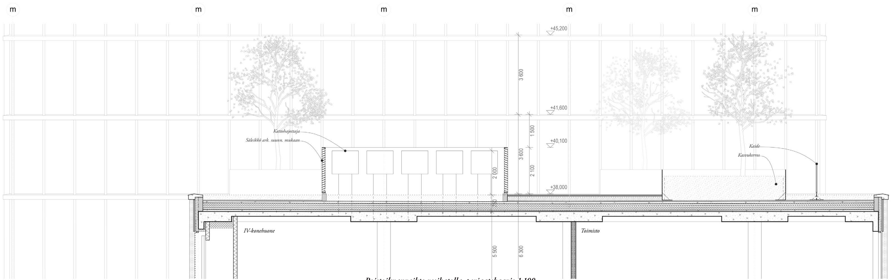
Poistoilmanvaihto vesikatolla, periaatekaavio 1:100
