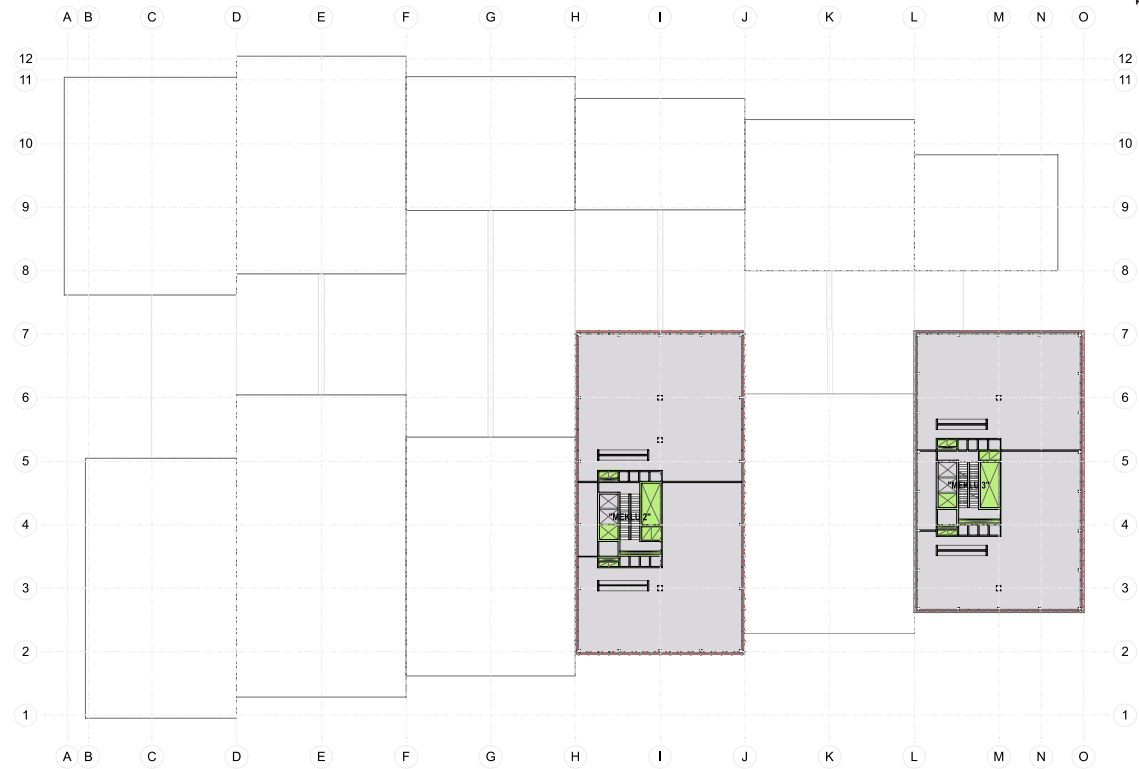
11.-kerros (+48,8)
