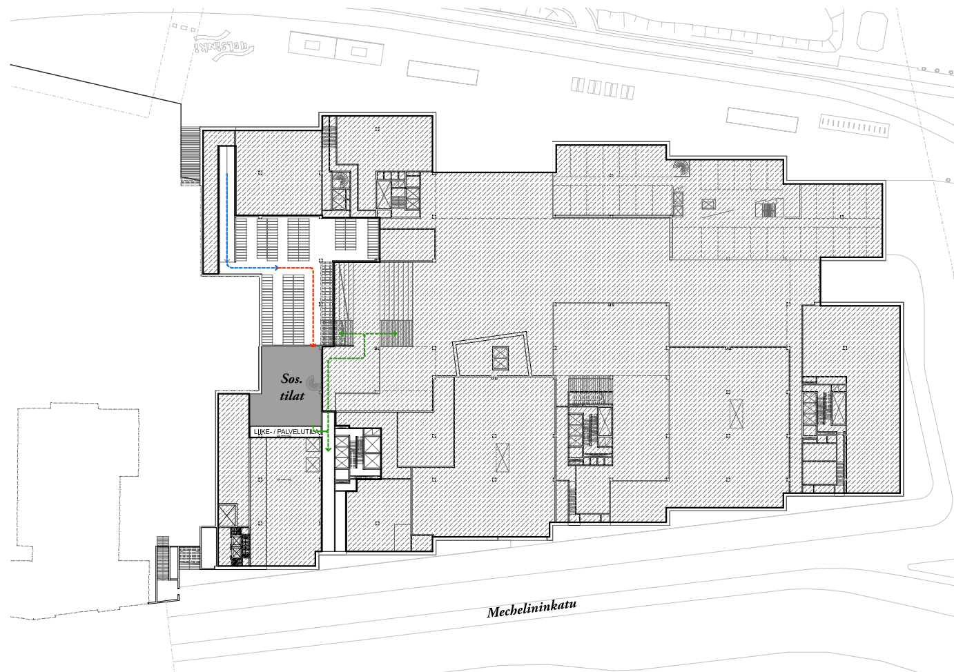
Polkupyöräpysäköinti parvitasolla
