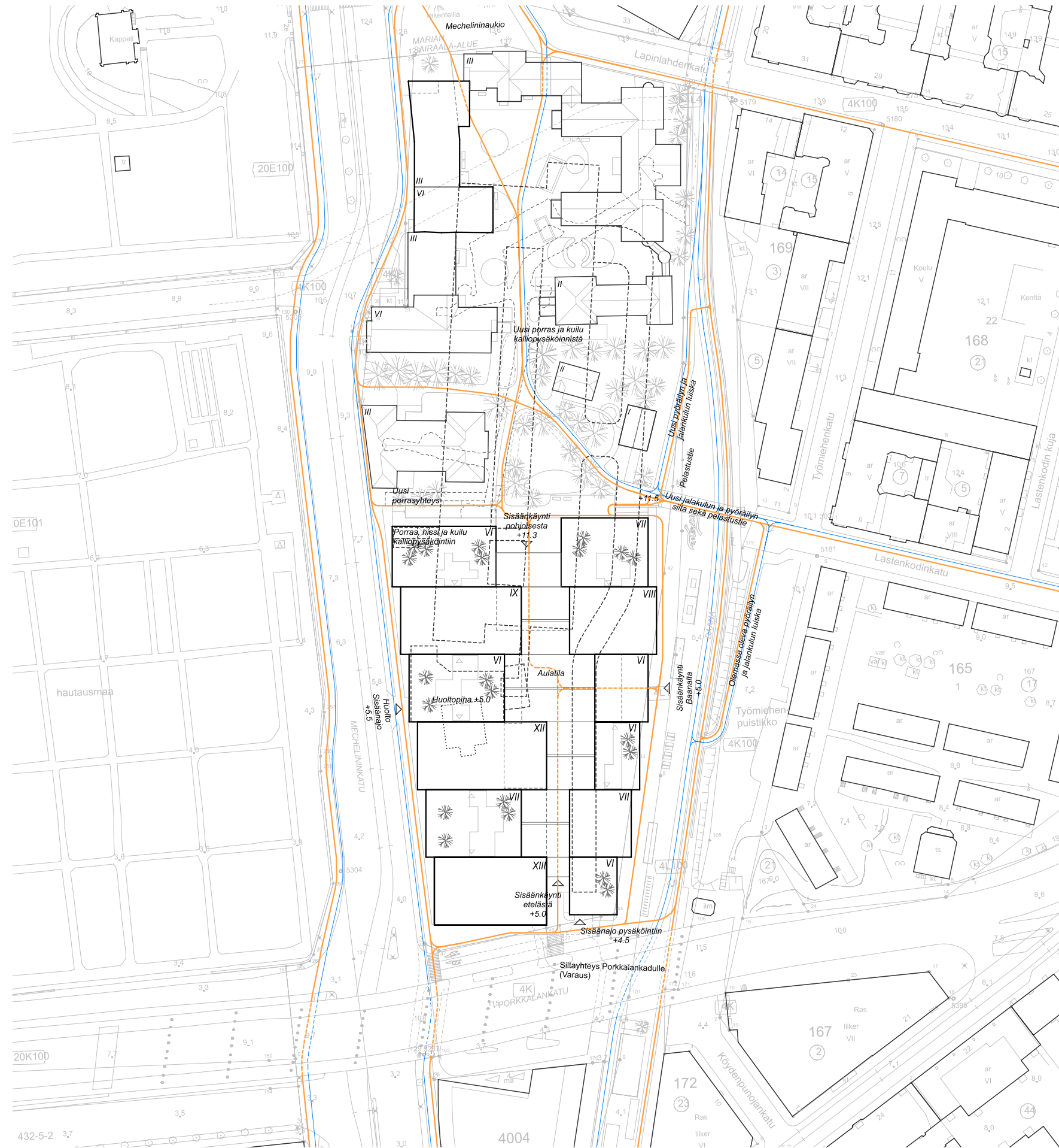
Liikennekaavio 1:1500
