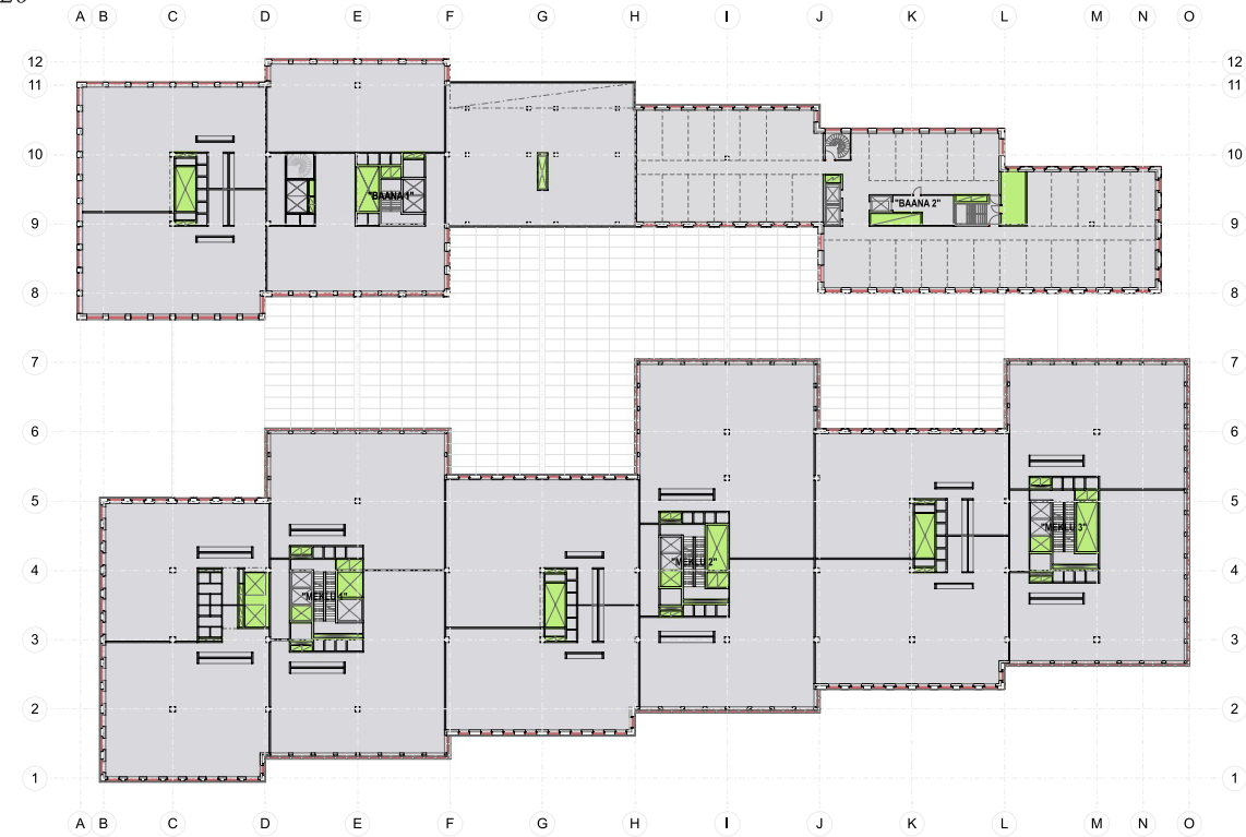
4.-kerros (+20,9)
