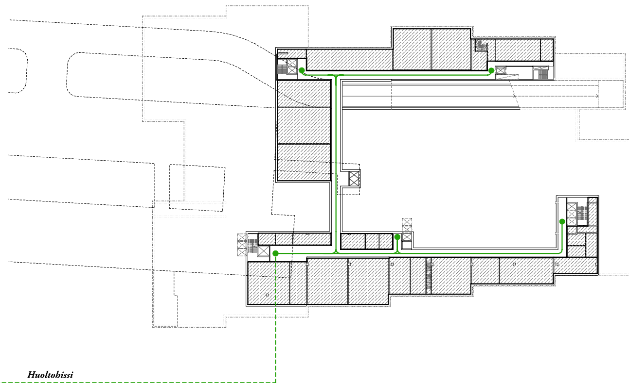
Huoltoyhteydet kellarikerroksessa
