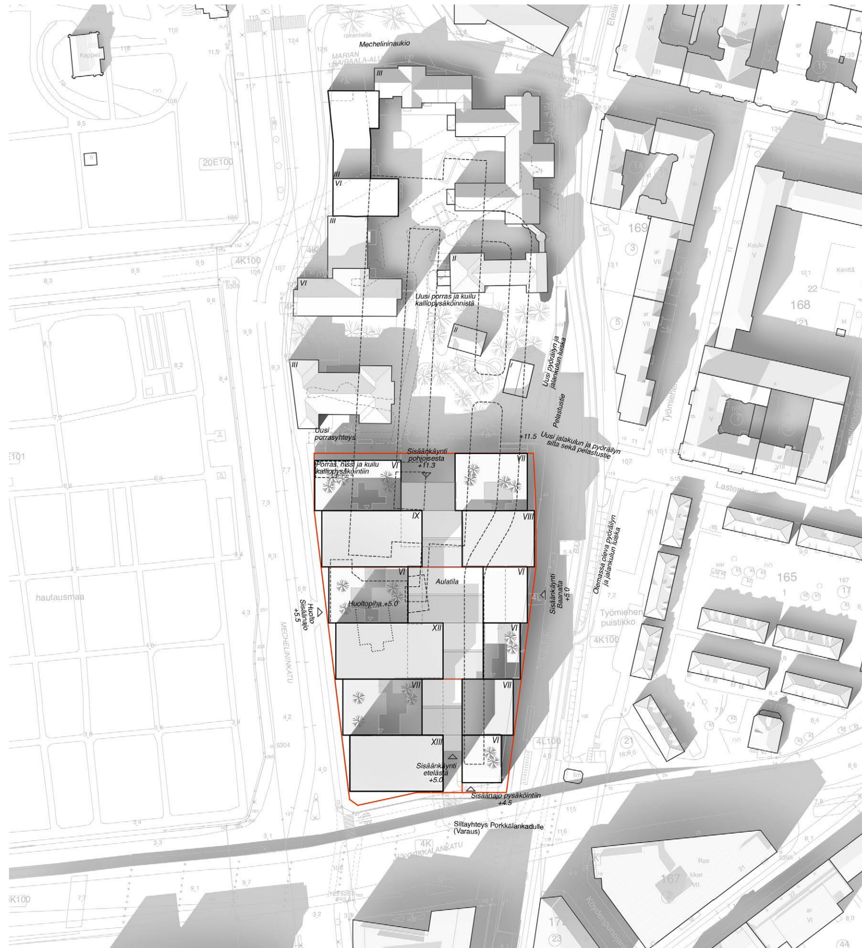
Asemapiirros 1:1500
