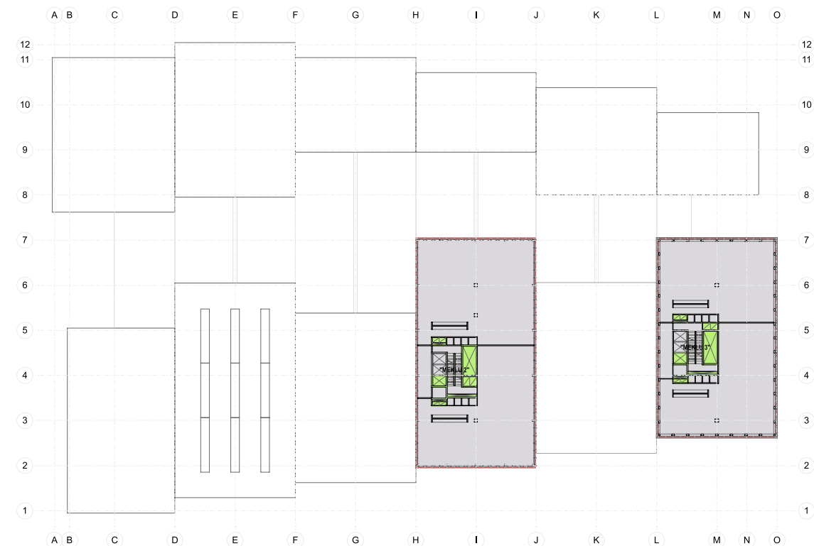
10.-kerros (+45,2)
