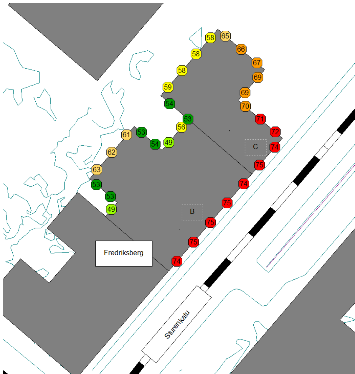
Kuva 1. Päiväkodin tilojen julkisivulle raitiotiestä kohdistuvat enimmäisäänitasot L_{AFmax} . Mallinnettu CadnaA-ohjelmistolla perustuen Articin tai vastaavan kaluston melupäästöön.
