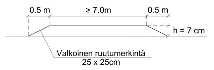
KOROTETTU SUOJATIE / KOROTETTU LIITTYMÄ POIKKILEIKKAUKSET 1:200
