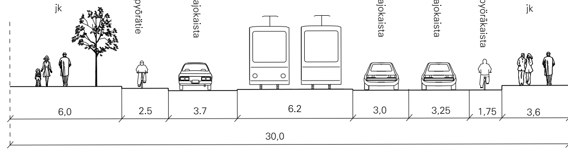
POIKKILEIKKAUS B-B 1:200
