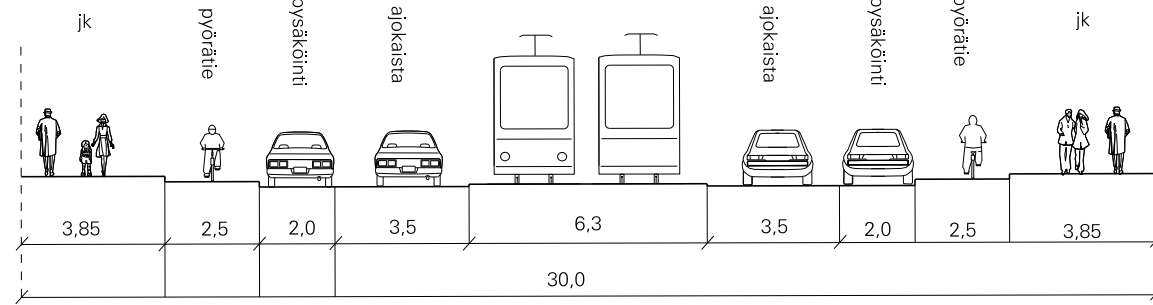
POIKKILEIKKAUS A-A 1:200
