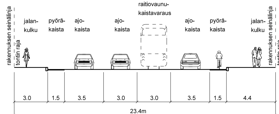
TYÖPAJANKATU D - D, 1:200
