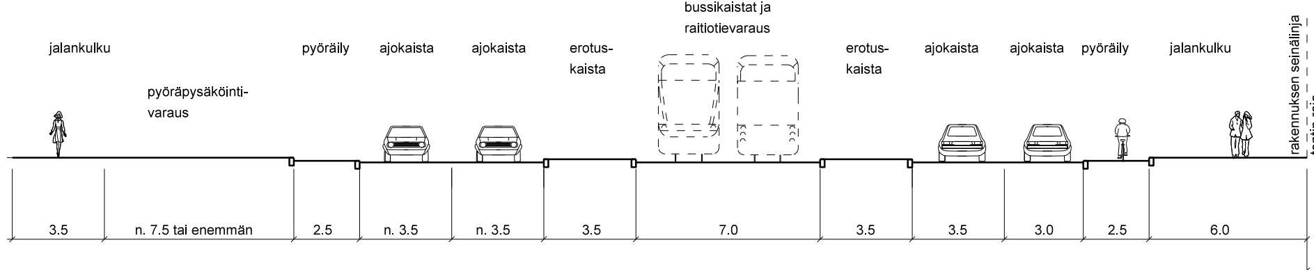
HERMANNIN RANTATIE B - B, 1:200
