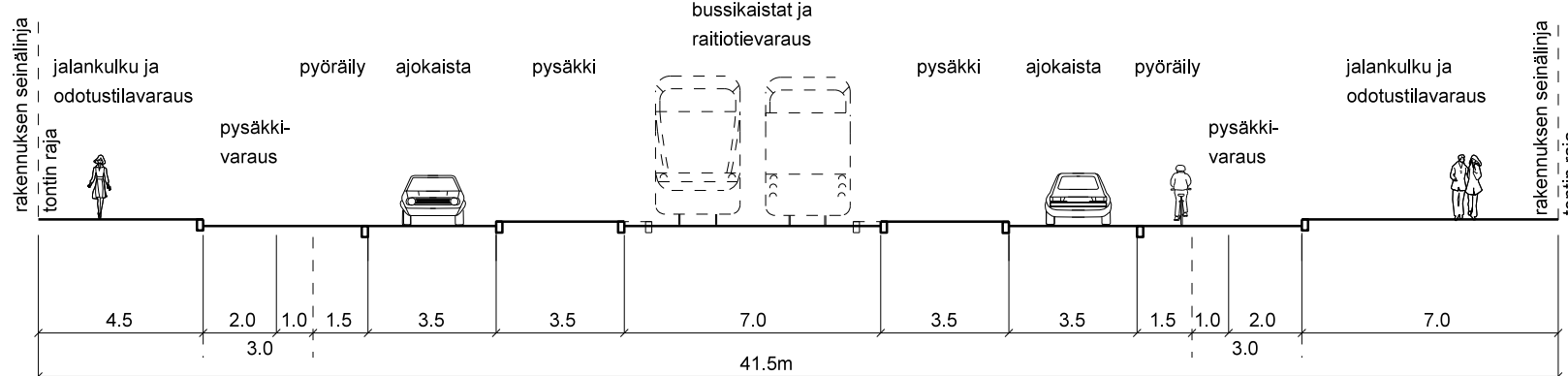
HERMANNIN RANTATIE A - A, 1:200
