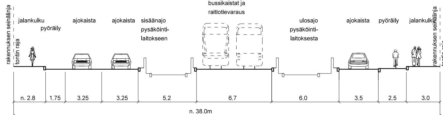
HERMANNIN RANTATIE C - C, 1:200
