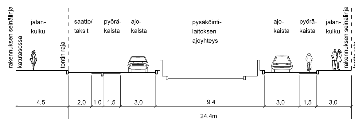
TYÖPAJANKATU E - E, 1:200
