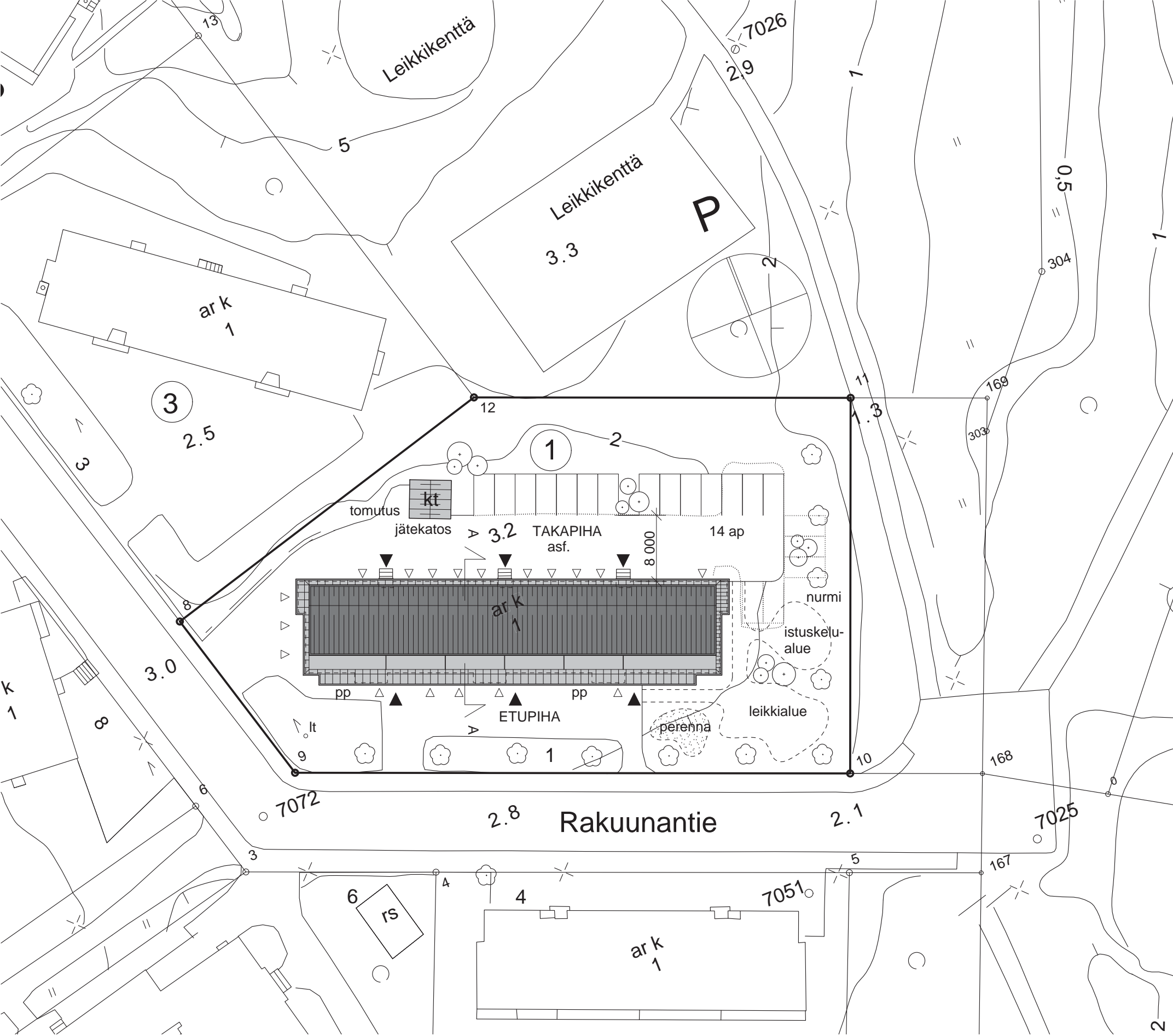
ASEMAPIIRUSTUS 1:500
