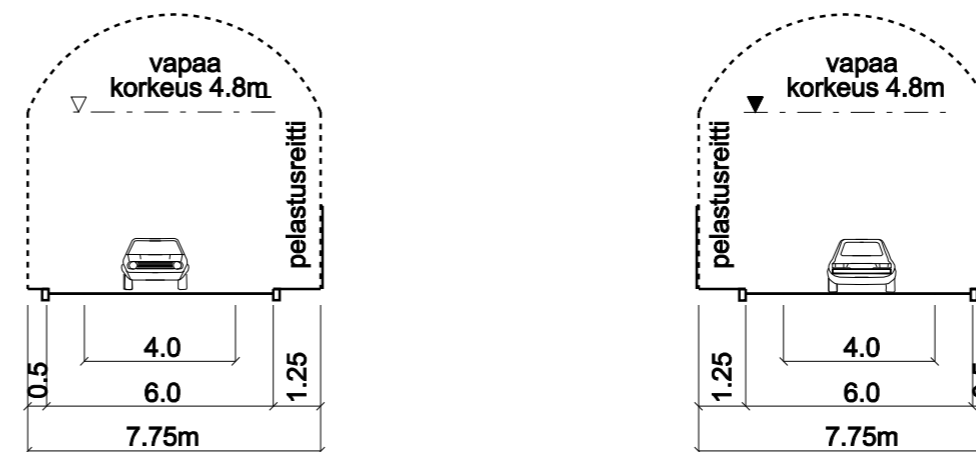
Tunnelin peruspoikkileikkaus 1:200
