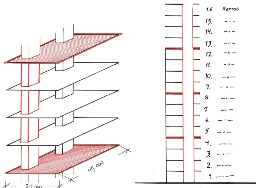
Kuva: Havainnekuva työnaikaisten palo-osastointien järjestämisestä. Osastointi EI 60 (pun.)
