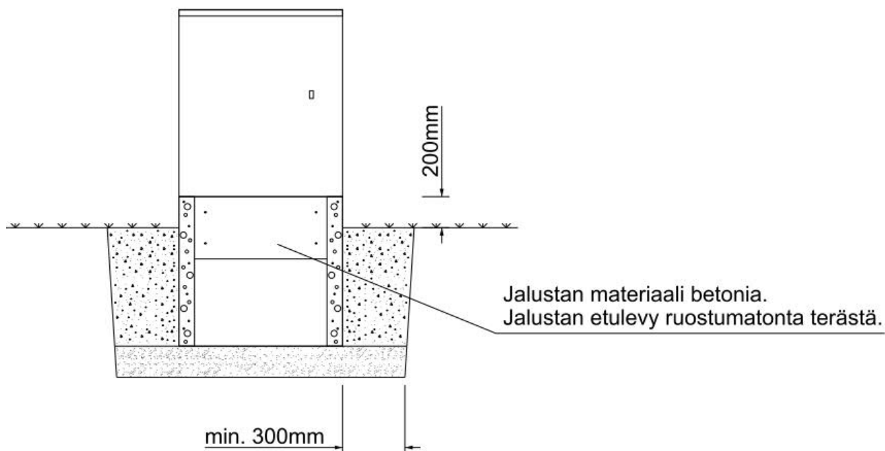
Kuva 13. Ulkovalaistuskeduksen asennusperiaate edestä.
