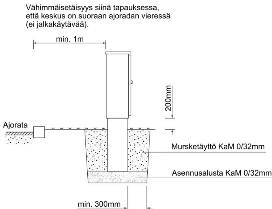
Kuva 12. Ulkovalaistuskeskuksen asennusperiaate sivulta.
