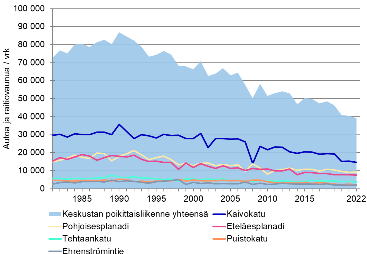
Kuva 15. Keskustan poikittaisen moottoriajoneuvoliikenteen pitkän aikavälin kehitys.
