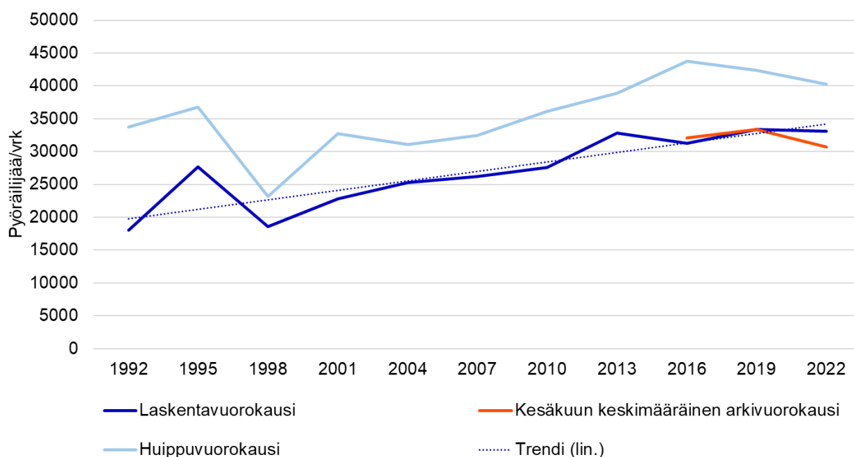
Kuva 9. Pyöräliikennemäärä Helsingin kantakaupungin rajalla 1992–2022 kesäkuun arkivuorokauden käsin-laskennoissa laskentavuorokautena, kesäkuun keskimääräisenä arkivuorokautena sekä kesän huippuvuorokautena.
