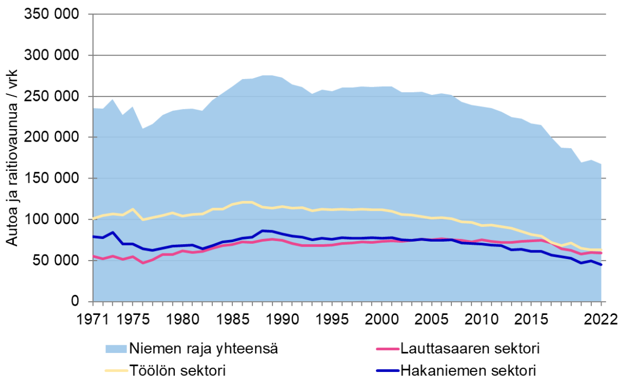
Kuva 14. Moottoriajoneuvoliikenteen pitkän aikavälin kehitys niemen rajalla.
