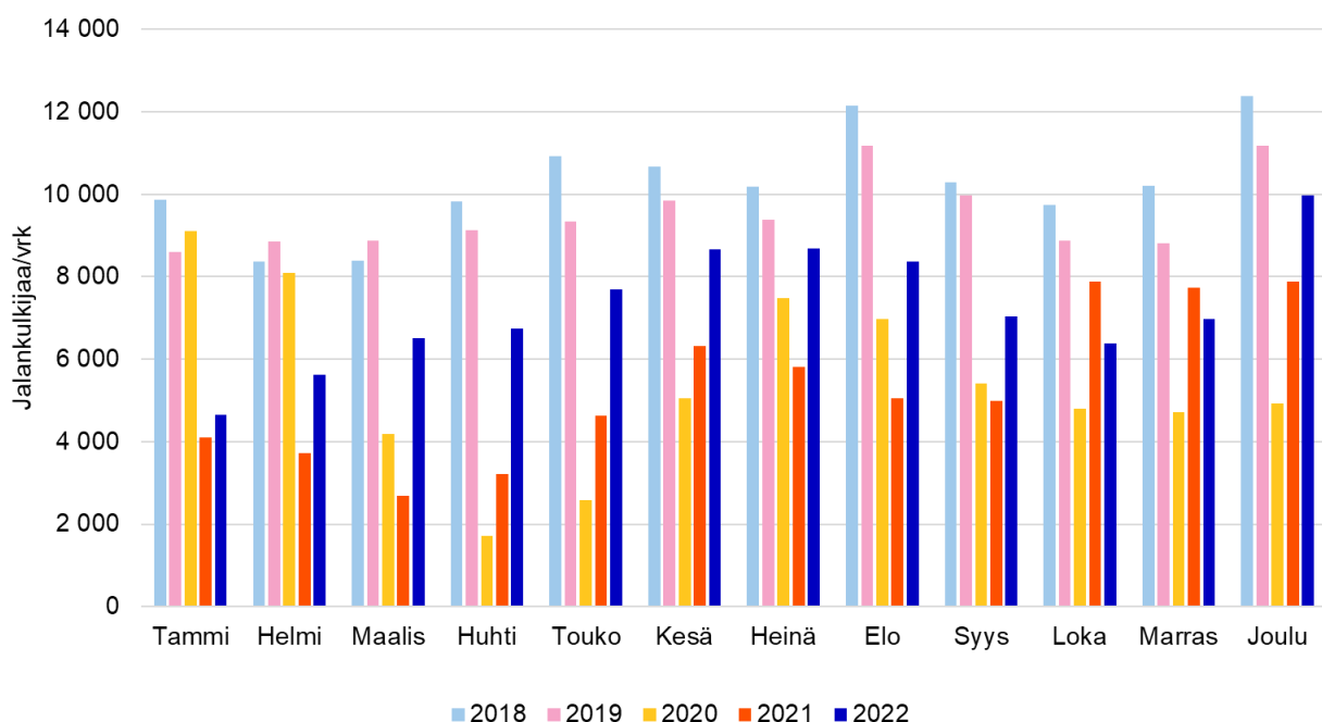
Kuva 7. Kuukauden keskimääräinen jalankulkijamäärä vuorokaudessa Aleksanterinkadun laskentapisteessä vuosina 2018–2022.
