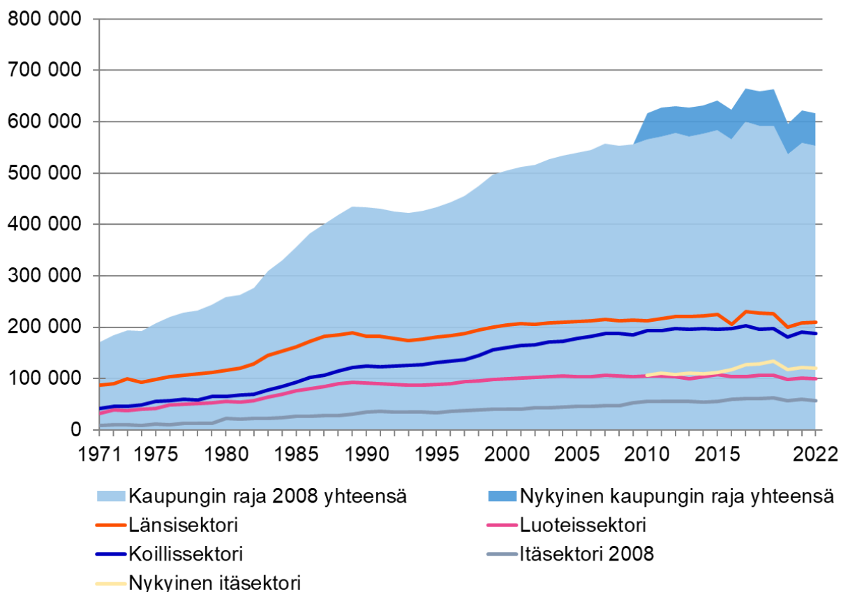
Kuva 17. Moottoriajoneuvoliikenteen pitkän aikavälin kehitys kaupungin rajalla.
