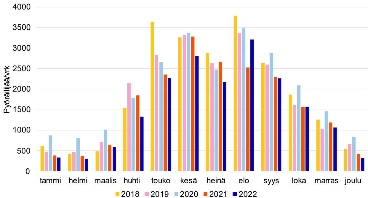
Kuva 11. Kuukauden keskimääräinen vuorokausiliikenne vuosina 2018–2022 (laskettu 14 konelaskentapisteen keskiarvona), pyörää/vrk.
