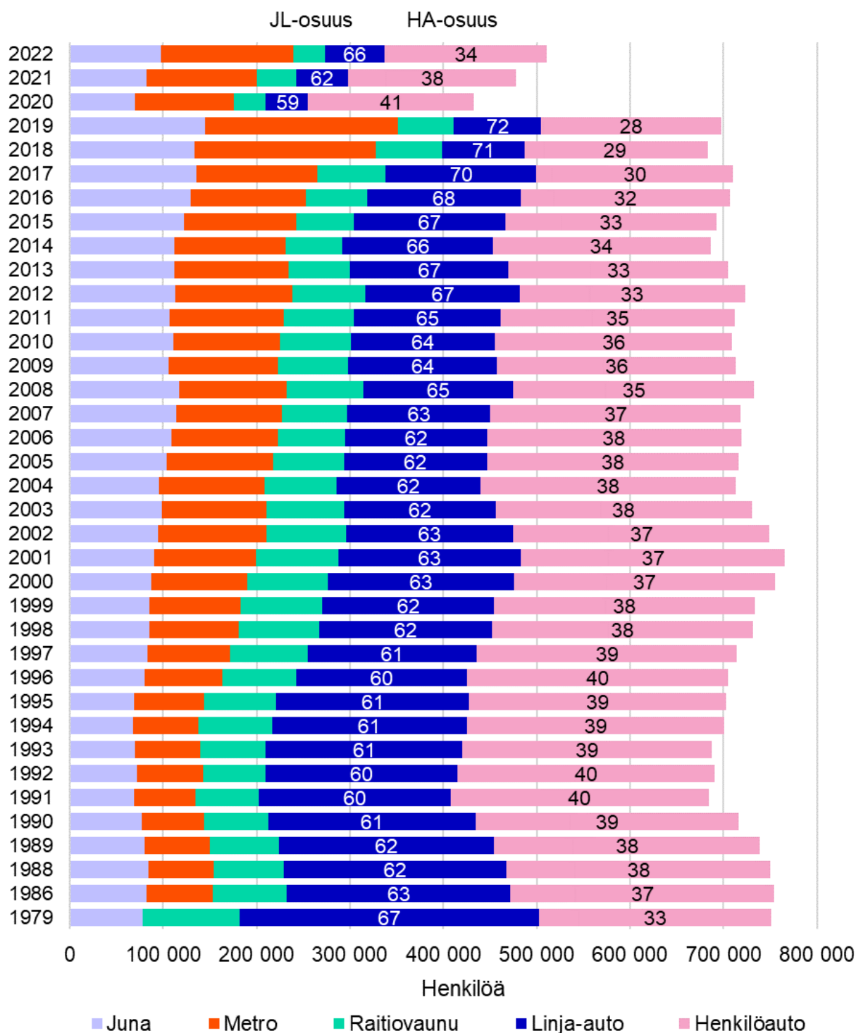
Kuva 2. Syksyn henkilöliikenteen matkustajamäärä kulkutavoittain ja henkilöautoliikenteen ja joukkoliikenteen osuudet niemen rajalla 1979–2022, %, koko vuorokausi, molemmat suunnat.
