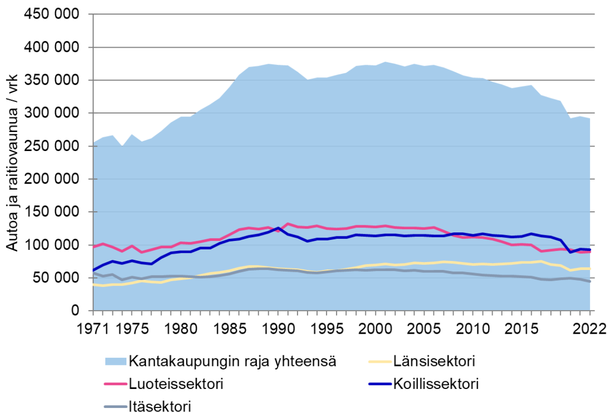
Kuva 16. Moottoriajoneuvoliikenteen määrien pitkän aikavälin kehitys kantakaupungin rajalla.
