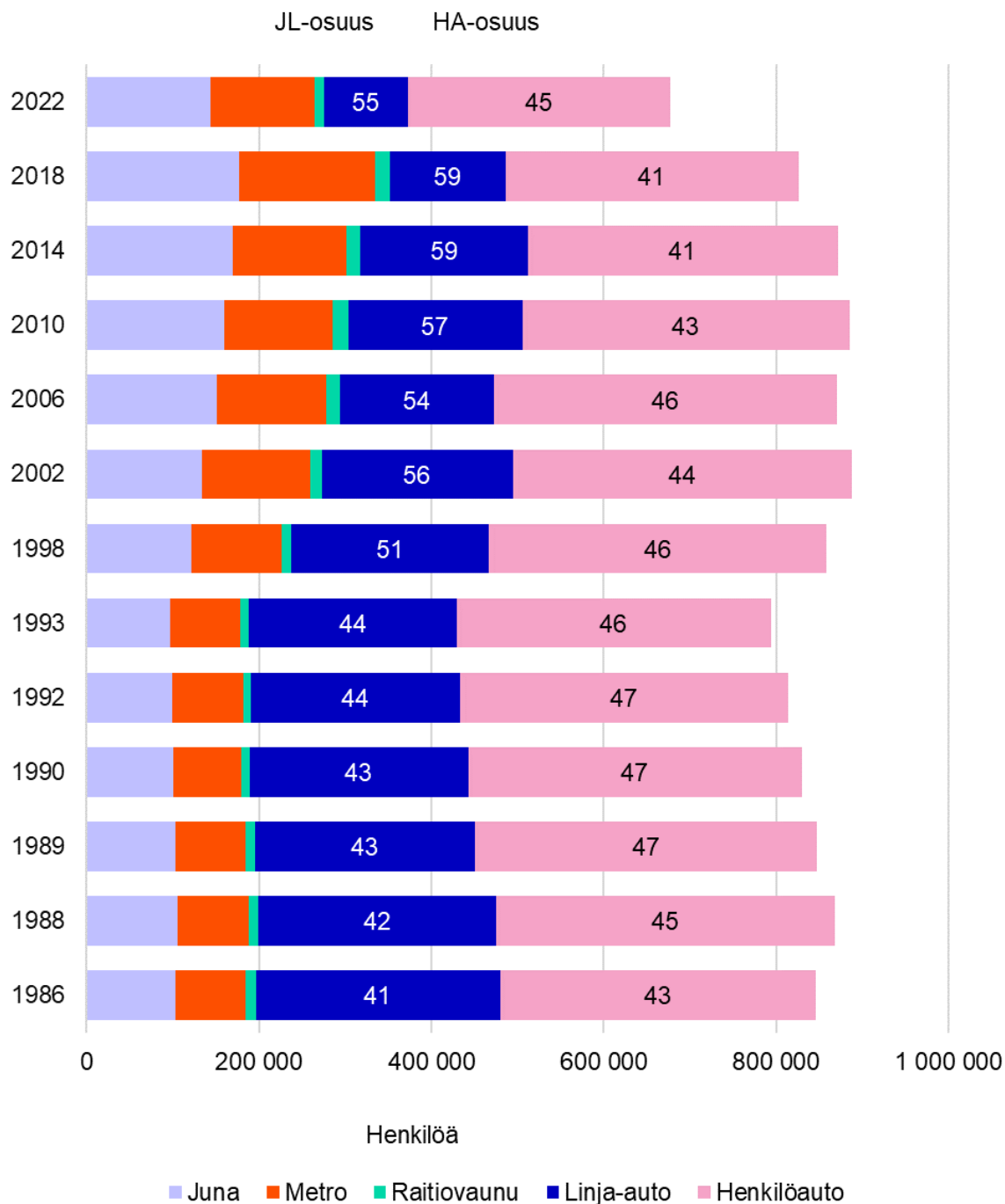
Kuva 4. Syksyn henkilöliikenteen matkustajamäärä kulkutavoittain ja henkilöautoliikenteen ja joukkoliikenteen osuudet kantakaupungin rajalla 1986–2022, %.
