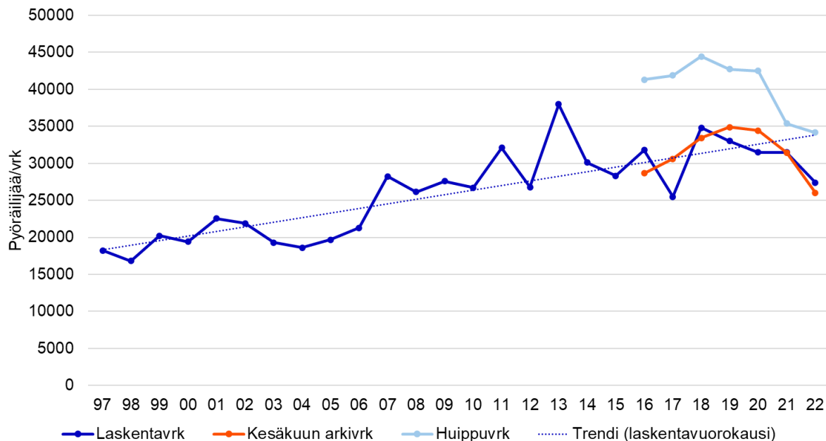
Kuva 8. Pyöräliikennemäärä Helsingin niemen rajalla 1997–2022 kesäkuun arkivuorokauden käsin-laskennoissa laskentavuorokautena, kesäkuun keskimääräisenä arkivuorokautena sekä kesän huippuvuorokautena.
