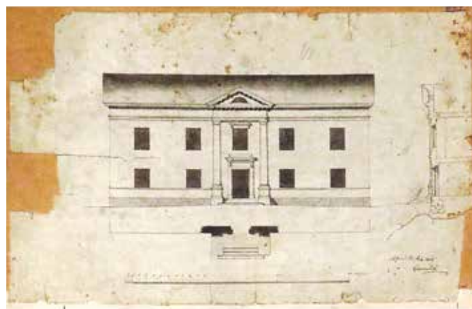
Kuva 13. Asuinrakennukseksi kunnostetun polttorakennuksen julkisivupiirros. Pehr Granstedt 1815. Skannaus kirjasta Herttoniemen kartano, alkuperäinen lähde SOV (Svenska Odlingens vänner).
