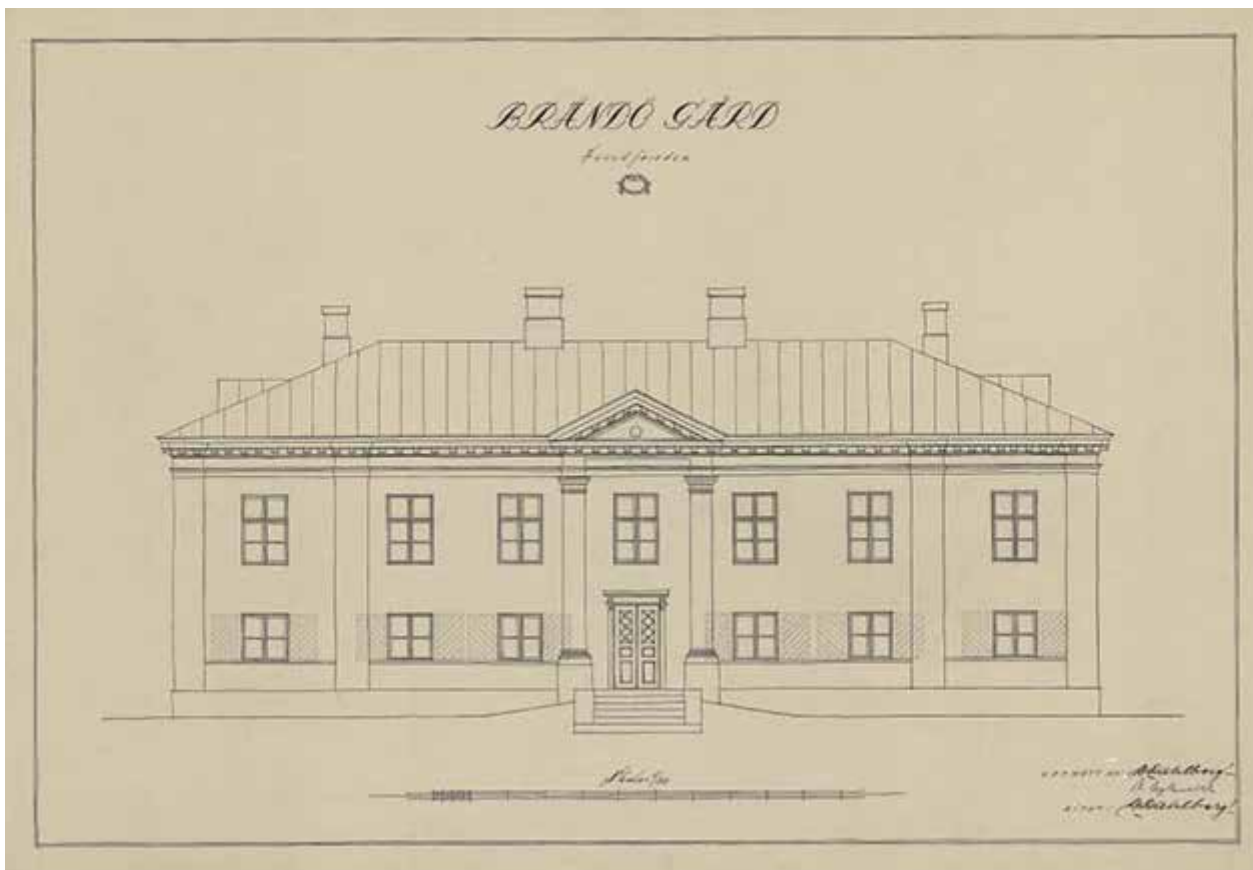
Kuva 12. Mittauspiirustus kartanon päärakennuksesta vuodelta 1922-23. Piirtäjä D. Dahlberg. AKR.
