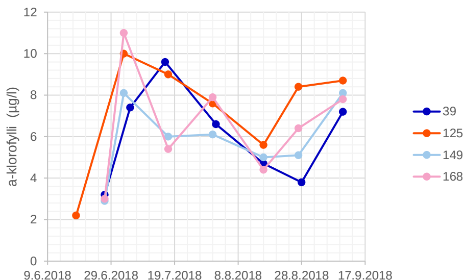
Kuva 5. Typenpoistohäiriön aikainen pintaveden a-klorofyllin pitoisuudet pääkaupunkiseudun merialueen yhteistarkkailun näyteasemilla etäällä purkupaikasta (114, 123, 148, 147) ja sen lähistöllä (39, 125, 149, 168).
