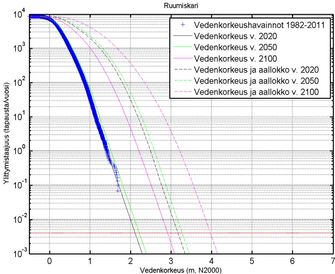
Kuva 130. Tuntihavaintoihin pohjautuva vedenkorkeuden ja aallonkorkeuden yhteisvaikutuksen arvioiminen Ruumiskarilla vuosille 2020, 2050 ja 2100. Pelkkä vedenkorkeusarvo on yksikössä tuntihavaintoja vuodessa, mutta kun tähän arvoon lisätään aallokko, on on lopputulos tapausta vuodessa. Punainen vaakaviiva on tässä raportissa käytetty todennäköisyystaso 1/250 tapausta vuodessa.
