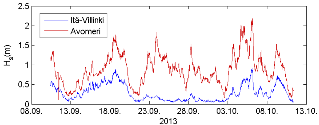
Kuva 98. Merkitsevä aallonkorkeus Itä-Villingissä ja avomerellä Helsingin edustalla.
