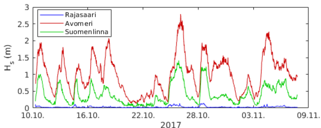
Kuva 126. Merkitsevä aallonkorkeus Rajasaaren poijulla, Suomenlinnan poijulla ja Helsingin avomeren poijulla.
