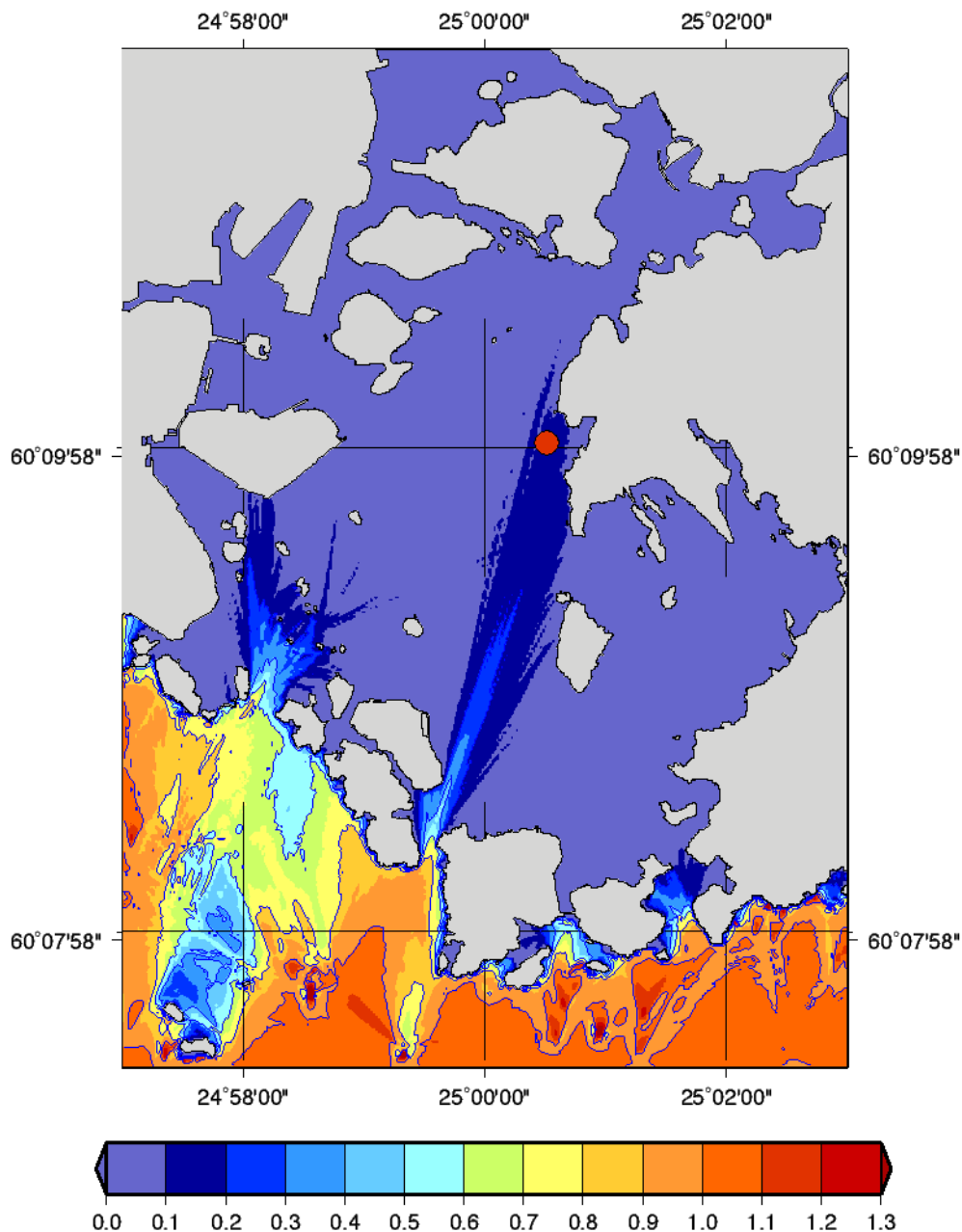
Kuva 62. Avomerén aallokon vaimeneminen Kruunuvuorenrantaan. Merkitsevä aallonkorkeus Kustaanmiekan edustalla 1 m, periodi 4 s, keskisunta 190 astetta.
