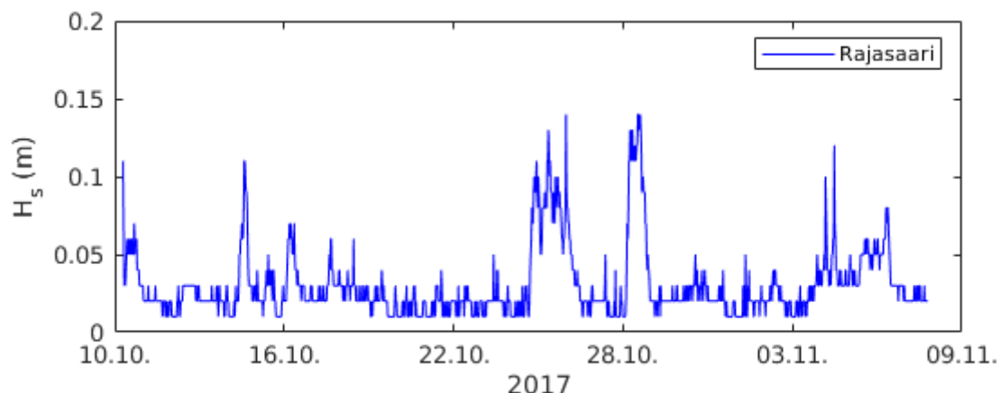
Kuva 125. Merkitsevä aallonkorkeus Rajasaarella koko mittausjakson aikana.
