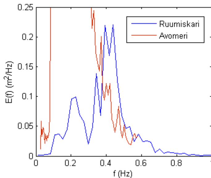
Kuva 32. Lankamittarilla mitattu Ruumiskarin aaltospektri (sininen) ja pojilla mitattu avomerien aaltospektri (punainen). Kuvasta näkyy, että noin 0.4 Hz aallot ovat heijastuneita, joskaan ei aivan täydellisesti. Merkitsevä aallonkorkeus Ruumiskarilla oli 0.84 m ja avomerellä 3.07 m suunnasta 251°.
