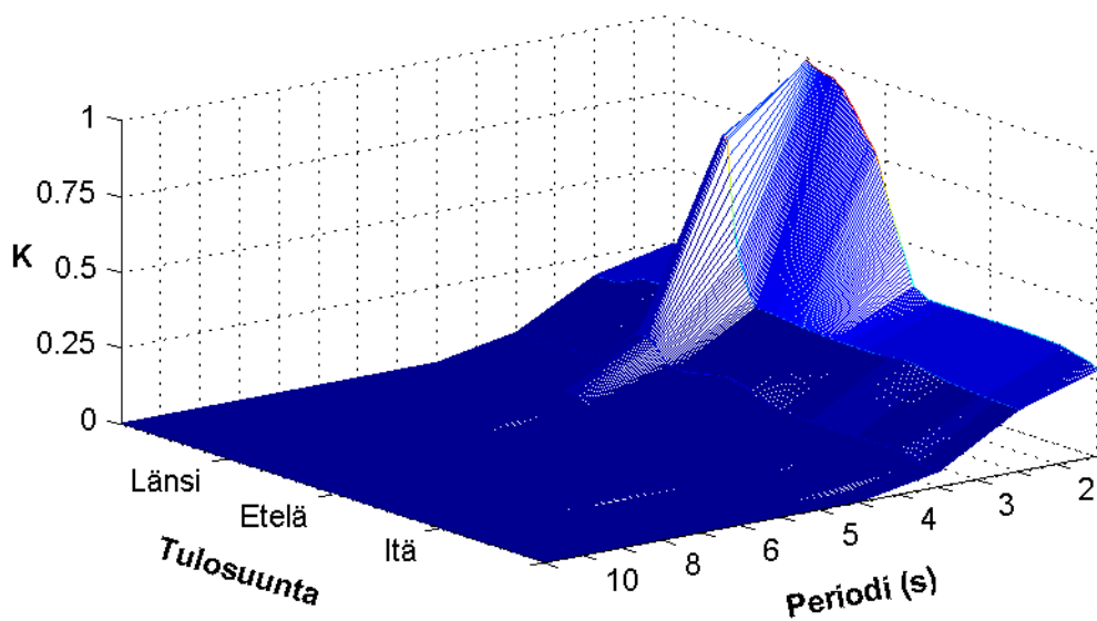
Kuva 66. Likimääräinen siirtofunktion amplitudivaste Kruunuvuorenrannalla kun lähtöaallokko on mitattu Helsingin edustalla.
