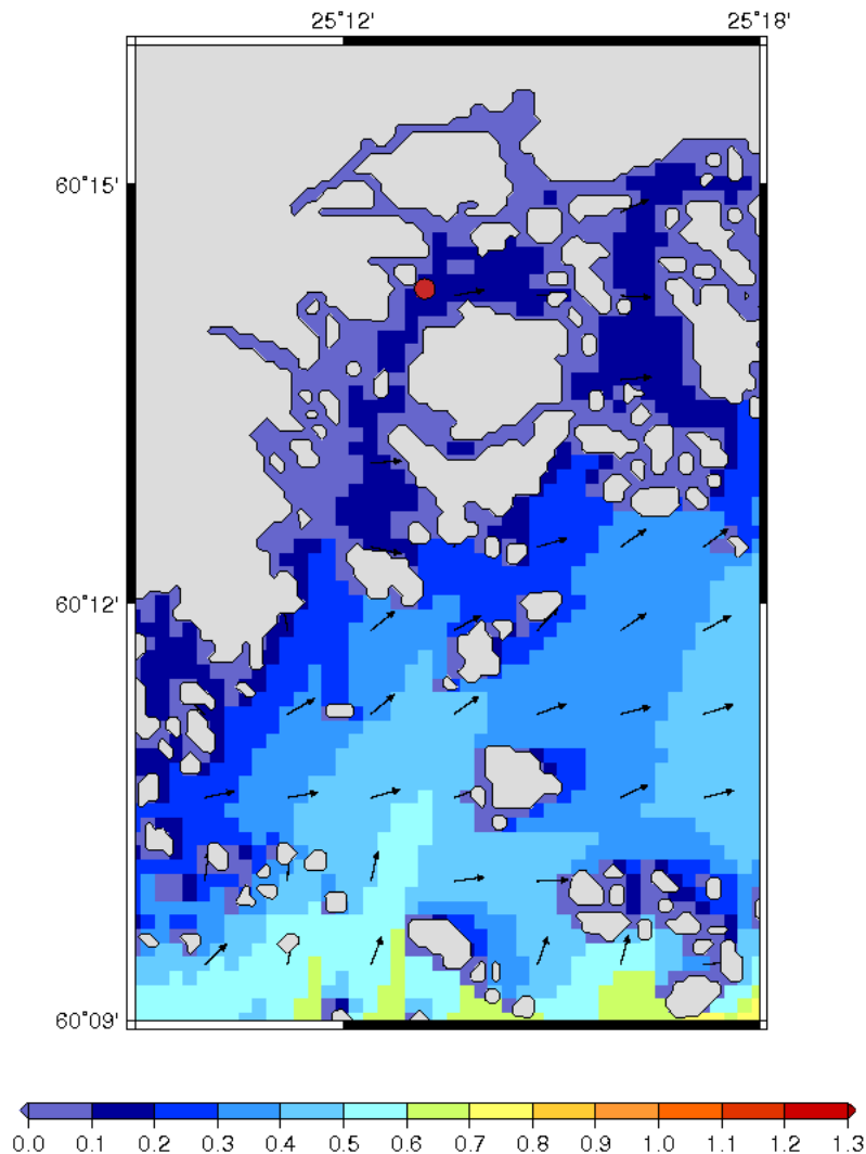
Kuva 92. Avomeren aallokon vaimeneminen Talosaarella. WAM-ajo ajalta 3.9.2012 kello 16:30, jolloin Helsingin pojulla mitattiin merkitsevä aallonkorkeus 1.73 \text{ m} suunnasta 243^{\circ} , hallitsevan periodin ollessa 5.7 \text{ s} .
