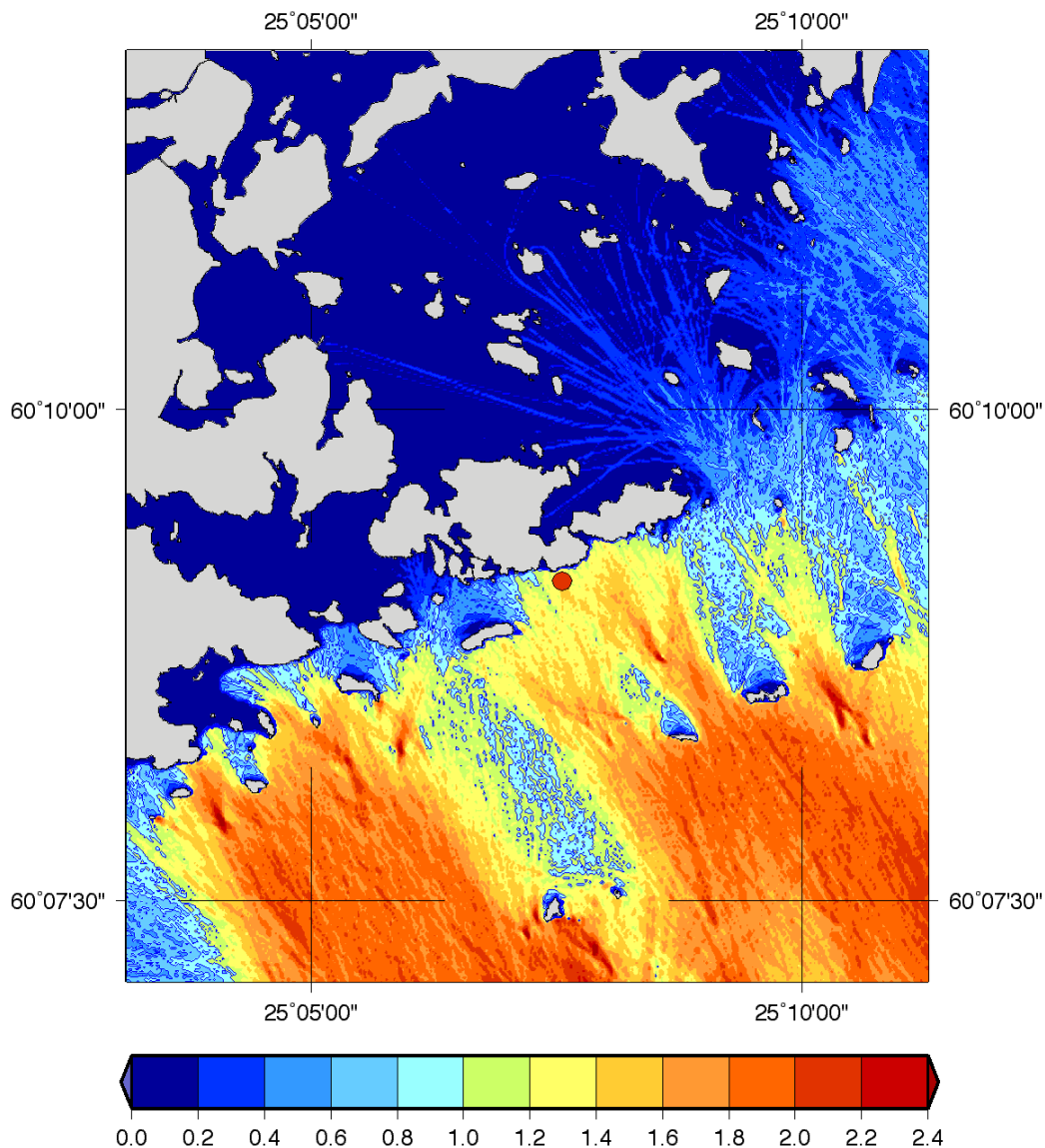
Kuva 96. Avomeren aallokon vaimeneminen Itä-Villingillä. Merkitsevä aallonkorkeus avomerellä 2 m, periodi 5 s, keskisunta 150 astetta.
