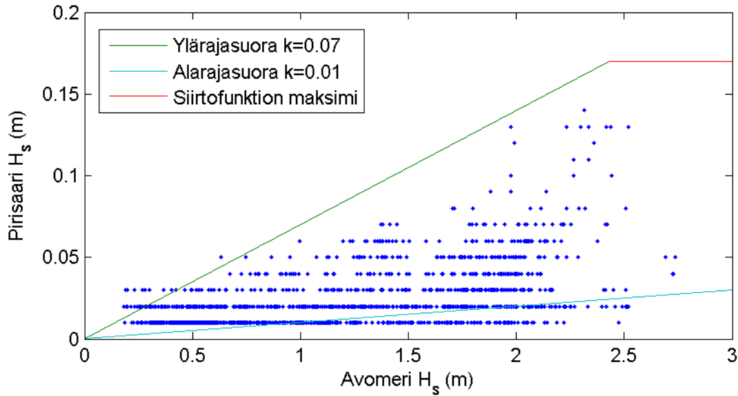
Kuva 11. Merkitsevä aallonkorkeus Pirsaassa ja avomerellä Helsingin edustalla koko mittausjakson aikana. Ylä- ja alarajasuorat vastaavat avomeren aallokon vaimenemista eri vaimenemiskertoimilla k .
