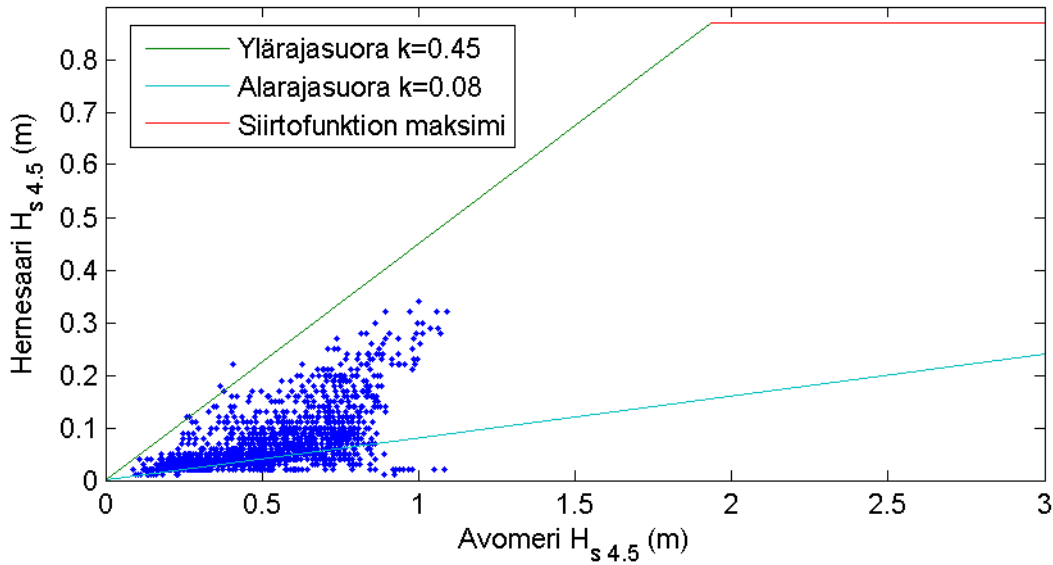
Kuva 40. Merkitsevä aallonkorkeus periodivälillä 4–5 s Hernesaaressa ja avomerellä Helsingin edustalla. Tällä periodivälillä avomeren aallot pääsevät usein Hernesaareen varsin korkeina.
