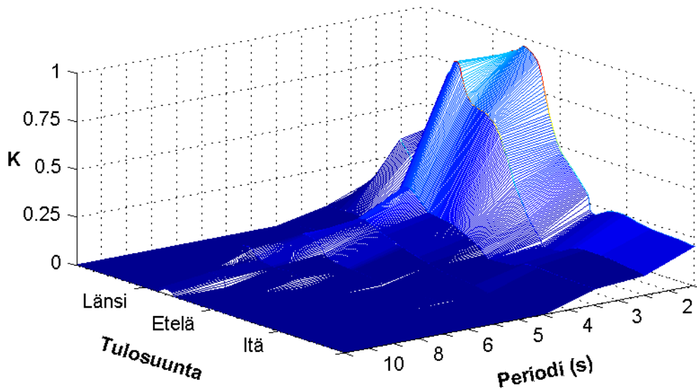
Kuva 61. Likimääräinen siirtofunktion amplitudivaste Koirasaareessa kun lähtöaallokko on mitattu Helsingin edustalla.
