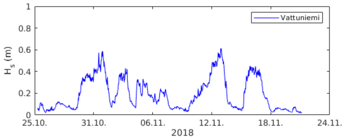
Kuva 119. Merkitsevä aallonkorkeus Vattuniemessä koko mittausjakson aikana.
