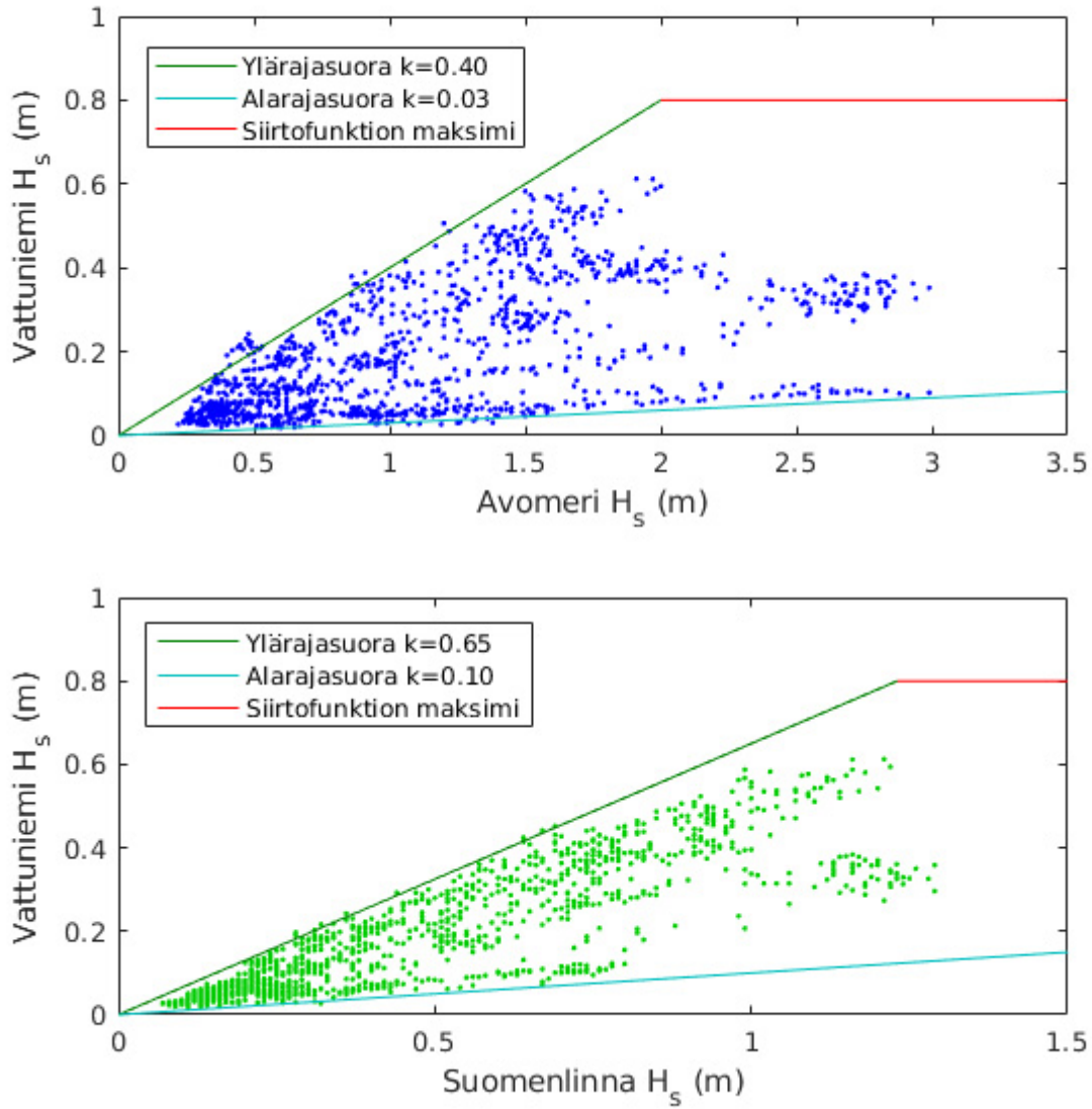
Kuva 122. Merkitsevä aallonkorkeus Vattuniemessä ja avomerellä Helsingin edustalla (yllä) sekä Suomenlinnan edustalla (alla) koko mittausjakson aikana. Ylä- ja alarajasuorat vastaavan ulompana olevien pisteiden vaimenemista eri vaimennuskertoimilla k .
