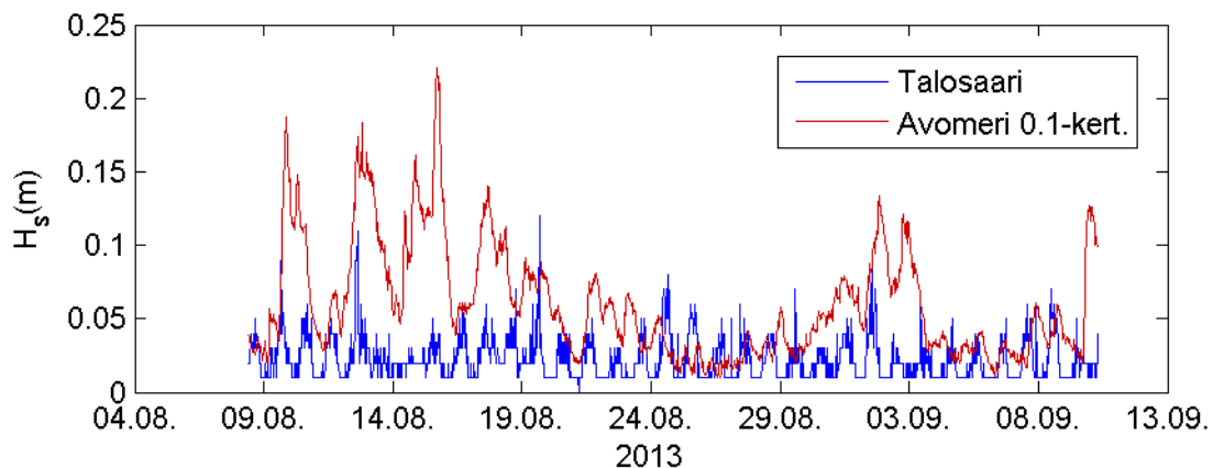
Kuva 94. Merkitsevä aallonkorkeus Talosaassa ja avomerellä Helsingin edustalla (0.1-kertaisena).
