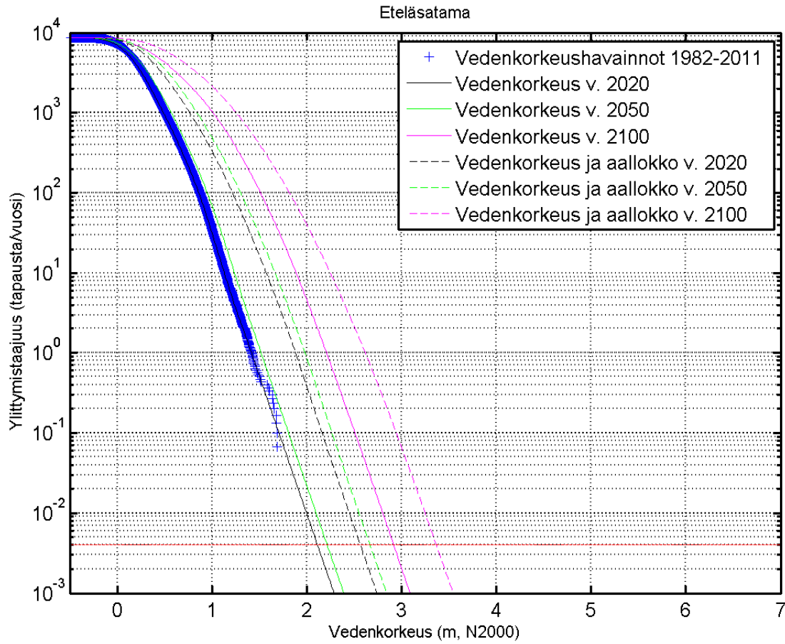
Kuva 131. Tuntihavaintoihin pohjautuva vedenkorkeuden ja aallonkorkeuden yhteisvaikutuksen arvioiminen Eteläsatamaan vuosille 2020, 2050 ja 2100. Pelkkä vedenkorkeusarvo on yksikössä tuntihavaintoja vuodessa, mutta kun tähän arvoon lisätään aallokko, on lopputulos tapausta vuodessa. Punainen vaakaviiva on tässä raportissa käytetty todennäköisyystaso 1/250 tapausta vuodessa.
