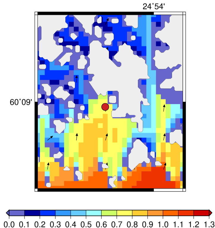
Kuva 118. Avomeren aallokon vaimeneminen Vattuniemessä. WAM-ajo ajalta 18.11.2012 kello 22:30, jolloin Helsingin pojulla mitattiin merkitsevä aallonkorkeus 1.95 m suunnasta 209°, hallitsevan periodin ollessa 5.0 s.
