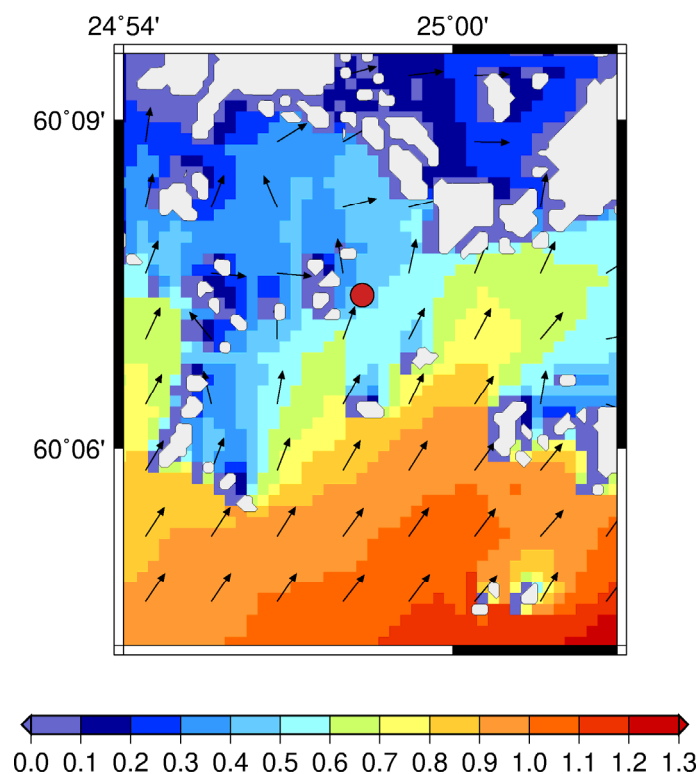
Kuva 111. Avomeren aallokon vaimeneminen Suomenlinnan edustalla. WAM-ajo ajalta 03.09.2012 kello 16:30, jolloin Helsingin poijualla mitattiin merkitsevä aallonkorkeus 1.73 m suunnasta 243°, hallitsevan periodin ollessa 5.6 s.
