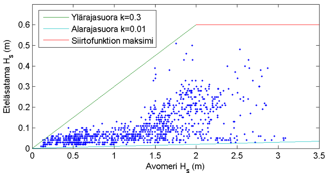
Kuva 78. Merkitsevä aallonkorkeus Eteläsatamassa ja avomerellä Helsingin edustalla koko mittausjakson aikana. Ylä- ja alarajasuorat vastaavat avomeri aallokon vaimenemista eri vaimenemiskertoimilla k .
