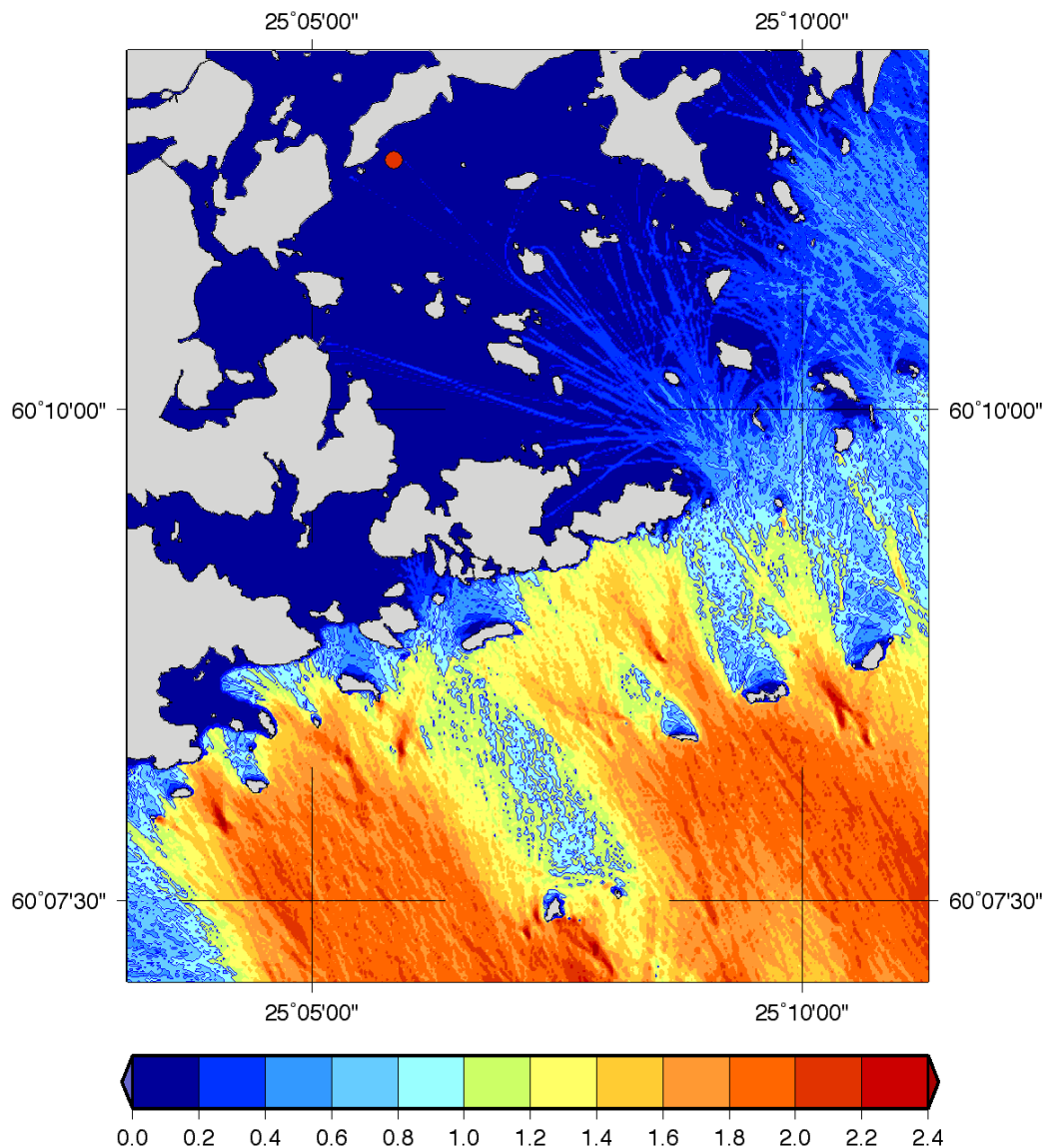
Kuva 79. Avomerén aallokon vaimeneminen Ramsinniemessä. Merkitsevä aallonkorkeus avomerellä 2 m, periodi 5 s, keskisuunta 150 astetta.
