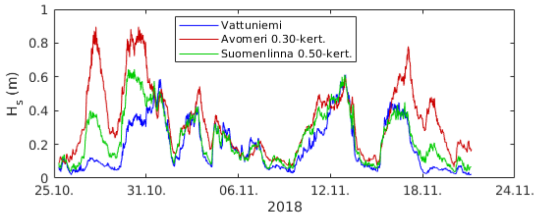
Kuva 121. Merkitsevä aallonkorkeus Vattuniemen poijulla, Suomenlinnan poijulla (0.5-kertaisena) ja Helsingin avomeren poijulla (0.3-kertaisena).
