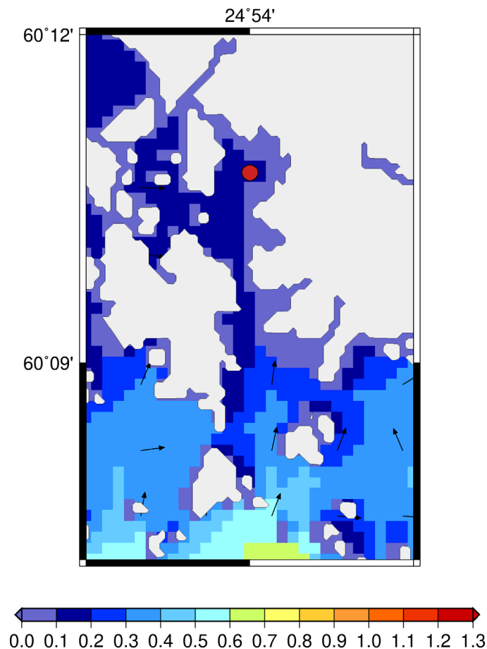
Kuva 124. Avomerien aallokon vaimeneminen Seurasaarenselällä. WAM-ajo ajalta 03.09.2012 kello 14:30, jolloin Helsingin poijulla mitattiin merkitsevä aallonkorkeus 1.73 m suunnasta 243^{\circ} , hallitsevan periodin ollessa 5.6 s.
