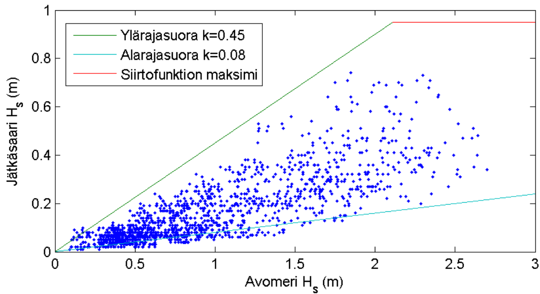
Kuva 22. Merkitsevä aallonkorkeus Jätkäsaarella ja avomerellä Helsingin edustalla. Ylä- ja alarajasuorat vastaavat avomerén aallokon vaimenemista eri vaimenemiskertoimilla k .
