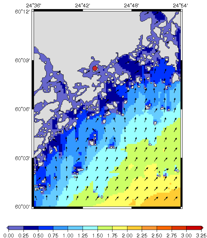
Kuva 8. Aallokko Pirisaarella on hyvin suojattu avomeren aallokolta. WAM-ajo ajalta 7.10.2012 kello 13:00, jolloin avomerellä mitattiin 2.49 m merkitsevä aallonkorkeus suunnasta 247^{\circ} , hallitsevan periodin ollessa 7.1 s.
