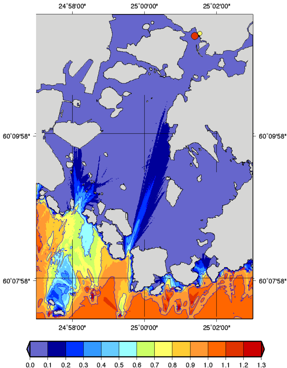
Kuva 67. Avomeren aallokon vaimeneminen Kipparlahdella. Merkitsevä aallonkorkeus Kustaanmiekkan edustalla 1 m, periodi 4 s, keskisuinta 190^{\circ} astetta. Punainen ympyrä näyttää poijun sijainnin ja keltainen ympyrä näyttää paikan mistä mittauksia tehtiin kapasitiivisella langalla rannasta.
