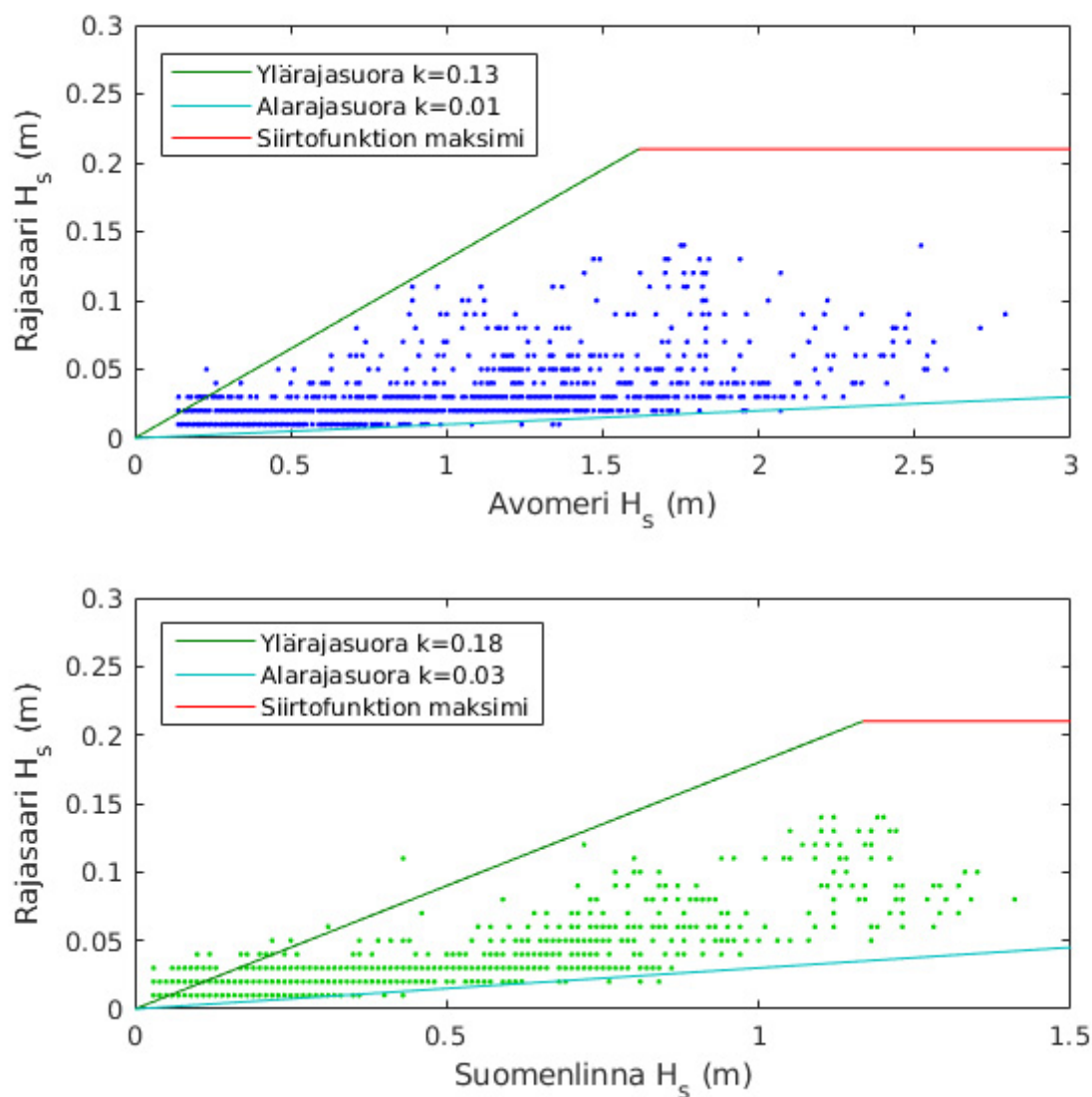
Kuva 128. Merkitsevä aallonkorkeus Rajasaarella ja avomerellä Helsingin edustalla (yllä) sekä Suomenlinnan edustalla (alla) koko mittausjakson aikana. Ylä- ja alarajasuorat vastaavat ulompänä olevien pisteiden aallokon vaimenemista eri vaimenemiskertoimilla k .
