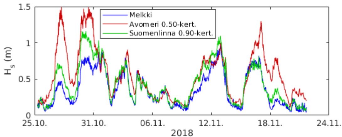
Kuva 115. Merkitsevä aallonkorkeus Melkin pojilla, Suomenlinnan pojilla (0.9-kertaisena) ja Helsingin avomeren pojilla (0.5-kertaisena).
