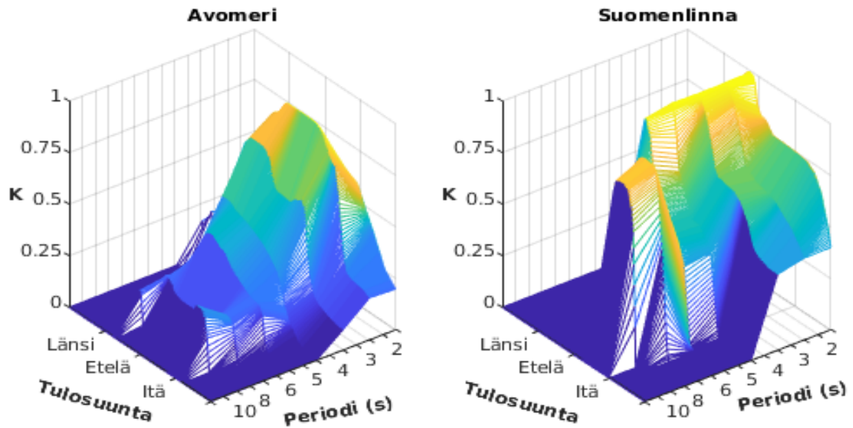
Kuva 117. Likimääräinen siirtofunktion amplitudivaste Melkissä kun lähtöaallokko on mitattu Helsingin edustalla (vasen) tai Suomenlinnan edustalla (oikea).
