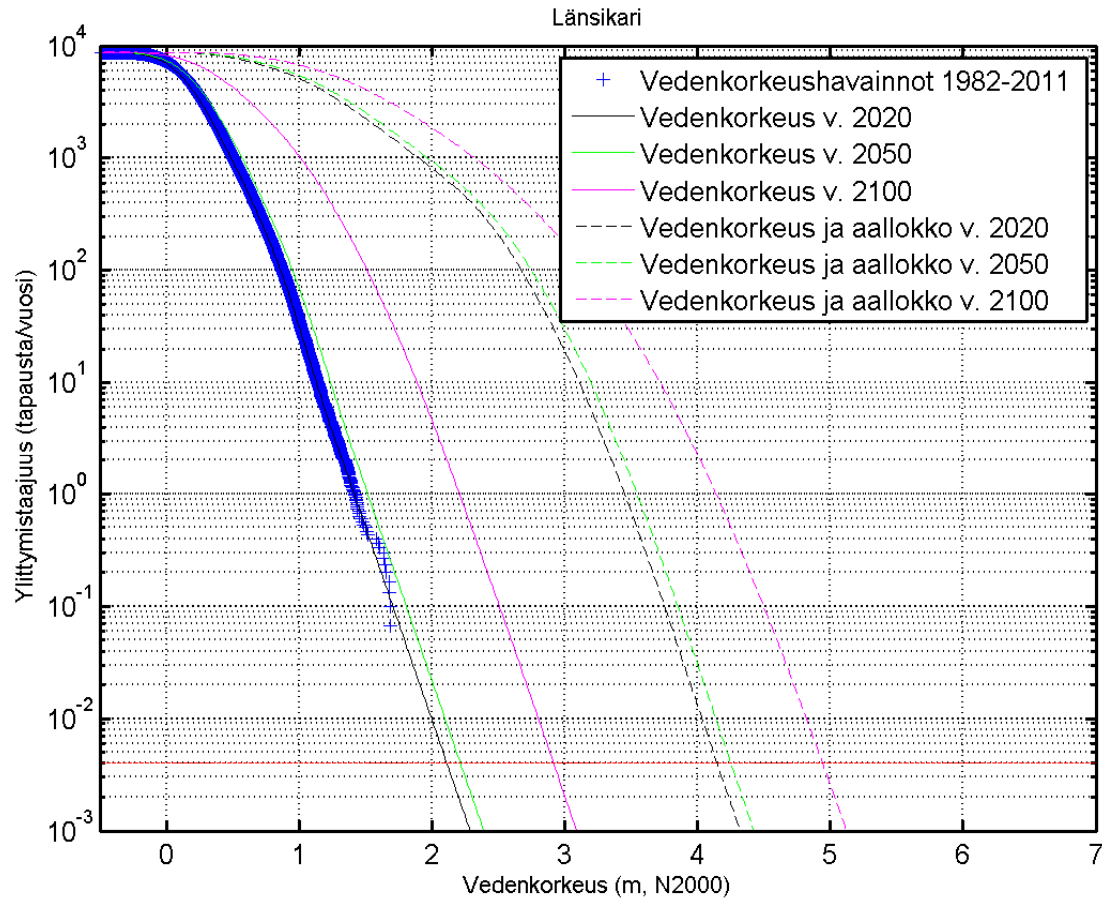
Kuva 132. Tuntihavaintoihin pohjautuva vedenkorkeuden ja aallonkorkeuden yhteisvaikutuksen arvioiminen Länsikarille vuosille 2020, 2050 ja 2100. Pelkkä vedenkorkeusarvo on yksikössä tuntihavaintoja vuodessa, mutta kun tähän arvoon lisätään aallokko, on lopputulos tapausta vuodessa. Punainen vaakaviiva on tässä raportissa käytetty todennäköisyystaso 1/250 tapausta vuodessa.
