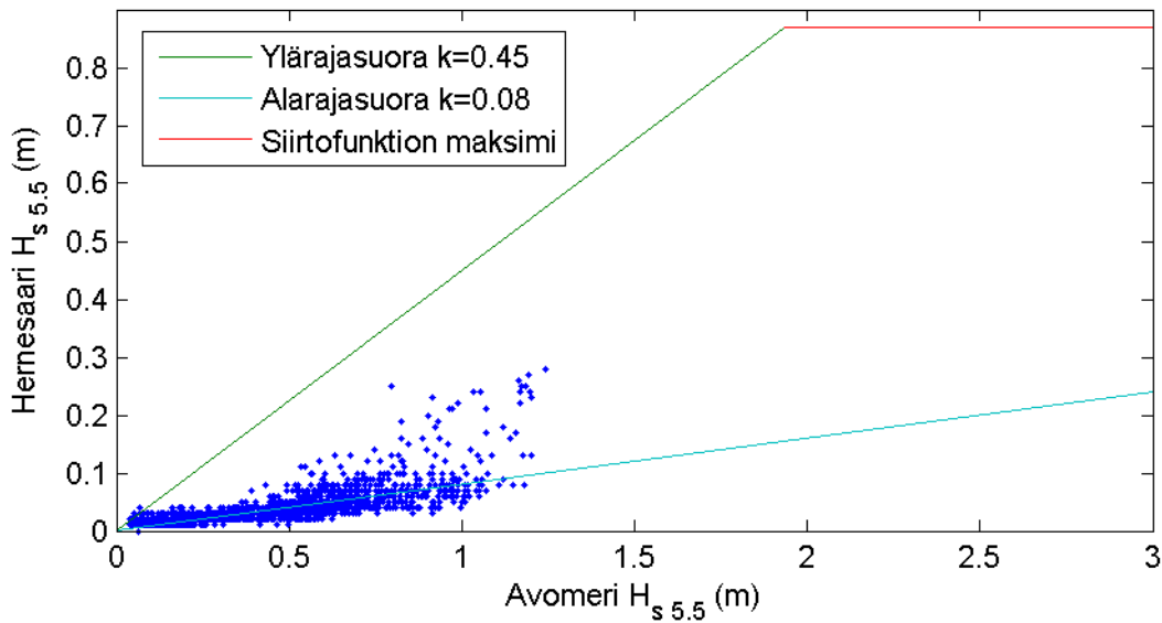
Kuva 41. Merkitsevä aallonkorkeus periodivälillä 5–6 s Hernesaaressa ja avomerellä Helsingin edustalla. Tällä periodivälillä avomeren aallot ovat jo vaimentuneet voimakkaasti.
