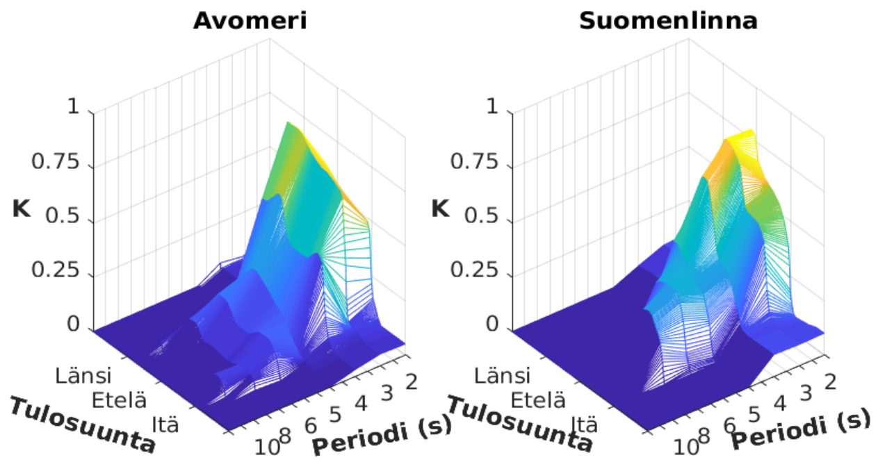
Kuva 123. Likimääräinen siirtofunktion amplitudivaste Vattuniemessä kun lähtöaallokko on mitattu Helsingin edustalla (vasen) tai Suomenlinnan edustalla (oikea).
