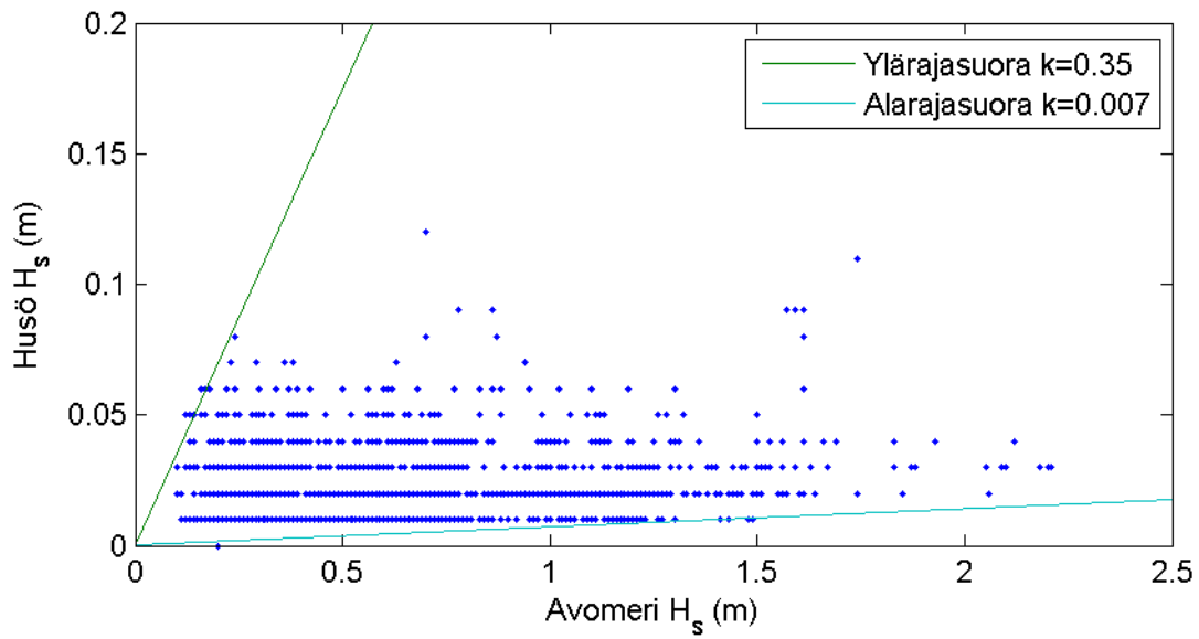
Kuva 95. Merkitsevä aallonkorkeus Talosaaressa ja avomerellä Helsingin edustalla koko mittausjakson aikana. Ylä- ja alarajasuorat vastaavat avomerien aallokon vaimenemista eri vaimenemiskertoimilla k .
