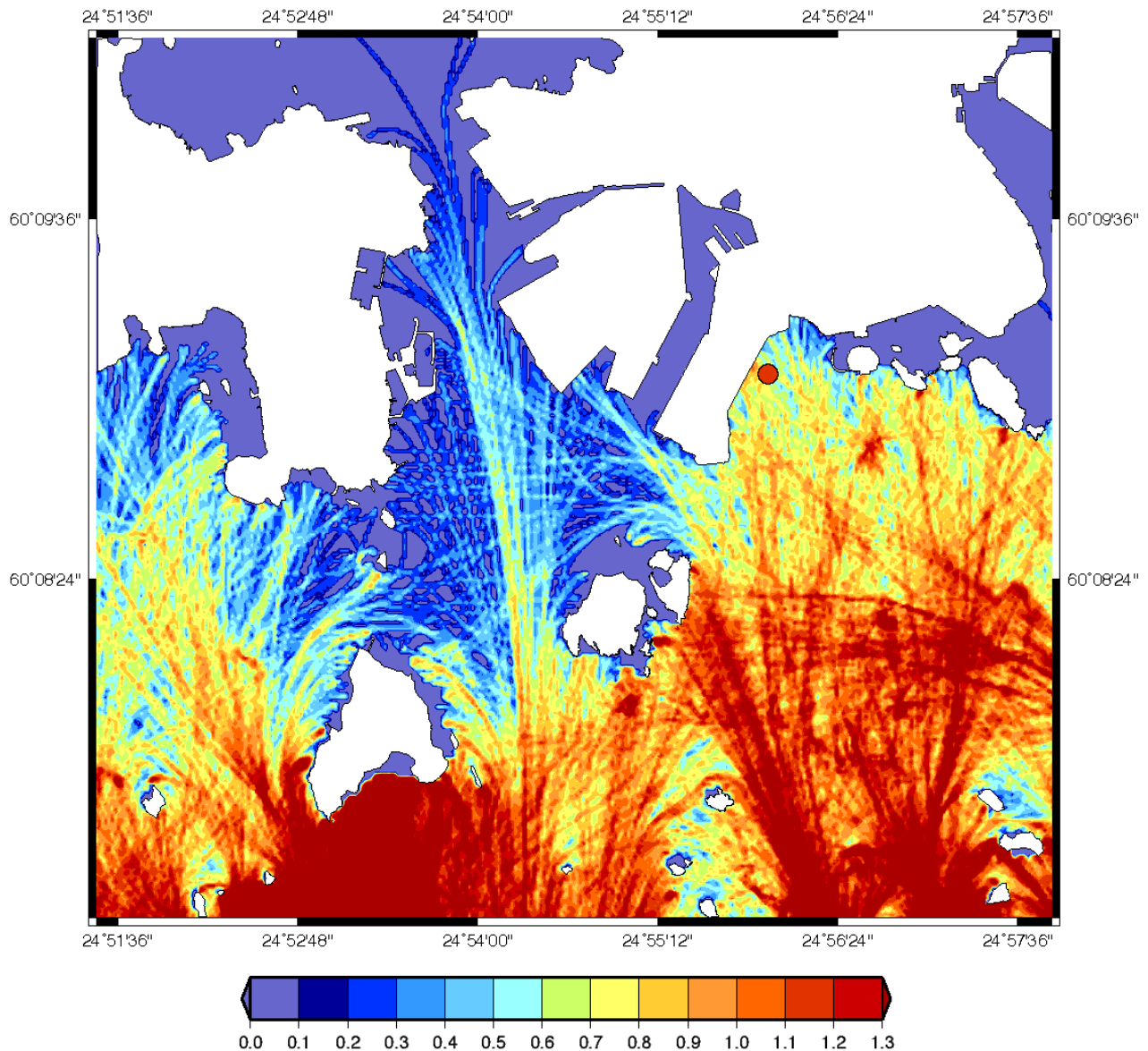
Kuva 35. Hernesaaren mittauspaikka (keltainen mustalla reunustettu ympyrä) sekä refraktiomallilla laskettu avomereltä tullut aallokko, jonka merkittävä aallonkorkeus on 2.91 m, periodi on 6 sekuntia ja tulosuunta avomerellä 180 astetta.
