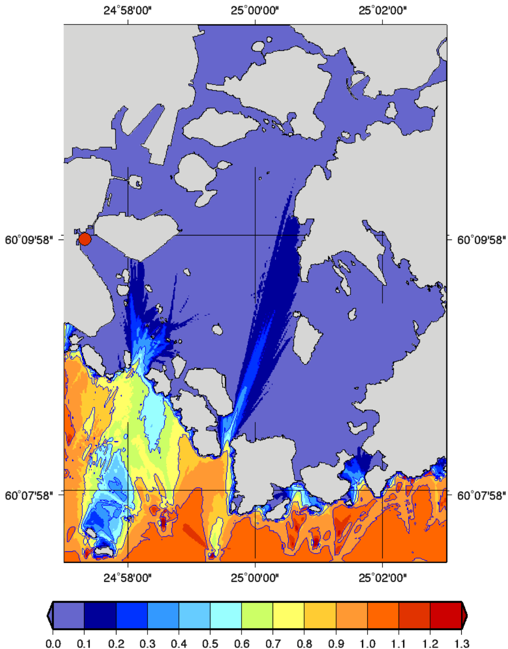
Kuva 74. Avomeren aallokon vaimeneminen Kruunuvuorenselällä. Merkitsevä aallonkorkeus Kustaanmiekan edustalla 1 m, periodi 4 s, keskisuinta 190 astetta. Eteläsataman mittauspiste on merkitty punaisella ympyrällä.
