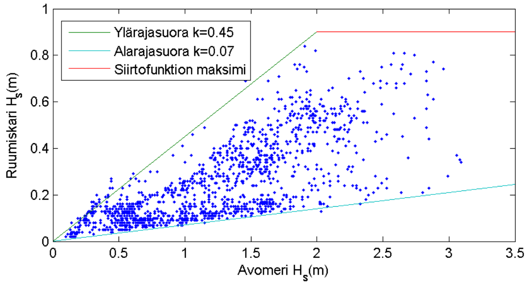
Kuva 33. Merkitsevä aallonkorkeus Ruumiskarilla ja avomerellä Helsingin edustalla koko mittausjakson aikana. Ylä- ja alarajasuorat vastaavat avomerren aallokon vaimenemista eri vaimenemiskertoimilla k .
