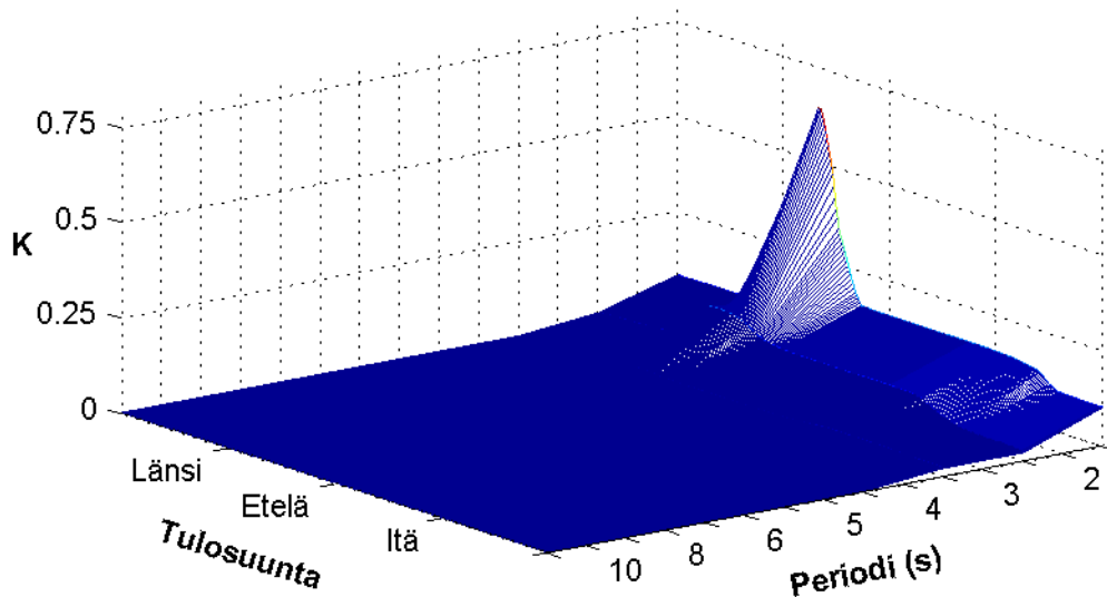
Kuva 12. Likimääräinen siirtofunktion amplitudivaste ( K ) Pirsaassa kun lähtöaallokko on mitattu Helsingin edustalla.
