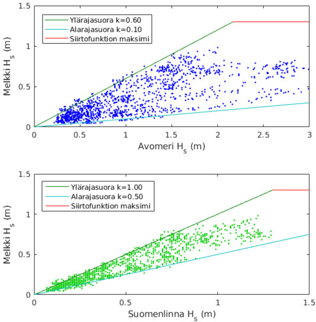
Kuva 116. Merkitsevä aallonkorkeus Melkissä ja avomerellä Helsingin edustalla (yllä) sekä Suomenlinnan edustalla (alla) koko mittausjakson aikana. Ylä- ja alarajasuorat vastaavan ulompana olevien pisteiden vaimenemista eri vaimennuskertoimilla k .
