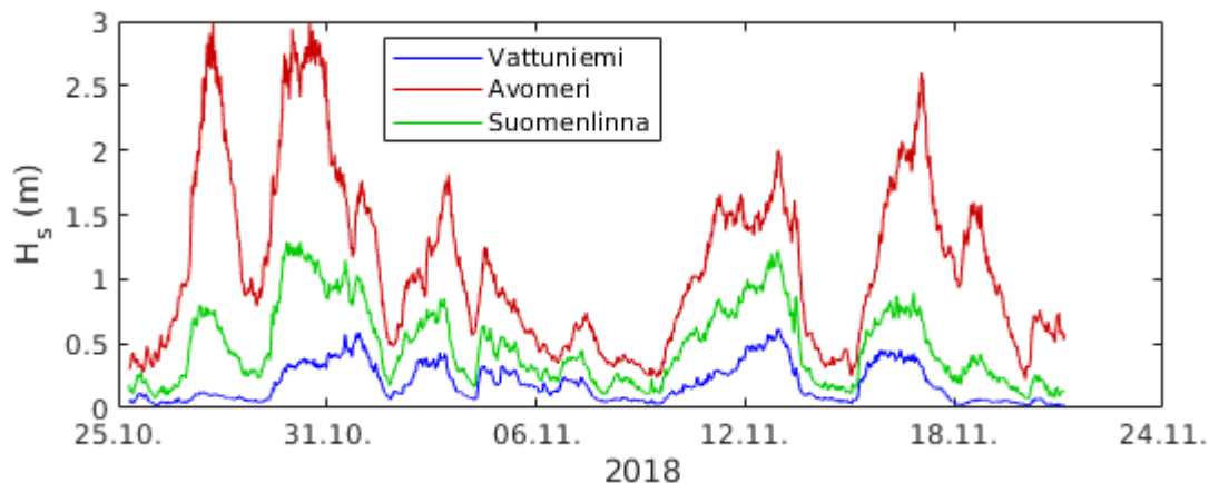
Kuva 120. Merkitsevä aallonkorkeus Vattuniemen poijulla, Suomenlinnan poijulla ja Helsingin avomeren poijulla.
