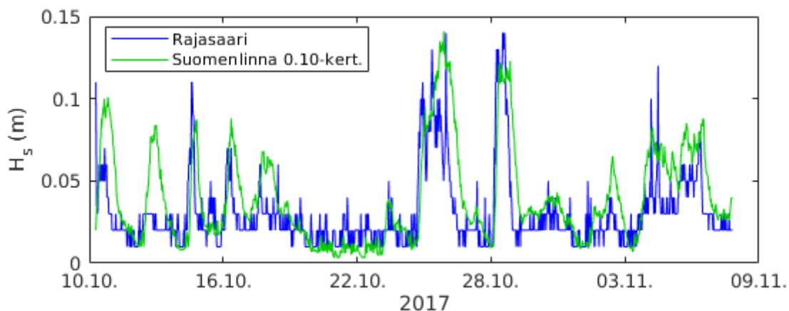
Kuva 127. Merkitsevä aallonkorkeus Rajasaaren poijulla ja Suomenlinnan poijulla (0.1-kertaisena).
