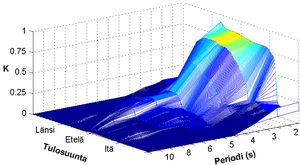
Kuva 26. Likimääräinen siirtofunktion amplitudivaste Jätkäsaarella kun lähtöaallokko on Helsingin edustalla mitattu. Suunta on Helsingin edustalla mitattu aallokon keskusuenta, joka Suomenlahden muodon vuoksi keskittyy suuntiin 240 astetta ja 90 astetta. Jätkäsaareen pääsee kuitenkin aallokkoa merkittävästi myös suunnasta 180 astetta.
