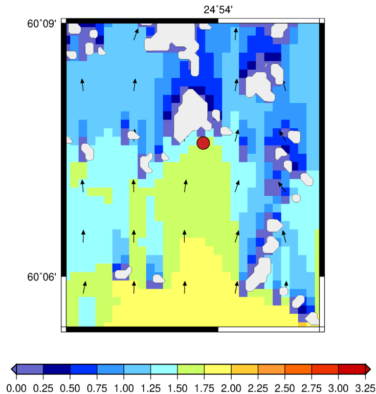
Kuva 112. Avomerén aallokon vaimeneminen Melkin edustalla. WAM-ajo ajalta 30.10.2012 kello 00:30, jolloin Helsingin pojulla mitattiin merkitsevä aallonkorkeus 1.98 m suunnasta 195°, hallitsevan periodin ollessa 5.2 s.
