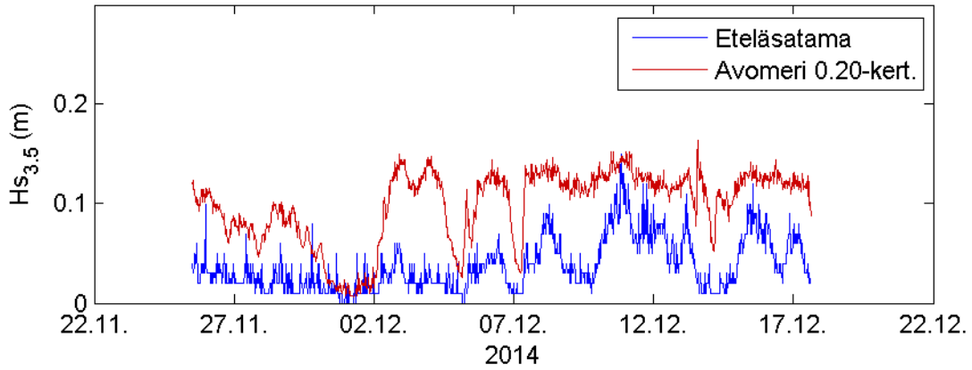
Kuva 77. Merkitsevä aallonkorkeus periodivälillä 3–4 s on mittausjakson aikana Eteläsatamassa poijulla enintään 0.2-kertainen avomeri aallokkoon verrattuna.
