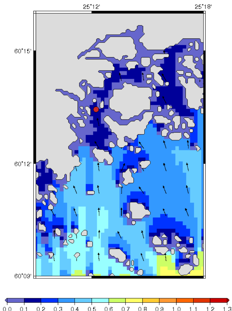
Kuva 88. Avomeren aallokon vaimeneminen Vuosaaren satamassa. WAM-ajo ajalta 4.10.2012 kello 23:30, jolloin Helsingin pojilla mitattiin merkitsevä aallonkorkeus 0.90 m suunnasta 180^{\circ} , hallitsevan periodin ollessa 4.0 s.
