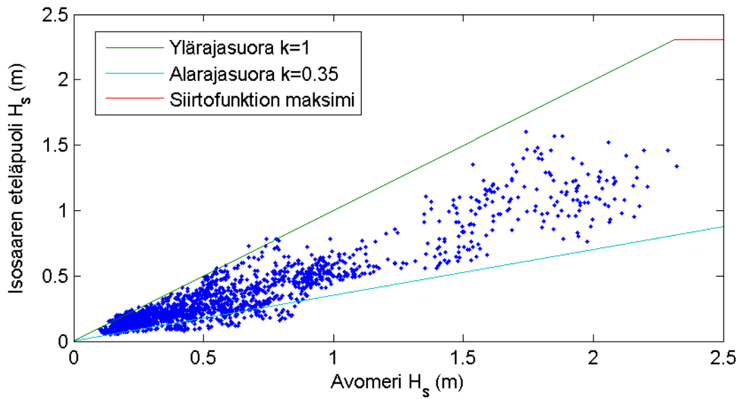
Kuva 104. Merkitsevä aallonkorkeus Isosaaren eteläpuolella ja avomerellä Helsingin edustalla koko mittausjakson aikana. Ylä- ja alarajasuorat vastaavat avomerén aallokon vaimenemista eri vaimenemiskertoimilla k .
