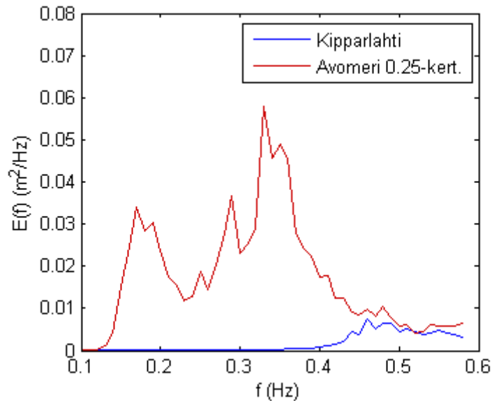
Kuva 70. 28.10.2013 kello 08:00 mitatut aaltospektrit mistä näkyvät Kipparlahden paikallinen aallokko (sininen) ja Helsingin poijulla mitattu aaltospektri 0.25-kertaisena (punainen). Merkitsevä aallonkorkeus oli Kipparlahdella 0.11 m ja Helsingin poijulla 0.74 m.
