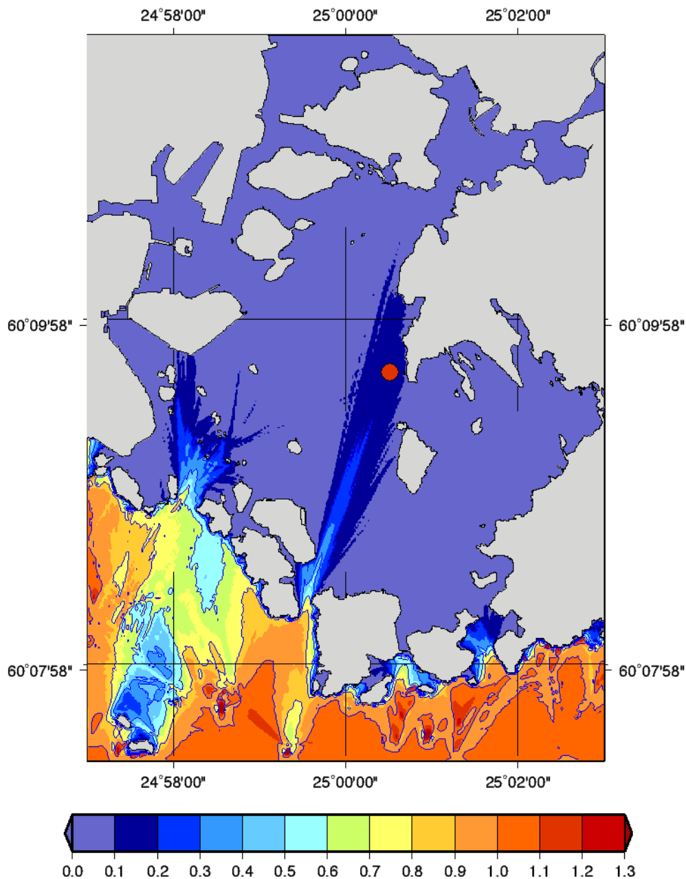
Kuva 56. Avomeren aallokon vaimeneminen Koirasaarella. Merkitsevä aallonkorkeus Kustaanmiekan edustalla 1 m, periodi 4 s, keskisuuunta 190 astetta.
