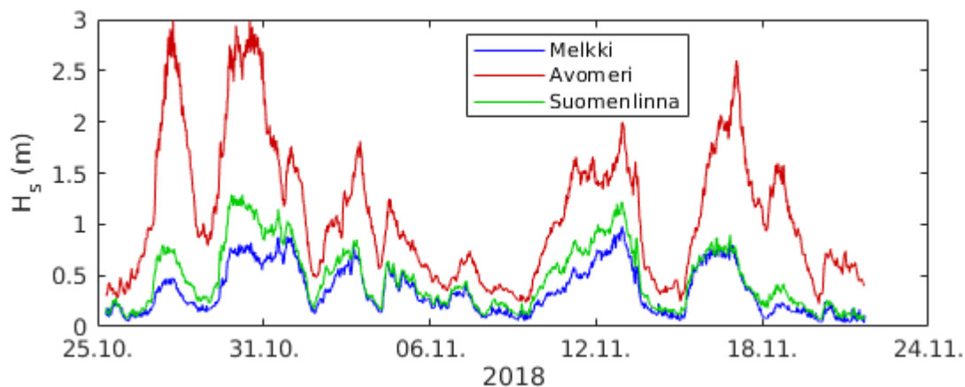
Kuva 114. Merkitsevä aallonkorkeus Melkin poijulla, Suomenlinnan poijulla ja Helsingin avomeren poijulla.
