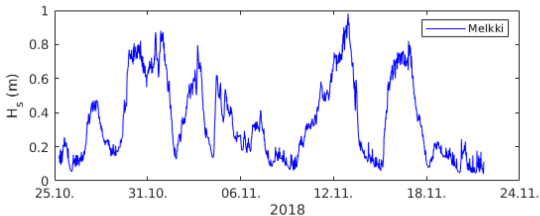
Kuva 113. Merkitsevä aallonkorkeus Melkin poijulla koko mittausjakson ajan.
