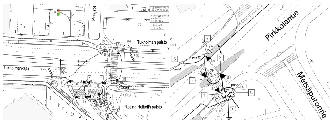
Kuva 18 Pihlajatie suuntaan ei ole valo-ohjausta. Valo-ohjaus on vain suojatie kohdalla.
