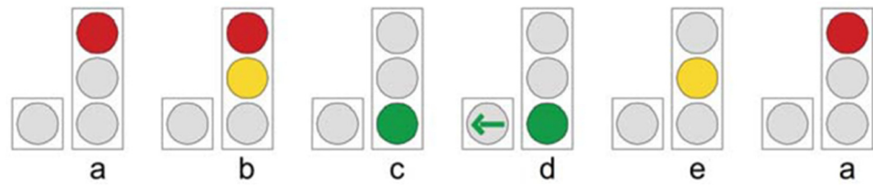
Kuva 6 Yksiaukkoisella lisäopastimella voidaan esimerkiksi vasemmalle kääntyvälle auto- liikenteelle antaa niin kutsuttu jälkivihreä (kohta d). (Liikennevirasto 2016)
