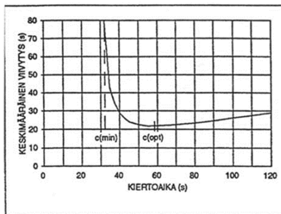
Kuva 8 Kiertoaajan vaikutus risteysen viivytyksiin. (Liikennevirasto 2016)
