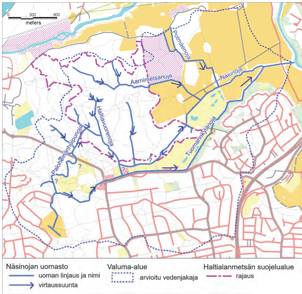
Kuva 23 Näsinöja haarautuu useaksi ojaksi tai puroksi 7 km 2 valuma-alueellaan.
