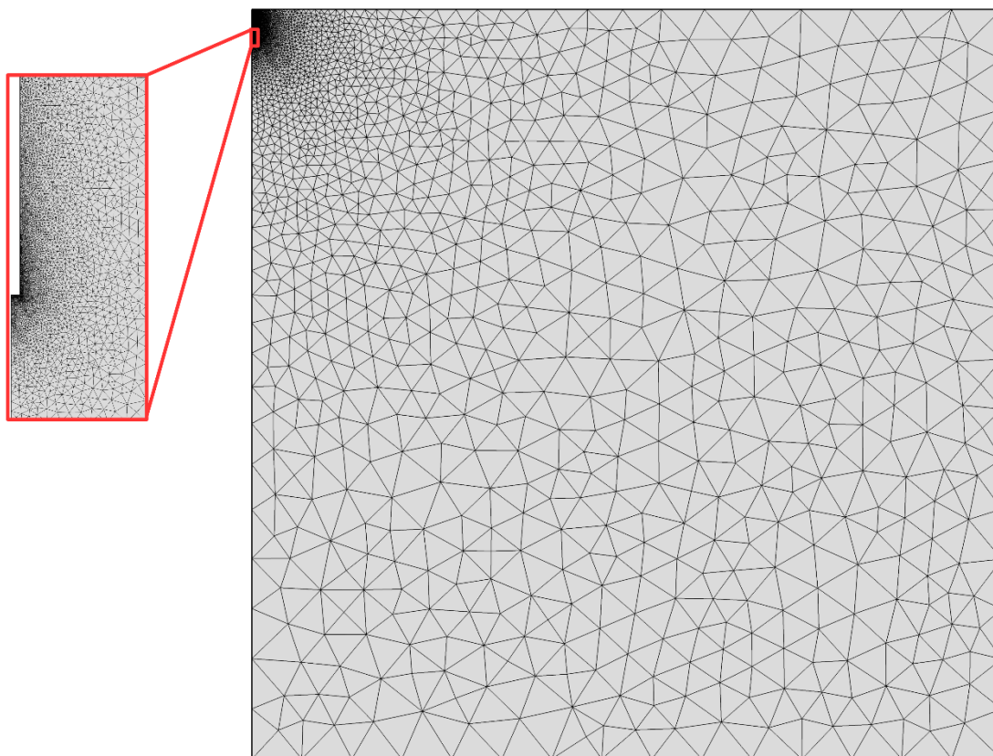
Kuva 100. Esimerkki aksiaalisymmetrisestä elementtimallista. Kuvassa on esitetty 150 metriä syvää lämpökaivoa kuvaava malli ja sen elementtiverkosto. Lähikuvassa on esitetty tarkemmin lämpökaivoa mallintava reuna.
