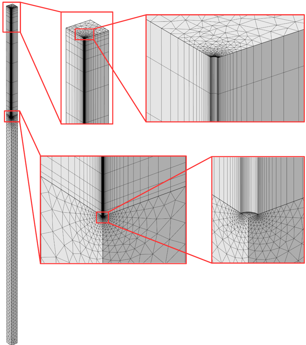
Kuva 94. Esimerkki elementtimallista. Kuvassa on esitetty 150 metriä syvää lämpökaivoa kuvaava malli ja sen elementtiverkosto. Lähikuvissa on esitetty mallin yksityiskohdat tarkemmin.
