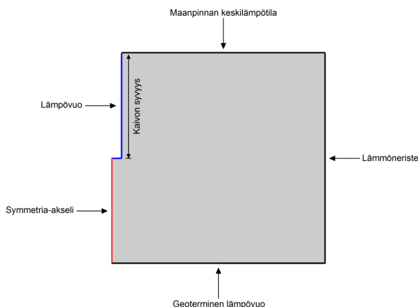
Kuva 99. Yksittäisen lämpökaivon mallin geometria. Malli on kaksikulotteinen ja aksiaalisymmetrinen.
