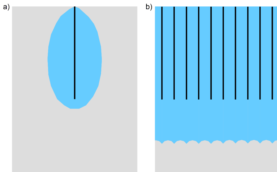
Kuva 103. Lämmönoton laajuus yksittäisen lämpökaivon ja lämpökaivokentän tapauksessa. Kuva esittää esimerkinomaisesti sitä, miten laajalta alueelta (a) yksittäinen lämpökaivo ja (b) suuri lämpökaivokenttä ottavat lämpöä. Mustat viivat esittävät lämpökaivoja. Sininen väri esittää sitä osaa kalliosta, josta lämpöä on otettu ja jonka lämpötila on siitä syystä laskenut. Harmaa väri esittää sitä osaa kalliosta, josta lämpöä ei ole saatu otettua eikä lämpötila sen takia ole laskenut.
