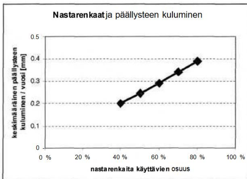
Kuva 1. Päällysteen kulumisen riippuvuus nastarenkaita käyttävien osuudesta testiliikennemäärillä (Arrojo 2000)
