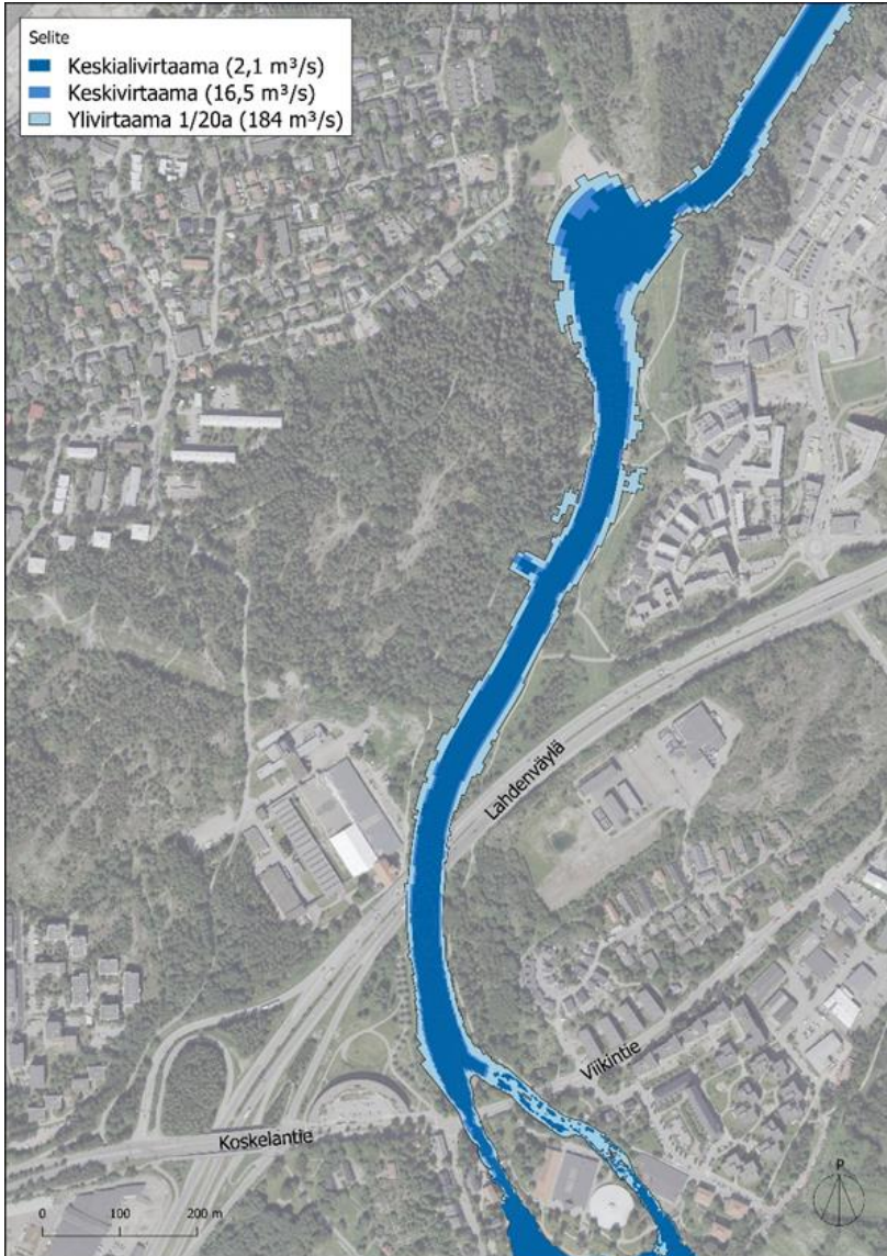
Kuva 27 Simuloidut vedenkorkeudet skenaariossa 2 Vanhankaupunginkosken Pikkukosken uimarannan välillä (keskiali-, keski- ja ylivirtaama).
