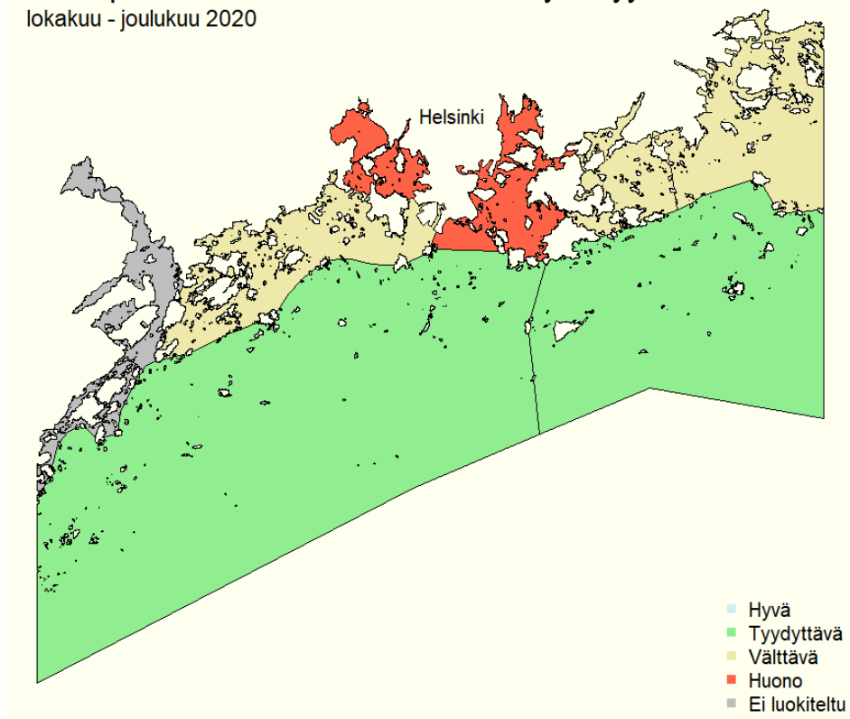
Kuva 16. TRIX-trofiaiindeksin avulla luokiteltu pääkaupunkiseudun merialueen rehevöityneisyyden tila.
