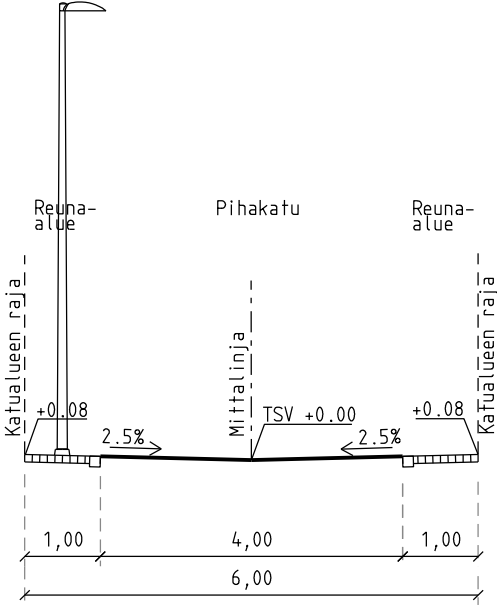
Tyyppipoikkileikkaus pl 60
