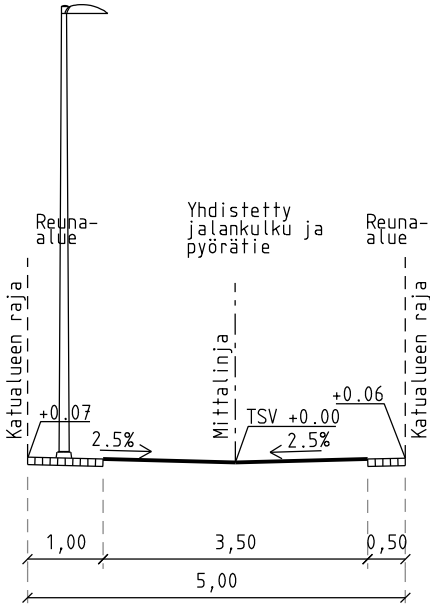
Tyyppipoikkileikkaus pl 20
