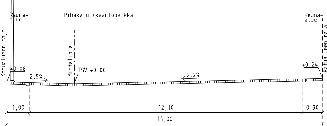
Tyyppipoikkileikkaus pl 40
