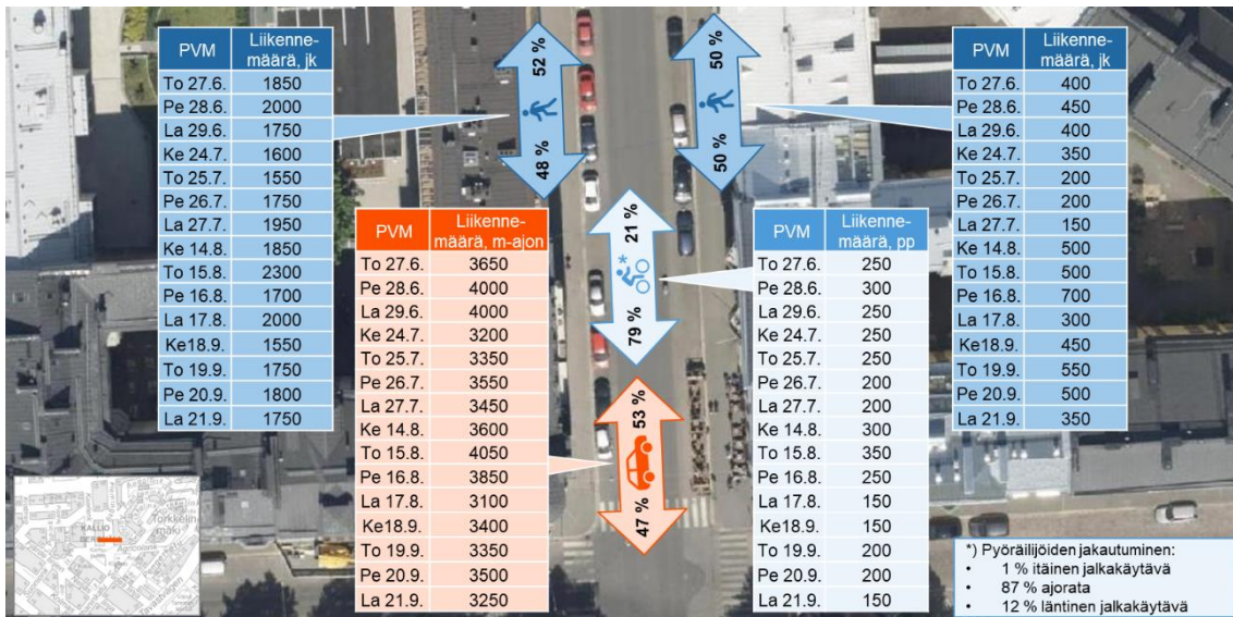
Kuva 12. Fleminginkatu – Agricolankatu liikenteen poikkileikkaustulokset.
