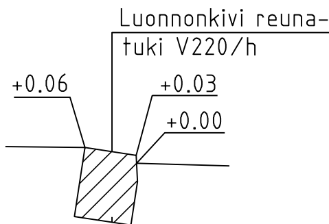
Leikkaus A-A 1:25
