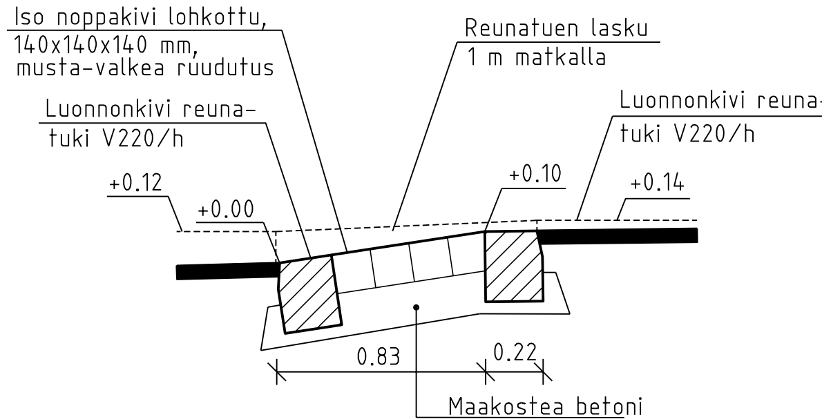
Leikkaus B-B 1:25
