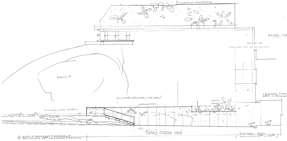
Martta ja Ragnar Ypyän sairaalasuunnitelmaan on liittynyt myös pihasuunnitelma, muun muassa muureihin liittyviä pihadetaljeja on mietitty huolellisesti. Pihamaan järjestely 1961. SRM
