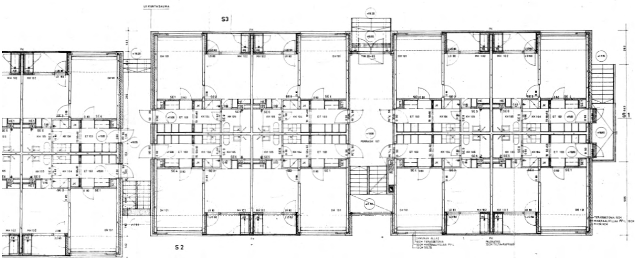
Kuva 3. Ote Medioma II:n ensimmäisen kerroksen pohjakaaviosta. Ensimmäisessä kerroksessa on kaksioita, toisessa ja kolmannessa kerroksessa on keskikäytävän varrelle sijoittuvia yksioitä.
