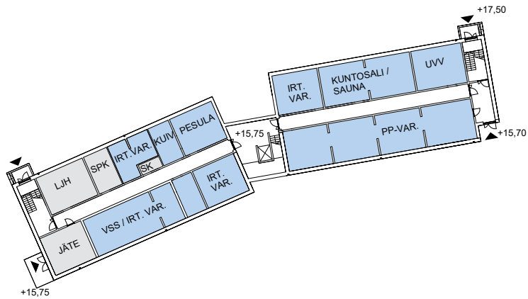
Rak 1 kellaritaso taso +15,75
