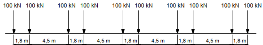
Kuva 6. Raitiotien väsytySKUORMAKAAVIO FLMT.
