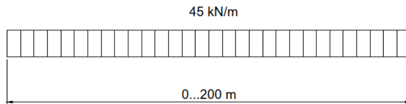
Kuva 4. Raitiotiekuormakaavio LMT.
