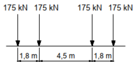
Kuva 5. Raitiotiekuormakaavio LMT-L.
