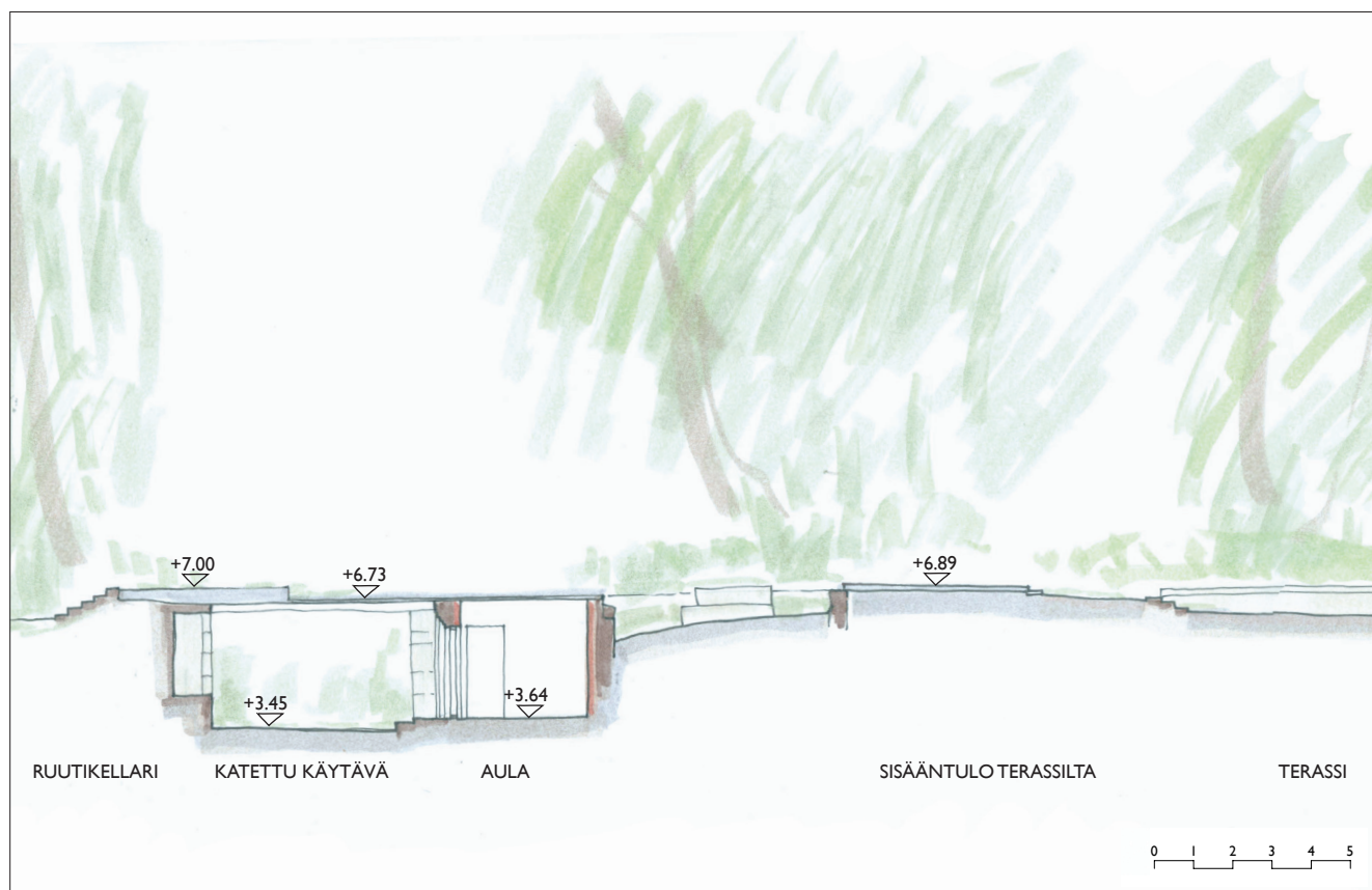
Kuva 9. Nykytilanne, alataso, leikkaus A-A.
