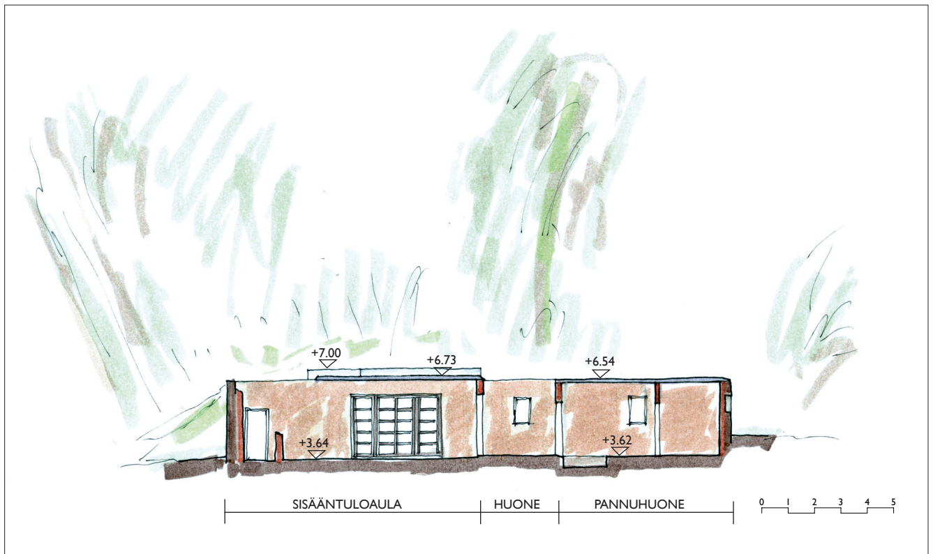
Kuva 13. Nykytilanne, ylätaso, leikkaus B-B
