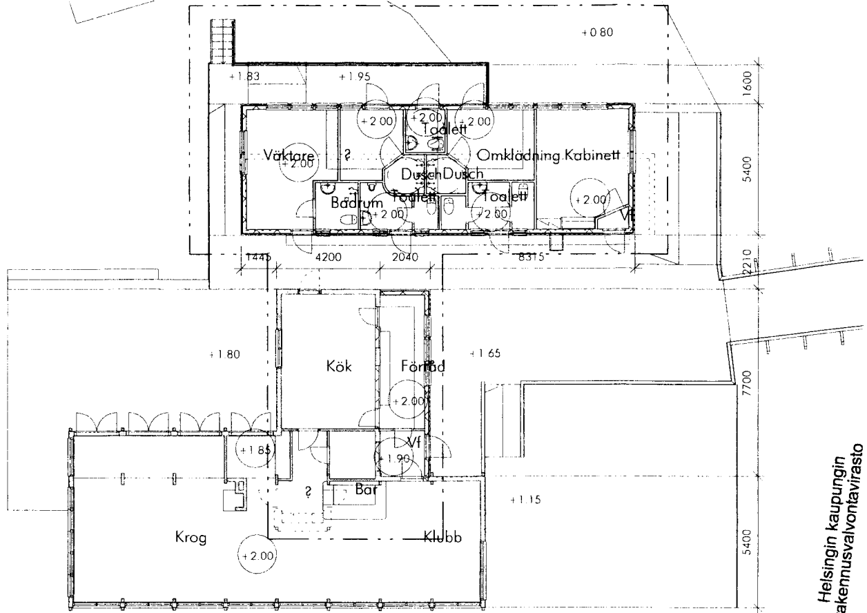
■ 2 - plan 1 : 200
