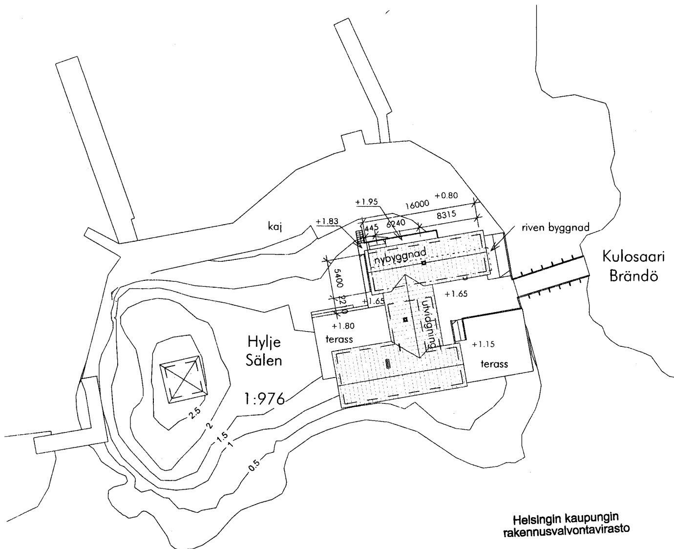
■ 1 - situationsplan 1 : 500
