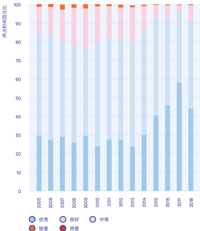
赫尔辛基市中心空气质量
