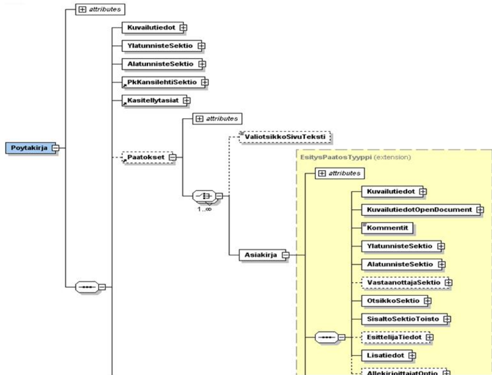
Kuva 12: OpenAhjon pöytäkirjan rakennekuvaotos
