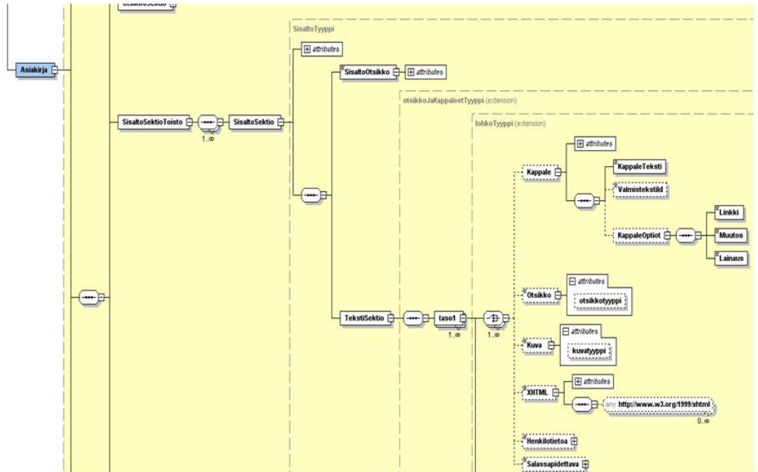
Kuva 13: OpenAhjon yleinen asiakirjan rakennekuvaotos
