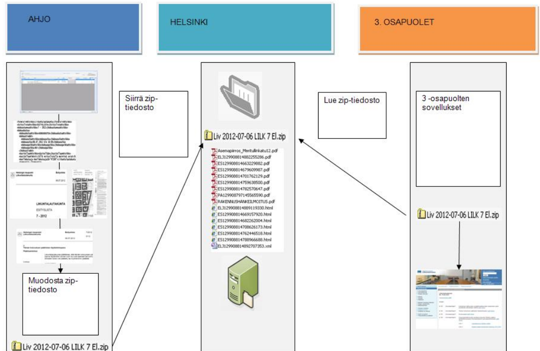
Kuva 6: OpenAhjo-ratkaisun tekninen kokonaiskuva
