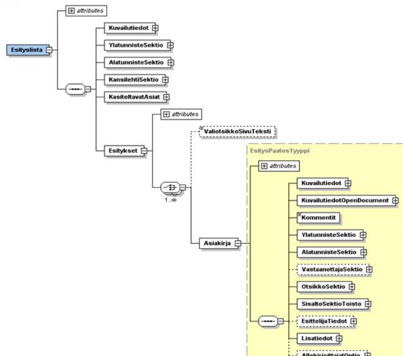
Kuva 11: OpenAhjon esityslistan rakennekuvaotos
