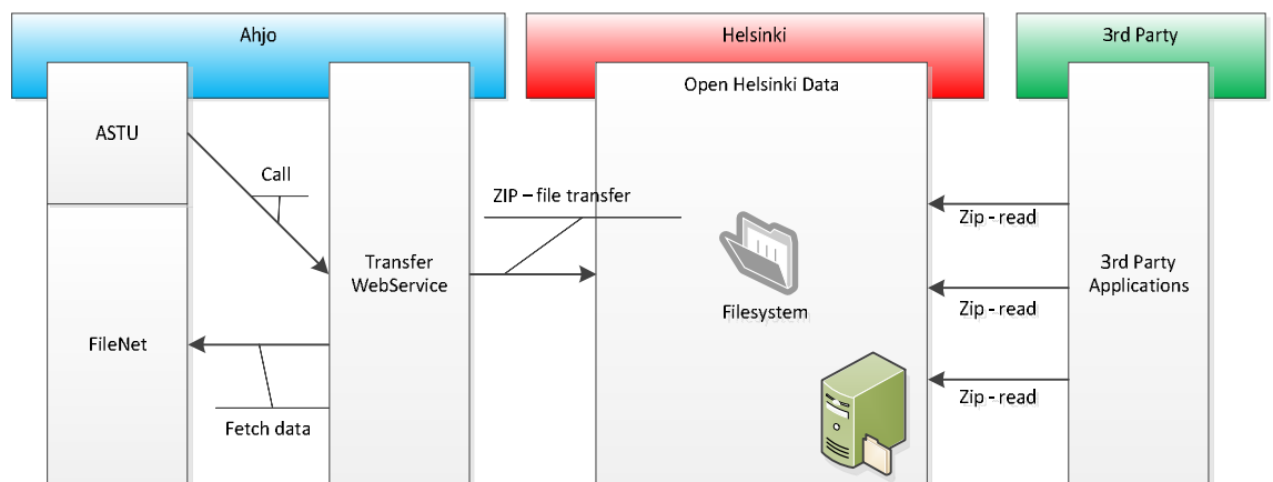
Kuva 14: Ensimmäisen vaiheen ”zip-tiedostoratkaisun” tekninen toimintakuva
