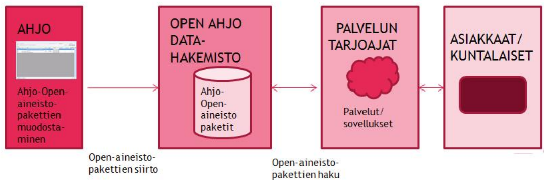
Kuva 1: OpenAhjo-ratkaisun karkea kokonaiskuva
