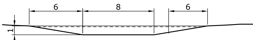
Havainnepoikkileikkaus avattavasta väylästä, B = 20 m
