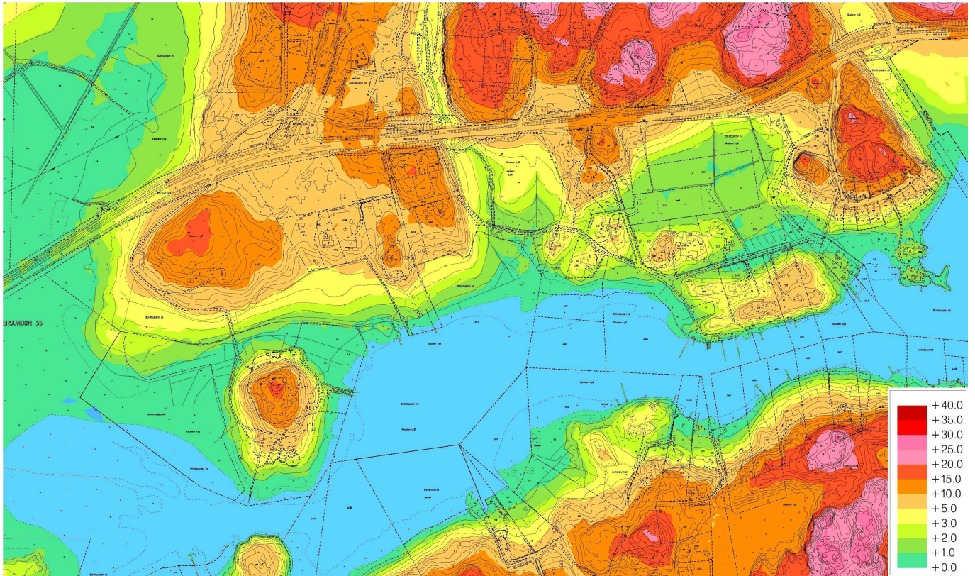
Kuva 4. Maanpinnan korkeusasema Korsnäsissa. Alava peltoalue erottuu kuvassa vihreällä. Kumpareet, joissa kallio on lähellä maanpintaa, näkyvät punaisella.
