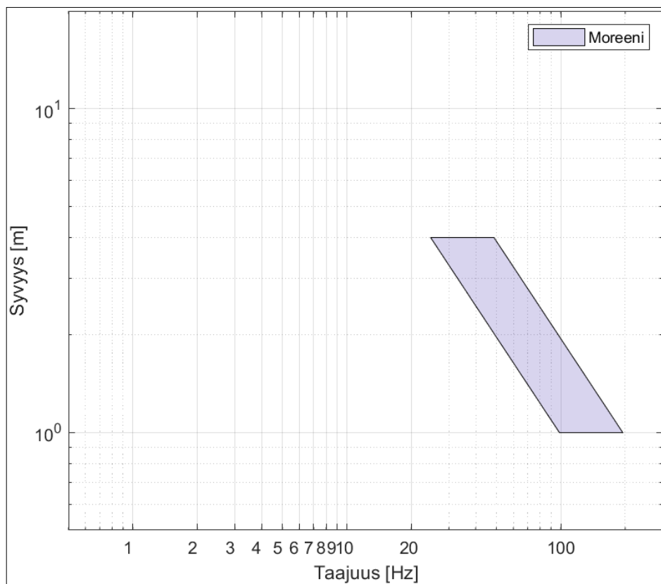
Kuva 2: Kohteessa esiintyvien maalajien resonanssi maakerroksen syvyyden suhteen mallin (1) mukaan.
