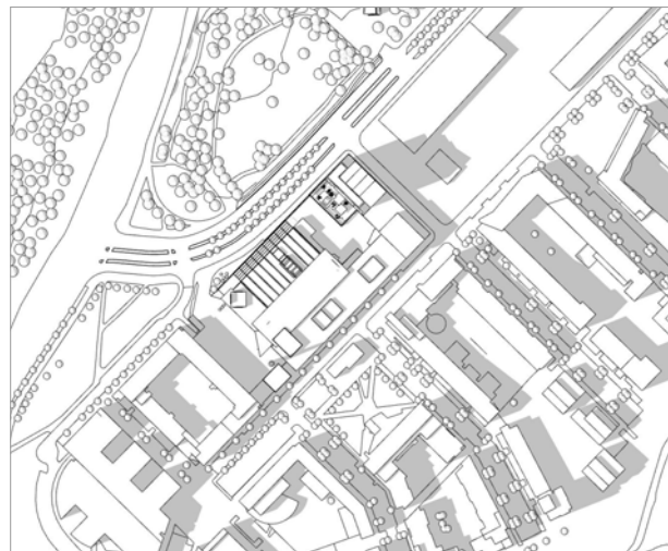
16:00 Kesäpäivänseisaus 1:2000
