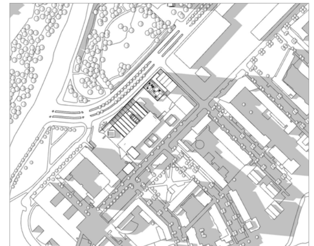
18:00 Kesäpäivänseisaus 1:2000
