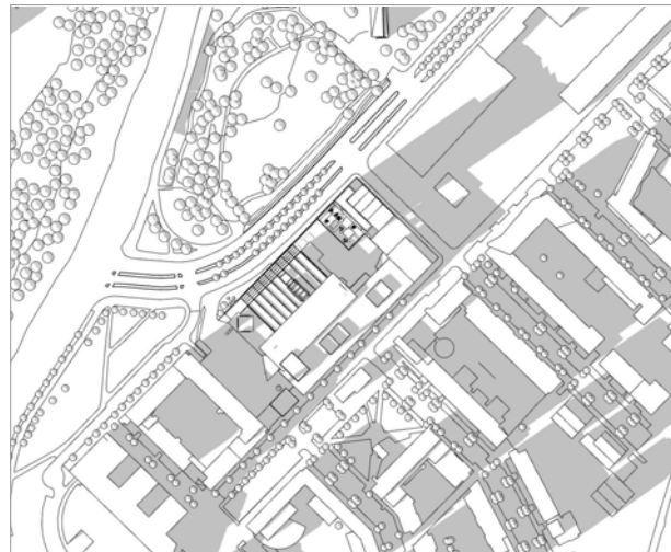
16:00 Kevätpäiväntasaus 1:2000
