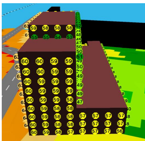
Kuva 4 Päiväajan julkisivumelutasot pohjoisesta, massavaihtoehto B.
