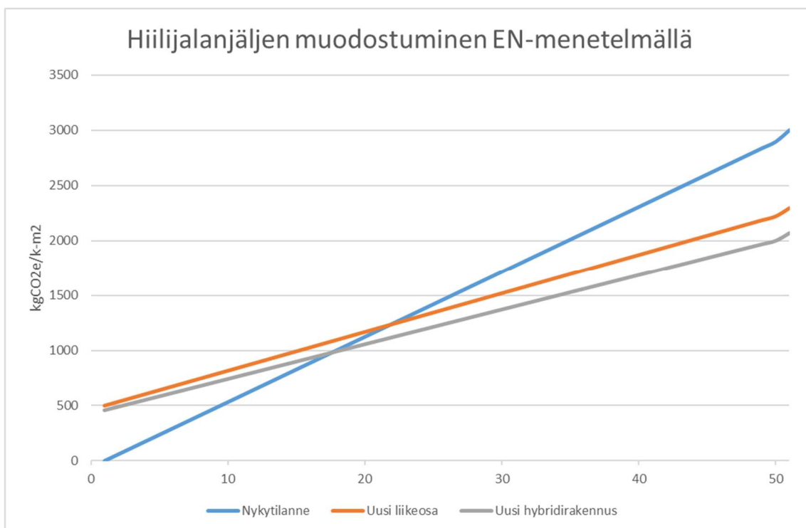
Kuva 6 Vaihtoehtojen hiilijalanjäljen ajallinen muodostuminen kerrosalaa kohden 50 vuodelle EN-standardin mukaisesti
