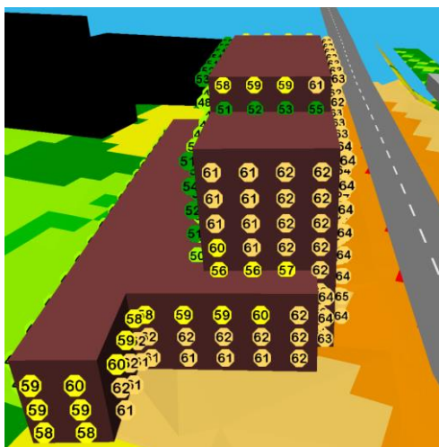
Kuva 10 Päiväajan julkisivumelutasot pohjoisesta, massavaihtoehto C.
