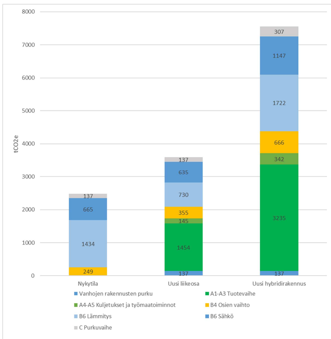
Kuva 3 Vaihtoehtojen kokonaishiilijalanjälki tonnia kgCO 2 e 50 vuoden aikana
