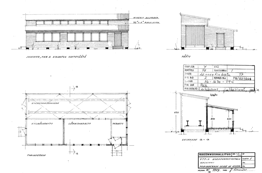
Pihalle rakennettava koekuormitusrakennus 1959. KA, RVV
