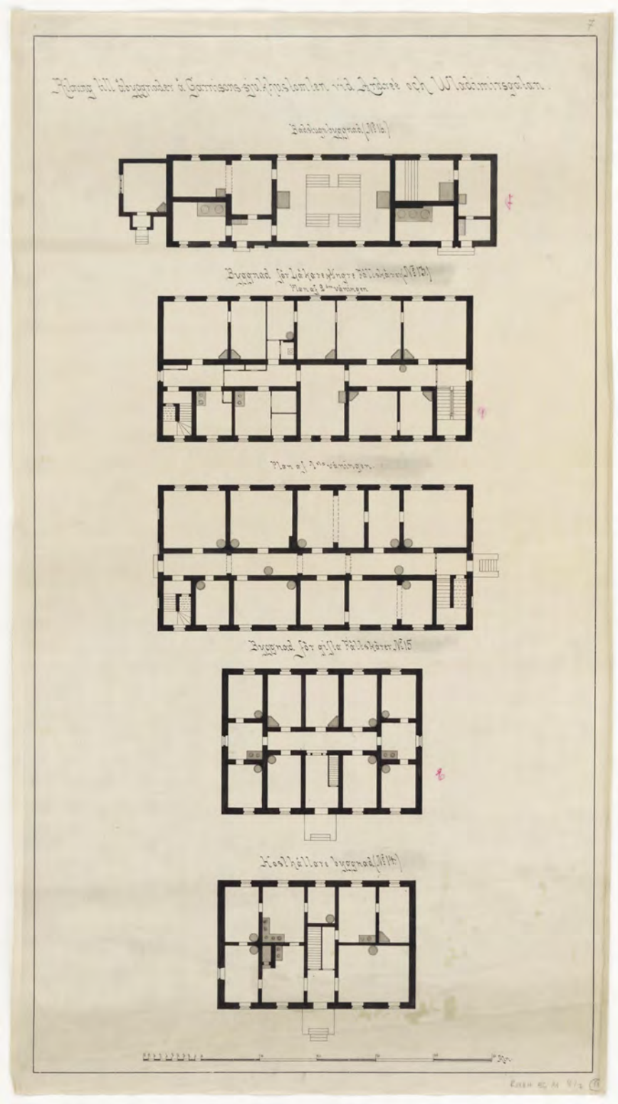
Sauna, vanha lasaretti, henkilökunnan asuinrakennus ja ruoanpitäjän rakennus, pohjapiirroksat 1880-l. KA
