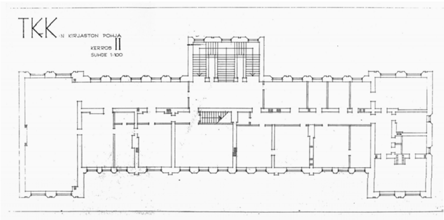
Sairaalan muutosluonnos – 2. kerroksen vanhojen käytävien jakaminen ja uuden käytävän rakentaminen. KA
