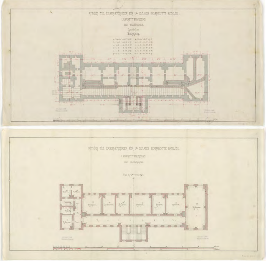
Varuskuntasairaalan kellarikerros lämmitys- ja ilmanvaihtolaitteineen ja 2. kerros. Päiväämättömät piirustukset 1880-luvulta. KA
