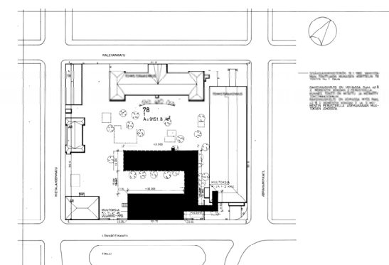
Maanalaisen laboratorion asemapiirros 1983. RVV, SKA
