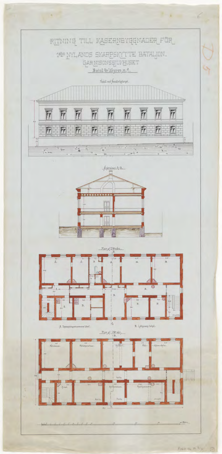
Lasaretin muutospiirustus n. 1884. KA
