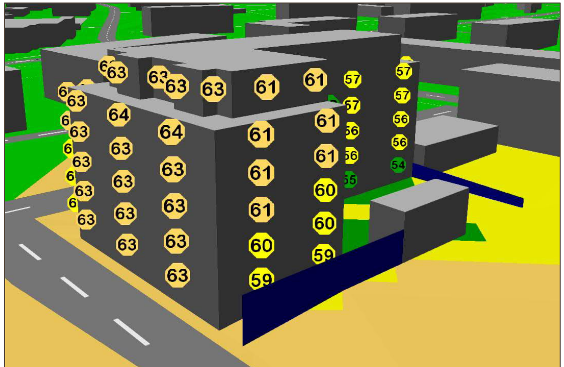
Kuva 2. 3D-näkymä kaakosta. Meluesteet esitetty kuvassa sinisellä.
