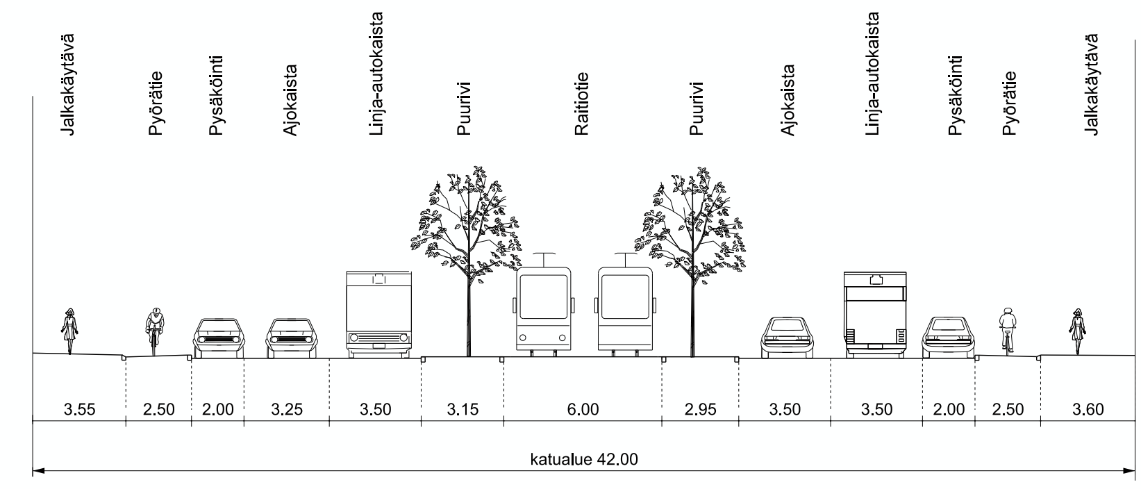
POIKKILEIKKAUS B - B 1:200
