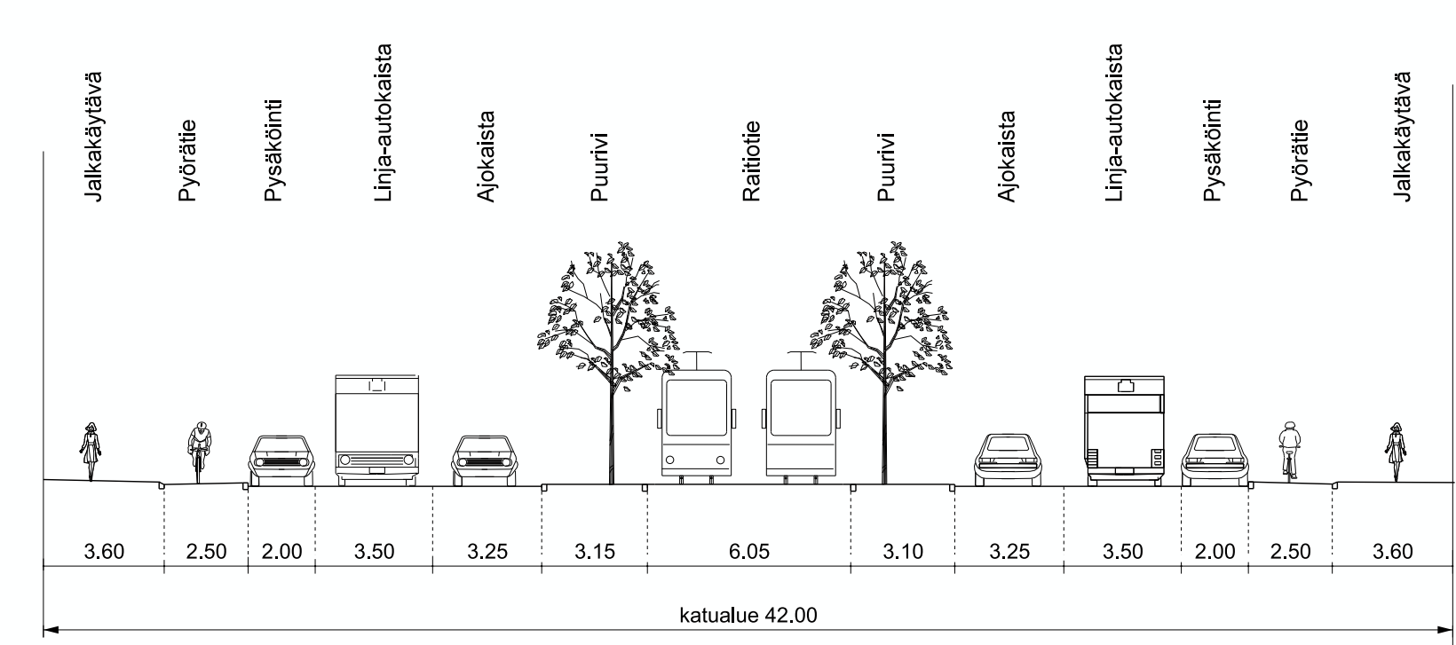
POIKKILEIKKAUS D - D 1:200
