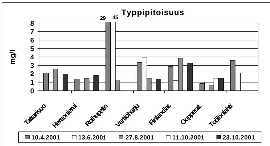
Kuva 6. Huleveden kokonaistyyppipitoisuus.
