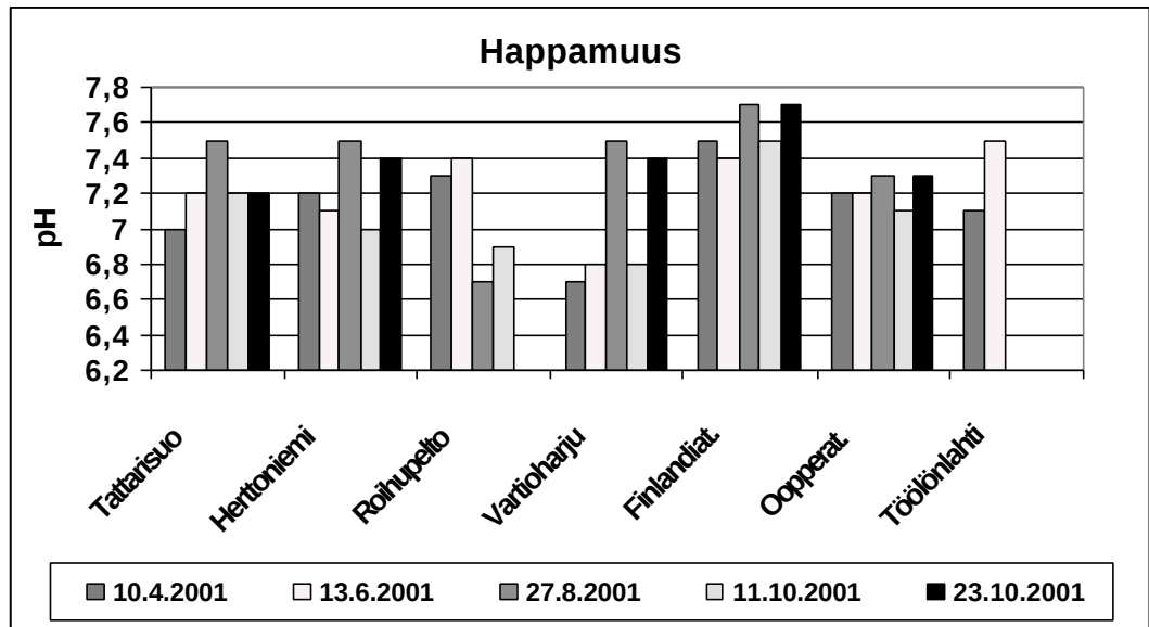
Kuva 2. Huleveden happamuus.
