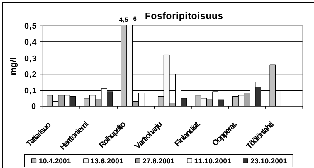
Kuva 5. Huleveden kokonaisfosforipitoisuus.
