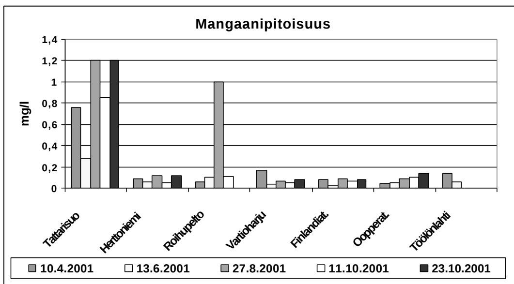
Kuva 11. Huleveden mangaanipitoisuus.
