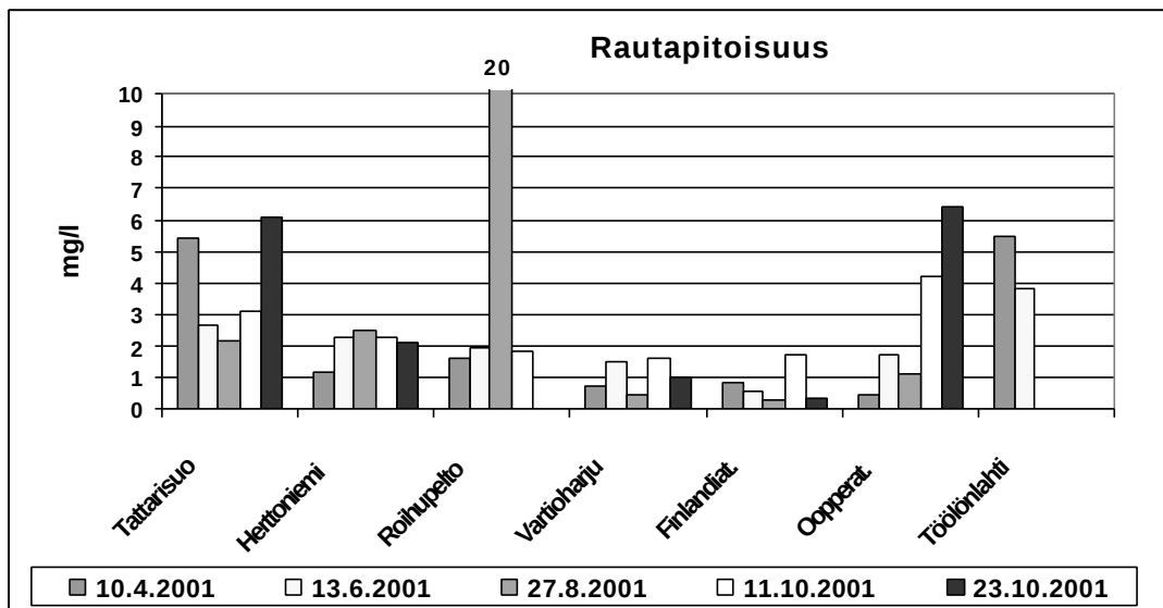
Kuva 10. Huleveden rautapitoisuus.
