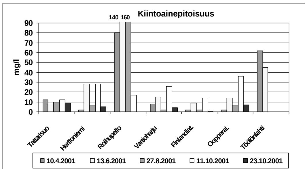
Kuva 3. Huleveden kiintoainepitoisuus.
