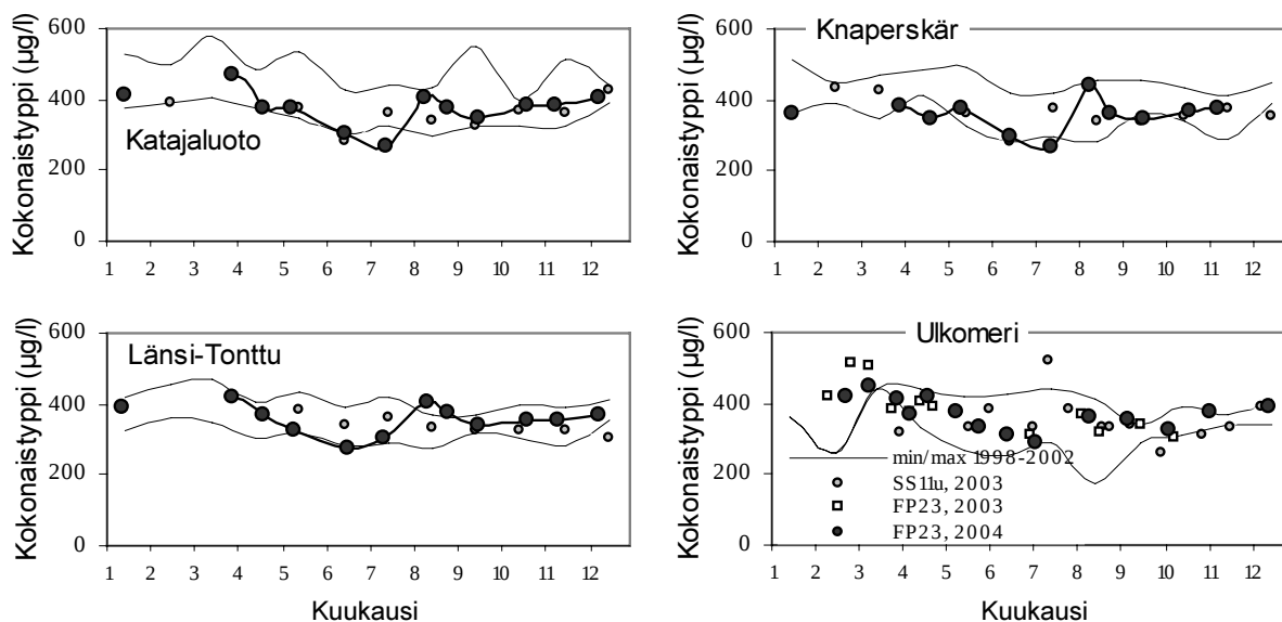
Kuva 5.25. Kokonaistypipitoisuus (vesipatsakeskiarvo) Katajaluodon, Knaperskärin ja Länsi-Tontun havaintopaikoilla vuosina 1995–2004. Ulkomereltä on Alg@line-projektin pintavesituloksia (minimi- ja maksimiarvot ovat vuosilta 1998–2002). —●— vuosi 2004, ○ vuosi 2003 ja — minimi- ja maksimiarvot vuosilta 1995–2002.
