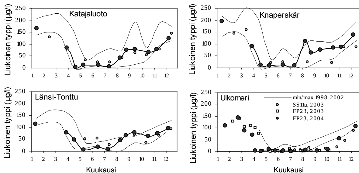
Kuva 5.21. Liukoisten typpiravinteiden (vesipatsakeskeskiarvo) pitoisuus Katajaluodon, Knaperskärin ja Länsi-Tontun havaintopaikoilla vuosina 1995–2004. Ulkomereltä on Alg@line-projektin pintavesituloksia (minimi- ja maksimi-arvot ovat vuosilta 1998–2002).
