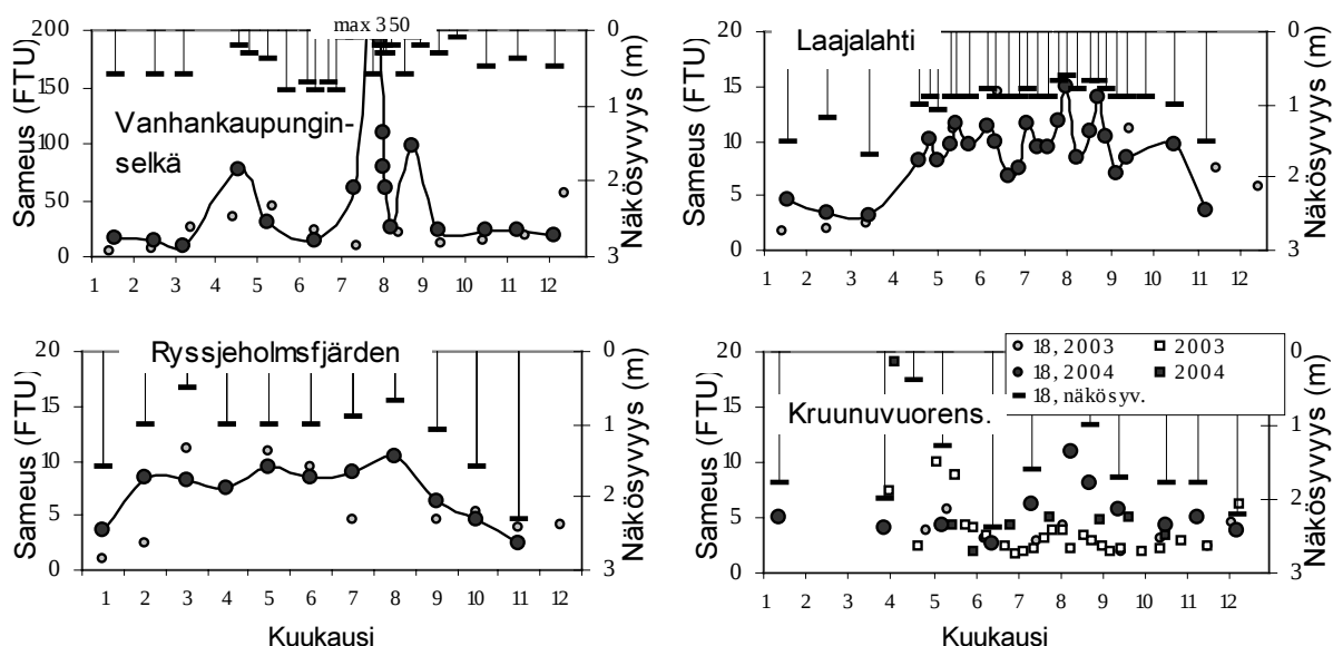
Kuva 5.3. Veden sameus (vesipatsakeskiarvo) ja näkösyyvyys Vanhankaupunginselän, Laajalahden ja Ryssjeholmsfjärdenin havaintopaikoilla vuosina 2003 ja 2004. Kruunuvuorenselältä on sekä Alg@line-projektin laivaseurantatuloksia että Vasikkasaaren (18) pintavesituloksia. Huomaa, että Vanhankaupunginselän kuvassa on muista poikkeava y-akselin skaalaus.
