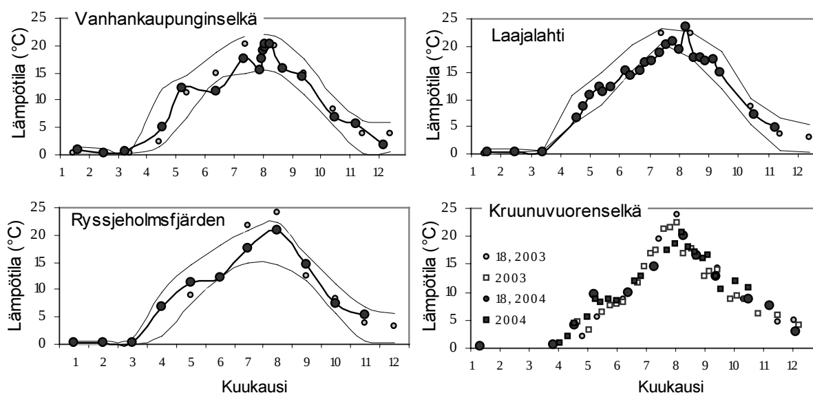
Kuva 5.1. Veden lämpötila (vesipatsaskeskiarvo) Vanhankaupunginselän, Laajalahden ja Ryssjeholmsfjärdenin havaintopaikoilla vuosina 1995–2004. Kruunuvuorenselältä on sekä Alg@line-projektin laivaseurantatuloksia että Vasikkasaaren (18) pintavesituloksia. —●— vuosi 2004, ○ vuosi 2003 ja ——— minimi- ja maksimiarvot vuosilta 1995–2002.
