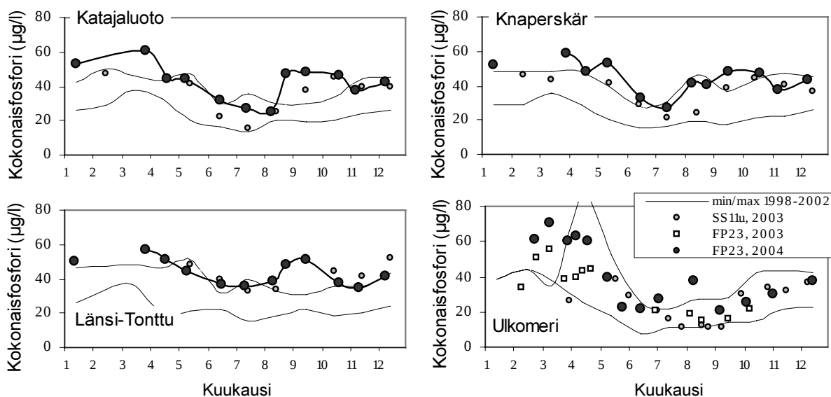
Kuva 5.23. Kokonaisfosforipitoisuus (vesipatsakeskiarvo) Katajaluodon, Knaperskärin ja Länsi-Tontun havaintopaikoilla vuosina 1995–2004. Ulkomereltä on Alg@line-projektin pintavesituloksia (minimi- ja maksimi-arvot ovat vuosilta 1998–2002). —●— vuosi 2004, ○ vuosi 2003 ja —□— minimi- ja maksimi-arvot vuosilta 1995–2002.
