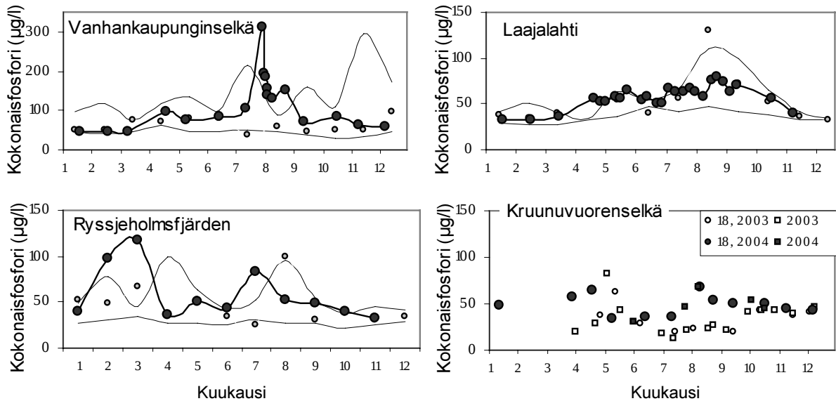
Kuva 5.7. Kokonaisfosforipitoisuus (vesipatsakeskiarvo) Vanhankaupunginselän, Laajalahden ja Ryssjeholmsfjärdenin havaintopaikoilla vuosina 1995–2004. Kruunuvuorenselältä on sekä Alg@line-projektin laivaseurantatuloksia että Vasikkasaaren (18) pintavesituloksia. Huomaa, että Vanhankaupunginselän kuvassa on muista poikkeava y-akselin skaalaus. —●— vuosi 2004, ○ vuosi 2003 ja — minimi- ja maksimiarvot vuosilta 1995–2002.
