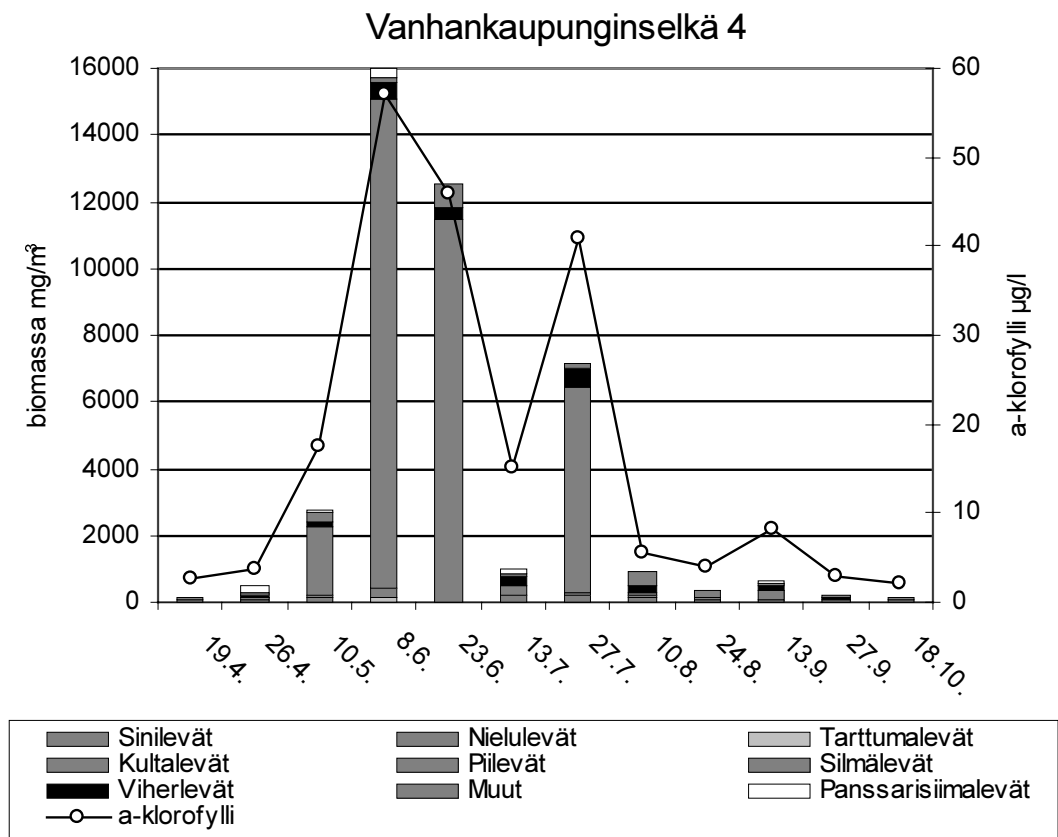
Kuva 6.1. Vanhankaupunginselän kasviplanktonin biomassat ( \text{mg}/\text{m}^3 ) ja a -klorofyllipitoisuudet ( \mu\text{g}/\text{l} ) kasvukaudella 2004, 0–2 metrin näytteet.
