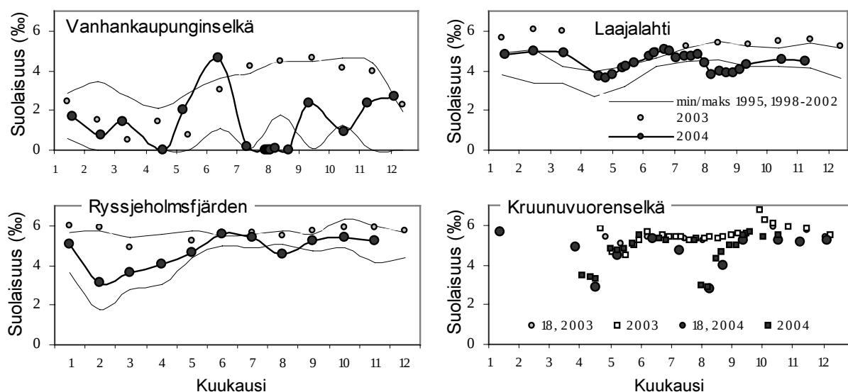
Kuva 5.2. Veden suolaisuus (vesipatsakeskiarvo) Vanhankaupunginselän, Laajalahden ja Ryssjeholmsfjärdenin havaintopaikoilla vuosina 1995–2004. Kruunuvuorenselältä on sekä Alg@line-projektin laivaseurantatuloksia että Vasikkasaaren (18) pintavesituloksia. —●— vuosi 2004, ○ vuosi 2003 ja — minimi- ja maksimiarvot vuosilta 1995–2002.
