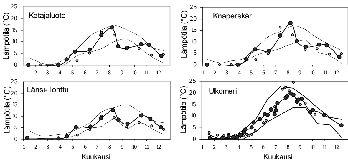
Kuva 5.11. Veden lämpötila (vesipatsakeskiarvo) Katajaluodon, Knaperskärin ja Länsi-Tontun havaintopaikoilla vuosina 1995–2004. Ulkomereltä on Alg@line-projektin pintavesituloksia (minimi- ja maksimi-arvot ovat vuosilta 1998–2002). —●— vuosi 2004, o vuosi 2003 ja — minimi- ja maksimi-arvot vuosilta 1995–2002.
