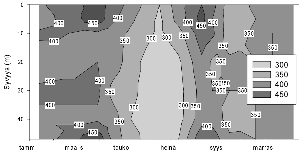
Kuva 5.26. Kokonaistypen pitoisuuden saman arvon käyrät Länsi-Tontun havaintopaikalla (nro 114) vuonna 2003.
