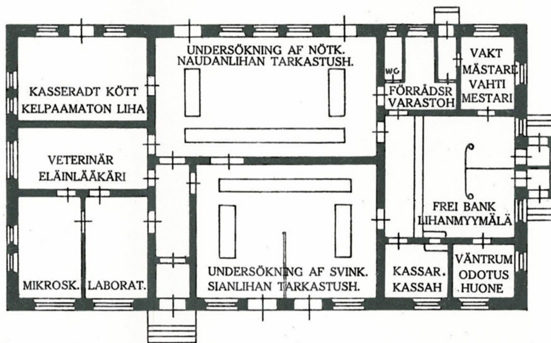
BETJENINGS BYGGNAD - PALVELUSVÄEN RAKENNUS
