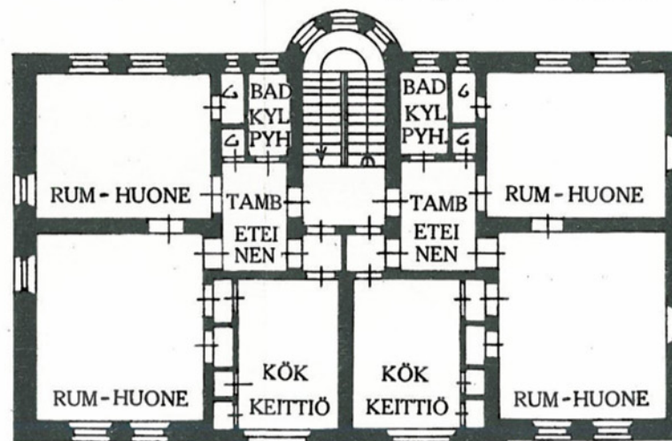
I, II OCH IIIJE VÄN. - I, II JA IIIAS KERROS
