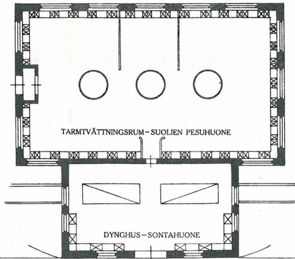
TARMTVÄTT- & DYNGHUS - SUOLIEN PESU- JA SONTAHUONE
