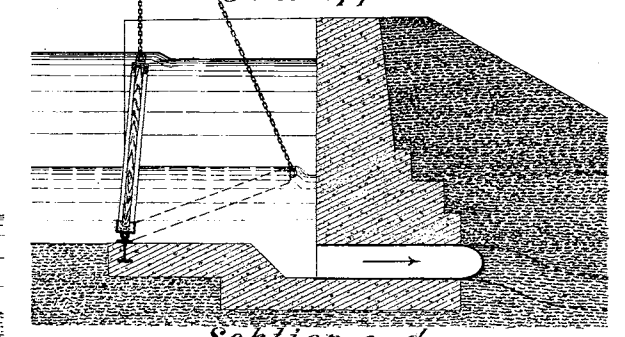
Sektion a-b. Ytaflopp till filterna.
