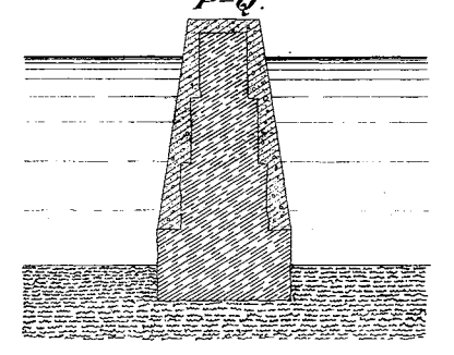
Profil af skärmdammen.
