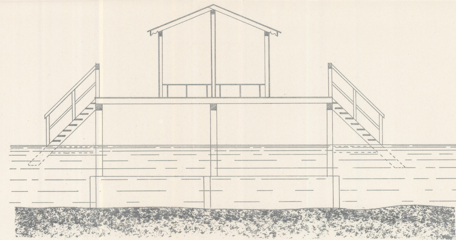
G. SKÄRNING. A-B.
