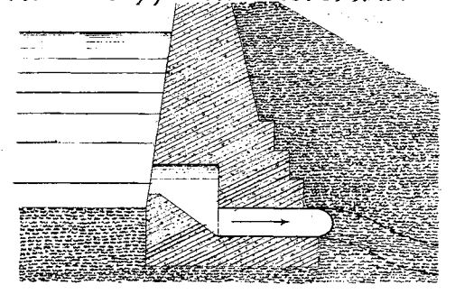
Sektion c-d. Bottenaflopp till filterna.
