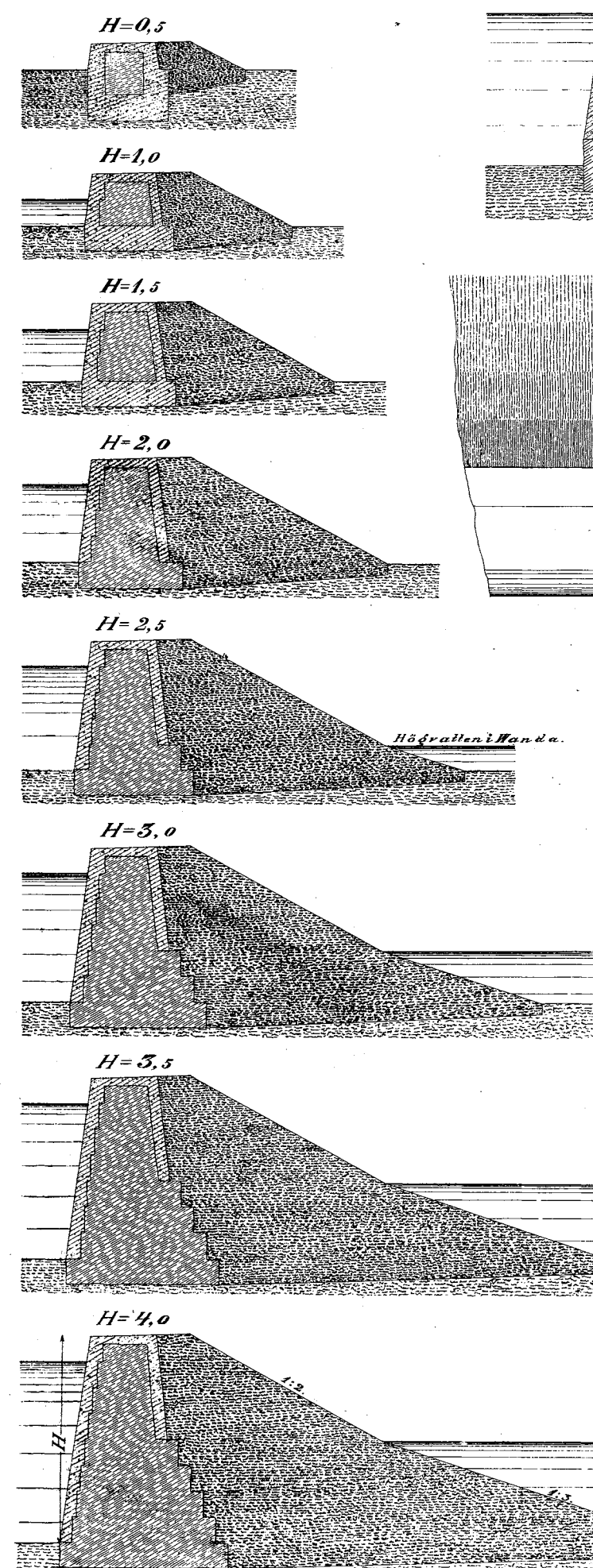
Dammprofiler.
