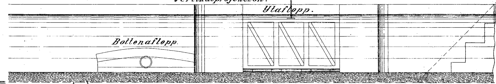
Sektion a-b. Ytaflopp till filterna.
