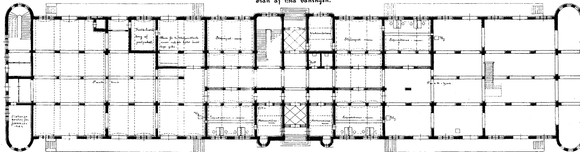
Plan af 1:ota våningen.
