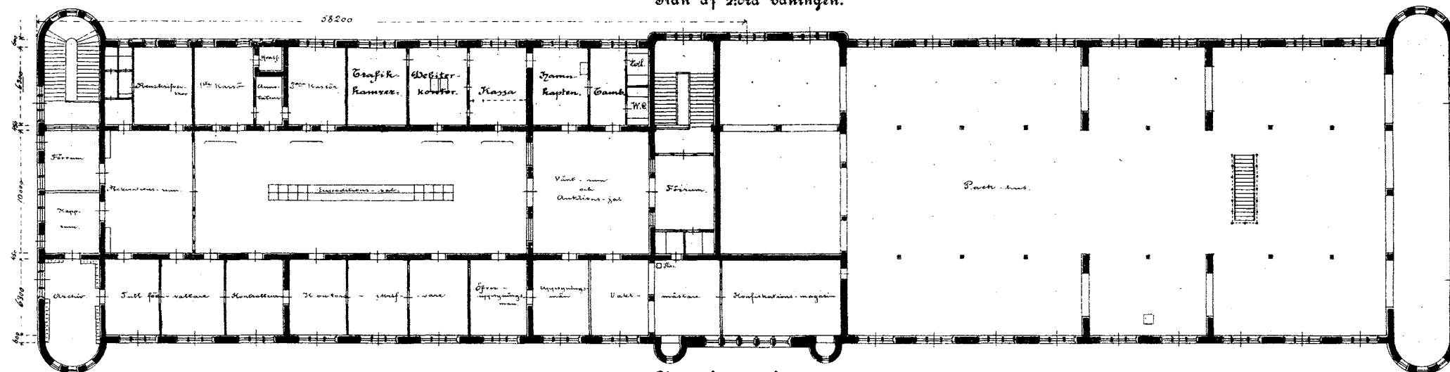
Plan af 1:ota våningen.
