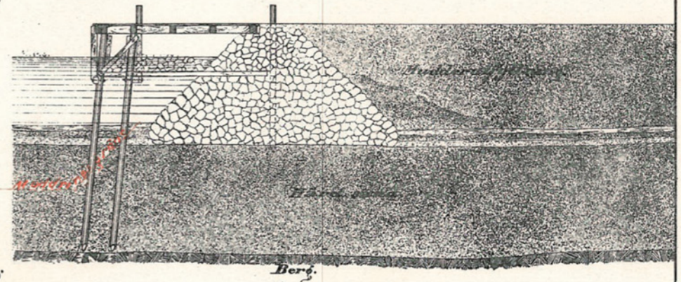
Tvärsektion af den föreslagna Gräsvikskajen vid a.
