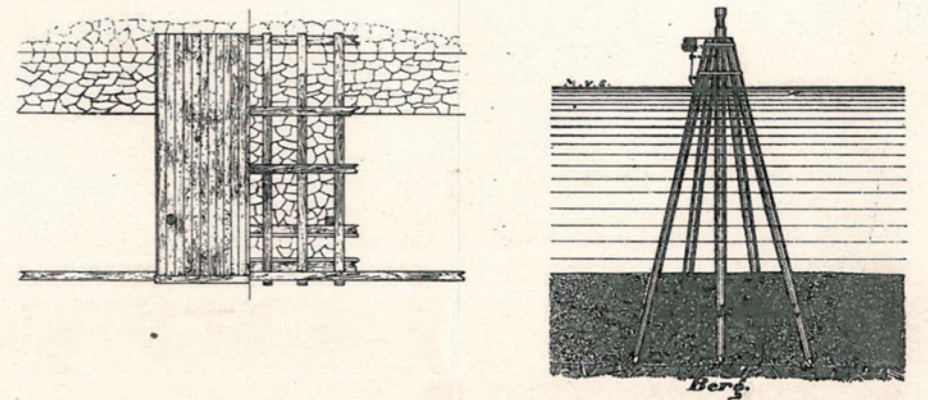
Plan jämte detaljer af en lastningsbrygga.
