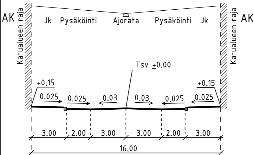
POIKKILEIKKAUS A-A, 1:200
