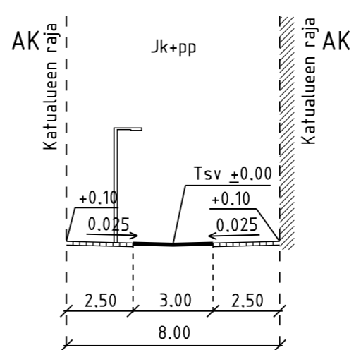
POIKKILEIKKAUS B-B, 1:200
