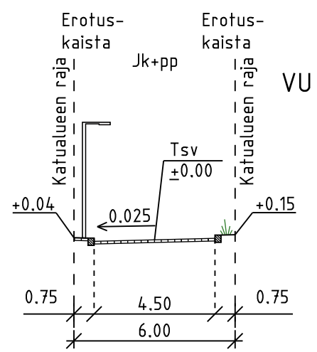
POIKKILEIKKAUS A-A, 1:200
