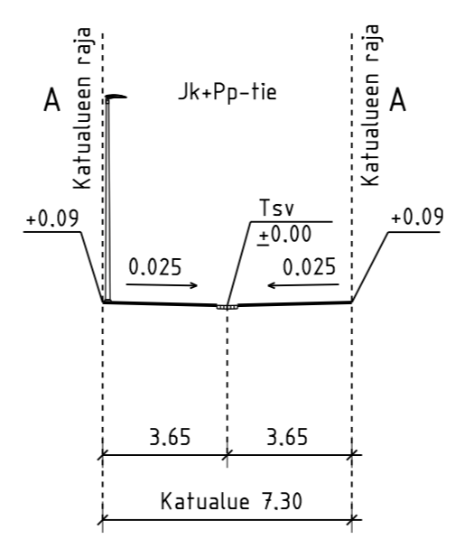
POIKKILEIKKAUS A - A 1:200
