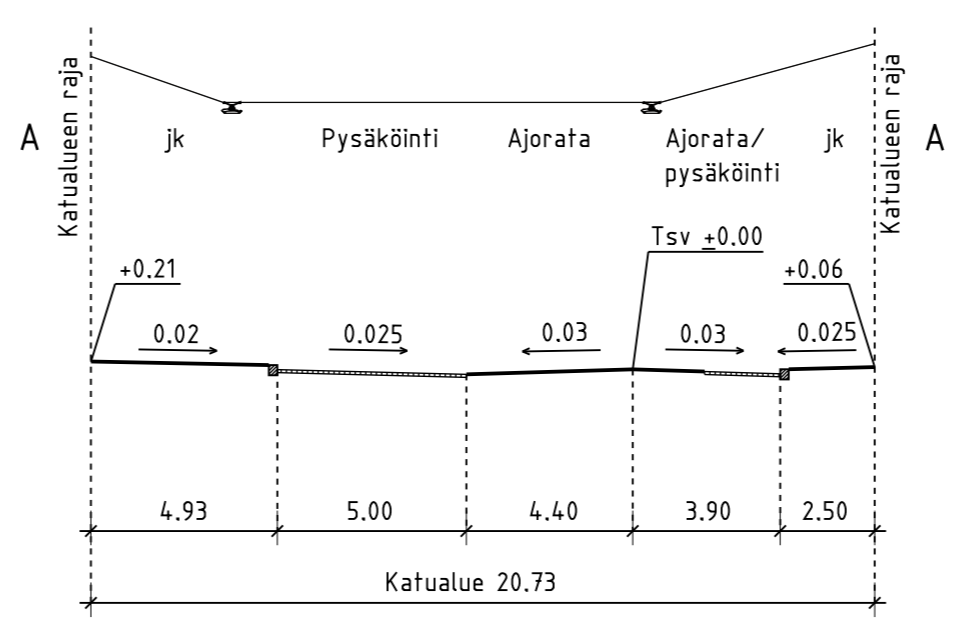
POIKKILEIKKAUS A - A 1:200
