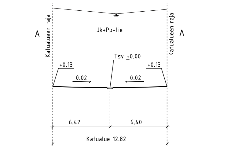
POIKKILEIKKAUS B - B 1:200
